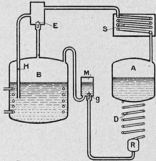
FIG. 3. — SCHEMA DU NOUVEL APPAREIL A GLACE A FONCTIONNEMENT INDEFINI
