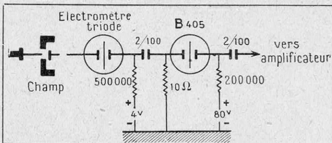
FIG. 7. — SCHÉMA DE L'AMPLIFICATEUR, RELIÉ, D'UNE PART, A LA LAME « A » DE L'APPAREIL REPRÉSENTÉ PAR LA FIGURE 6 ET, D'AUTRE PART, A UN OSCILLOGRAPHE, ET QUI PERMET D'OBTENIR LES COURBES DE LA FIGURE 8
