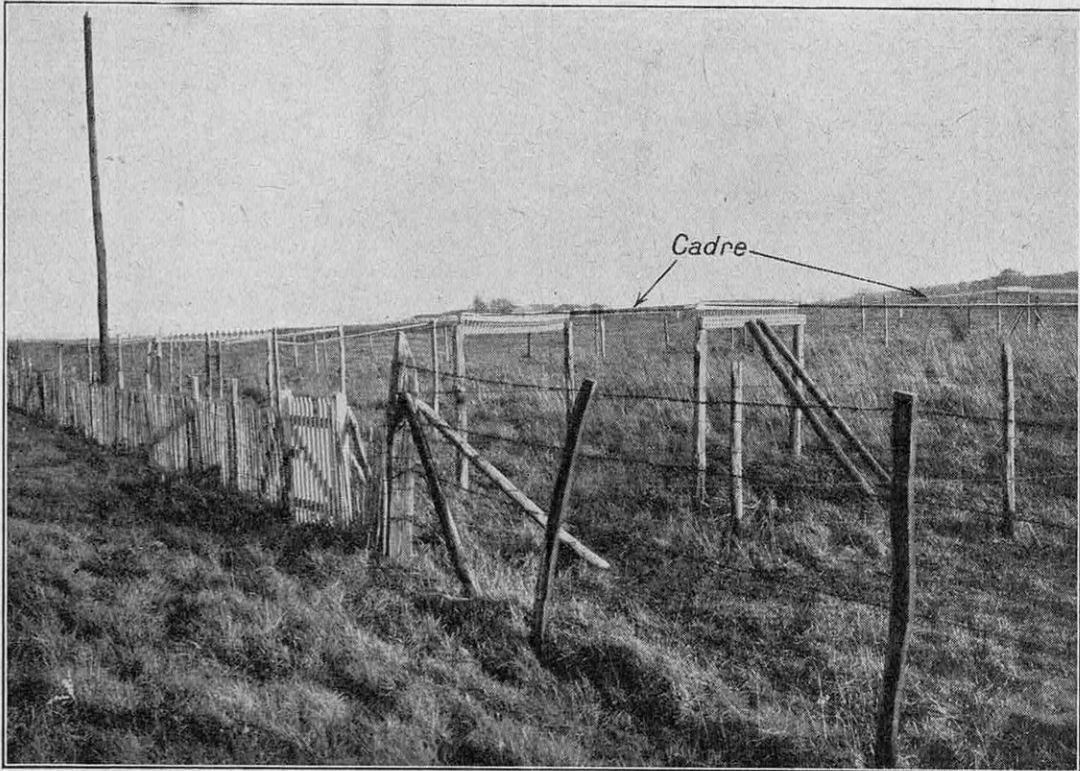
A L'OBSERVATOIRE DU VAL-JOYEUX, PRÈS DE PARIS, UN GRAND CADRE HORIZONTAL DE 80.000 MÈTRES CARRÉS PERMET DE MESURER ET D'ÉTUДИER LES VARIATIONS DE LA COMPOSANTE VERTICALE DU CHAMP MAGNÉTIQUE TERRESTRE
