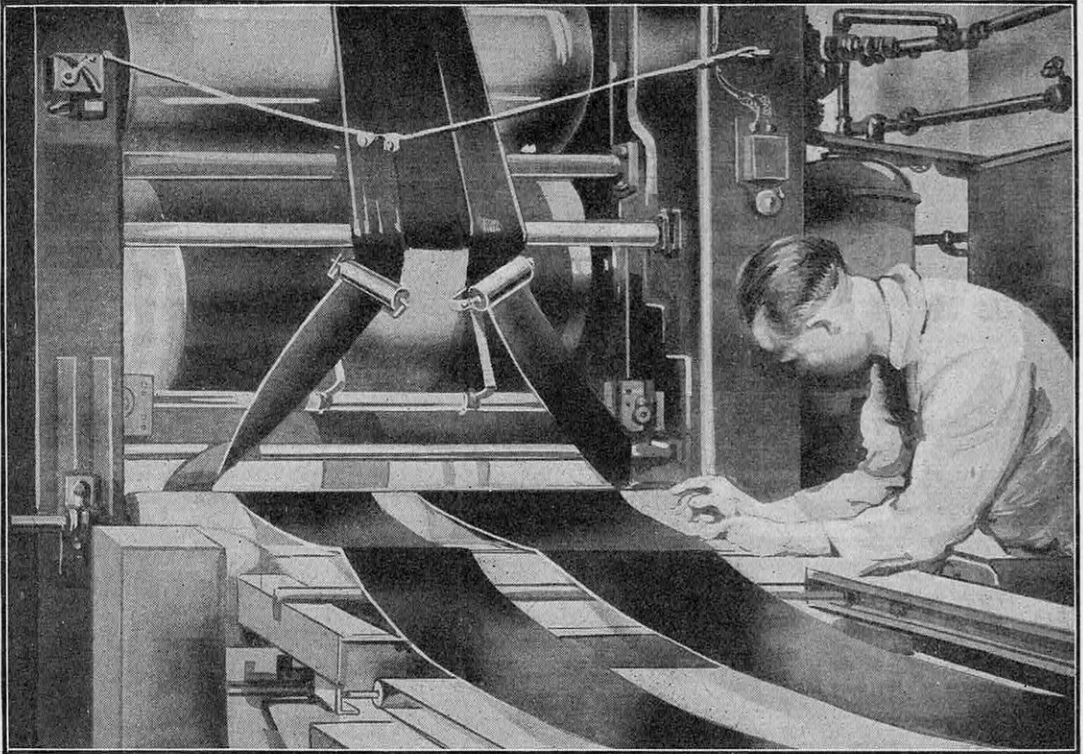
FIG. 1. — FABRICATION DES CHAPES, OU BANDES DE ROULEMENT, D'UN PNEUMATIQUE Calandre à quatre rouleaux pour la fabrication des chapes, ou bandes de roulement. Cette calandre agit comme un véritable laminoir, qui donne à la gomme la forme voulue.
