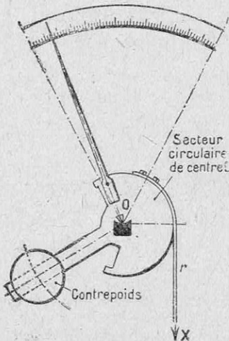
FIG. 12. — PESON, DIT « PESON A SINUS »
