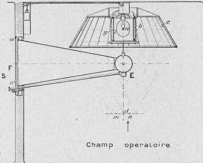
SCHÉMA DE FONCTIONNEMENT DU SCYALISCOPE DU PROFESSEUR CONSTANTINI
