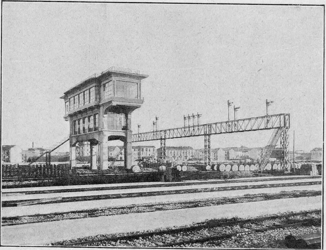
LA PASSERELLE DES SIGNAUX ET LE POSTE D'ENCLENCHEMENT QUI COMMANDE LES VOIES ABOUTISSANT AUX VINGT-QUATRE QUAIS DE LA GARE DE MILAN
