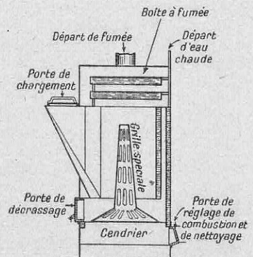
COUPE DE LA CHAUDIÈRE
