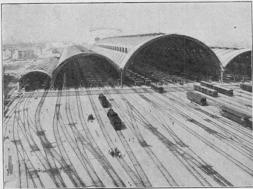
ENSEMBLE DES CINQ HALLS MÉTALLIQUES QUI ABRITENT LES VINGT-QUATRE QAIS DE LA GARE DE MILAN. LEUR LONGUEUR ATTEINT 341 MÈTRES
