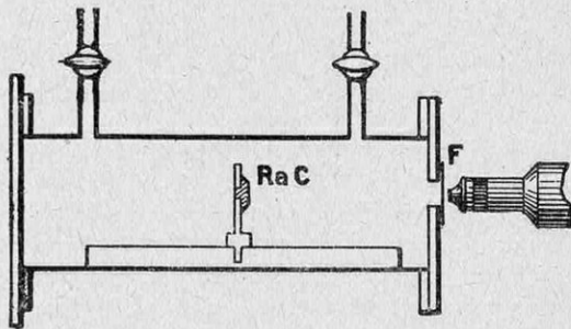
FIG. 5. — APPAREIL DE RUTHERFORD POUR LA DÉSINTÉGRATION DES ATOMES Ra C, radium C ; F, écran fluorescent.
