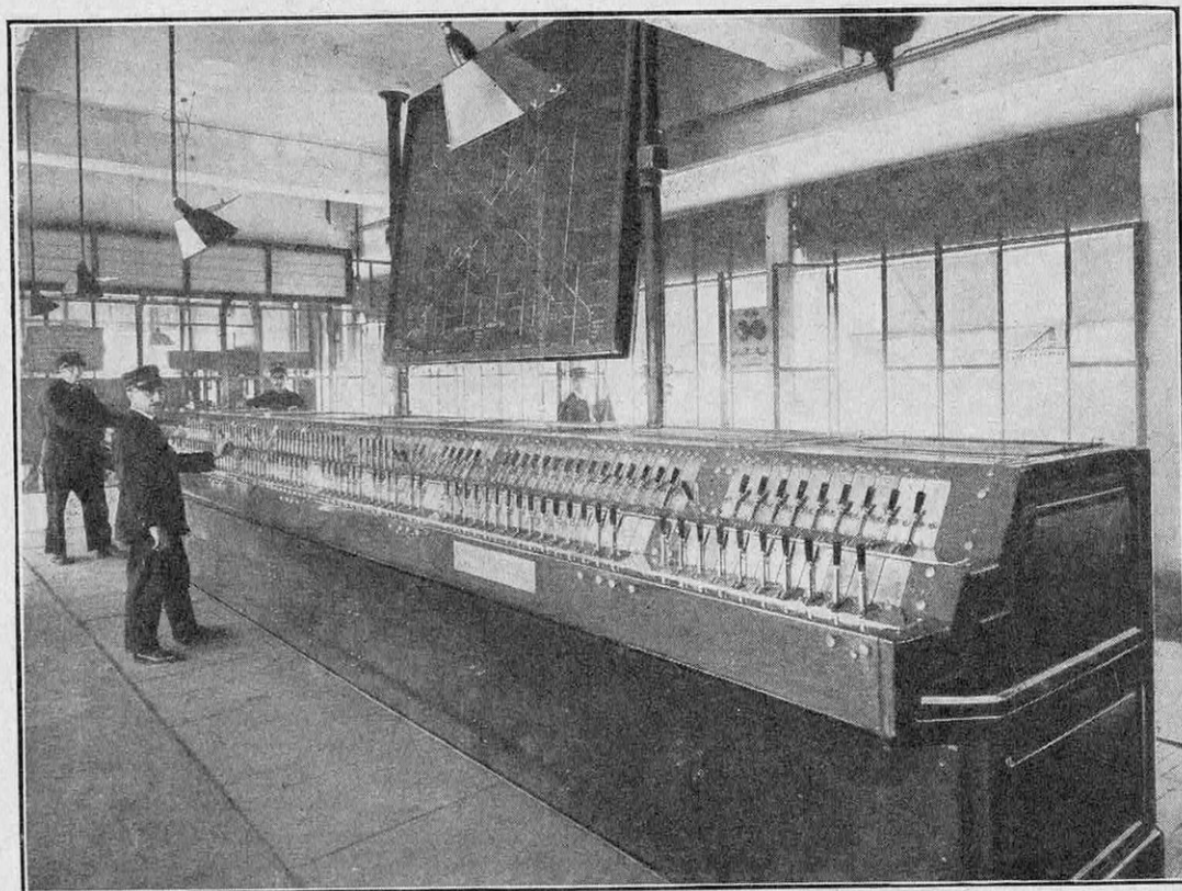
LA TABLE D'ENCLENCHEMENT DE LA CABINE CENTRALE DE LA GARE DE MILAN COMPORTE DEUX CENT-VINGT LEVIERS, COMMANDANT LES ARRIVÉES ET DÉPARTS DES TRAINS RAPIDES DANS TOUTES LES DIRECTIONS
