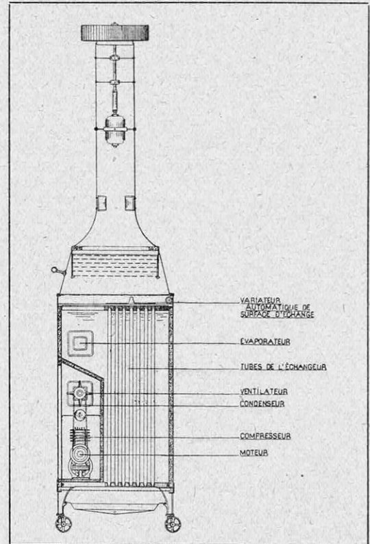
COUPE SCHÉMATIQUE DE L'APPAREIL PERMETTANT DE CONDITIONNER L'AIR DES APPARTEMENTS
