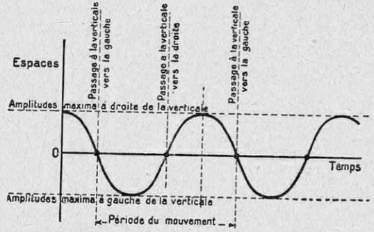
FIG. 17. — MOUVEMENT PENDULAIRE NON AMORTI, LA PALETTE DE LA FIGURE 16 ÉTANT COMPLÈTEMENT HORS DE L'HUILE
