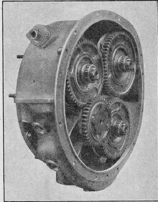
LES ENGRENAGES D'UN COMPRESSEUR A TROIS VITESSES PERMETTANT DE RÉTABLIR, A DIVERSES ALTITUDES, LA « PUISSANCE AU SOL » DU MOTEUR
