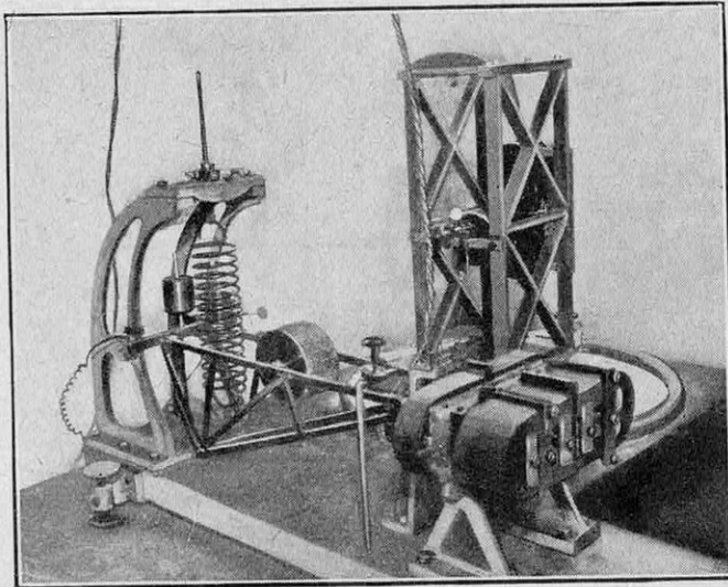
SÉISMOGRAPHE GALITZINE, EN SERVICE A L'OBSERVATOIRE DU PARC-SAINT-MAUR, PRÈS DE PARIS
