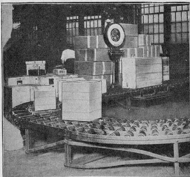
FIG. 30. — EXEMPLE DE BASCULE AUTOMATIQUE ADAPTÉE SUR UN TRANSPORTEUR A ROULEAUX
