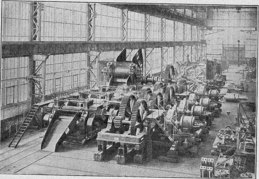
FIG. 3. — MOULIN PERMETTANT DE BROYER 1.200 TONNES DE CANNES A SUCRE PAR JOUR ET ACTIONNÉ PAR LES MOTEURS ÉLECTRIQUES VISIBLES A DROITE DE LA PHOTOGRAPHIE
