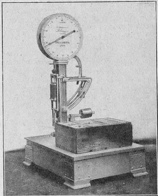
FIG. 14. — BASCULE « DUJOUR » DE 100 KILOGRAMMES GRADUÉE PAR 100 GRAMMES
