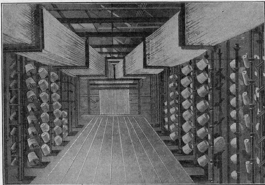
FIG. 2. — CONFECTION DU CABLÉ, QUI SERA ENSUITE CHARGÉ DE GOMME
