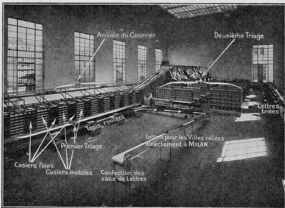
VUE D'ENSEMBLE DE LA SALLE DE TRIAGE DU BUREAU DE POSTE DE LA GARE DE MILAN
