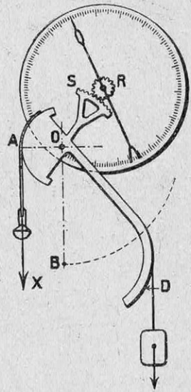
Cadran à divisions équidistantes
