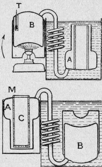
FIG. 1 ET 2. — SCHEMA D'UN APPAREIL A GLACE « CARRÉ » B , chaudière ; A , réservoir ; C , récipient à refroidir ; T , thermomètre.
