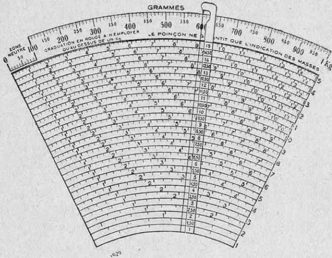
FIG. 27. — REPRODUCTION D'UN CADRAN DE BALANCE AUTOMATIQUE AVEC BARÈME DES PRIX
