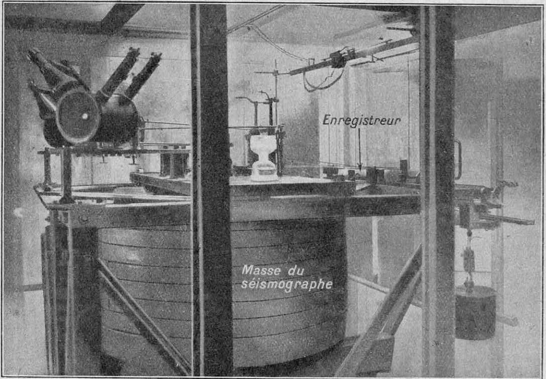
SÉISMOGRAPHE WIECHERT EN SERVICE A L'OBSERVATOIRE DU PARC-SAINT-MAUR, PRÈS DE PARIS La masse du séismographe, formée par un empilement de rondelles, est de 1 tonne. Dans le haut, à gauche, apparaissent les amortisseurs à air ; à droite, l'enregistreur.
