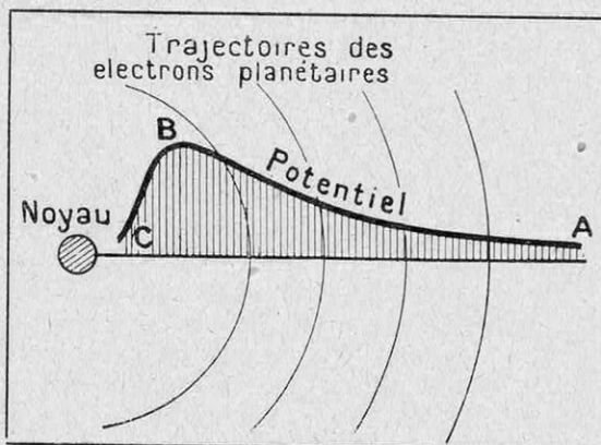
FIG. 2. — COURBE DES VARIATIONS DU POTENTIEL A L'INTÉRIEUR DE L'ATOME, D'APRÈS MAURICE DE BROGLIE
