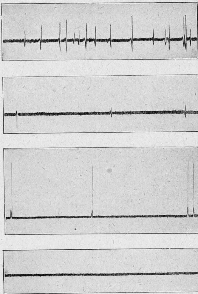
FIG. 8. — LES DEUX COURBES DU HAUT REPRÉSENTENT LA BANDE OBTENUE DANS LA DÉSINTÉGRATION DE L'ALUMINIUM, APRÈS 11 CENTIMÈTRES ET 24 CENTIMÈTRES D'ABSORPTION PAR L'AIR DES RAYONS « H ». CELLES DU BAS CORRESPONDENT À L'ENREGISTREMENT DES RAYONS « ALPHA » SUR LE MÊME PARCOURS ET LA BANDE DUE AU SOUFFLE SEUL DE L'APPAREIL AMPLIFICATEUR (FIG. 7)
