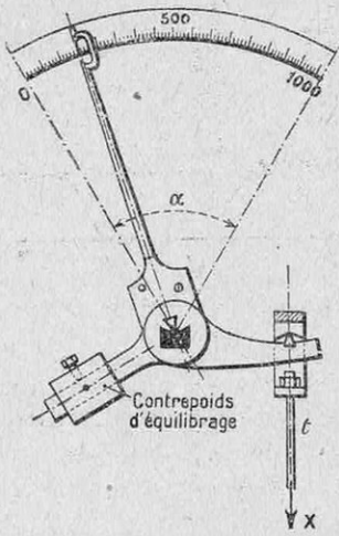
FIG. 11. — PESON, DIT « PESON A TANGENTE »
