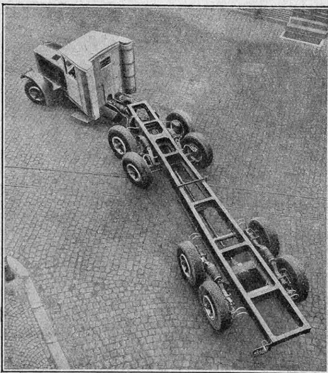
VUE D'ENSEMBLE DU CHASSIS DU CAMION KRUPP A DIX ROUES, MONTRANT COMMENT S'ARTICULE L'ARBRE DE TRANSMISSION ET COMMENT S'ORIENTENT LES ROUES AVANT DE LA REMORQUE PENDANT LES VIRAGES
