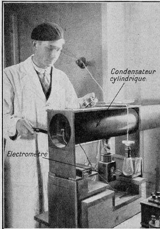
MESURE DE LA CONDUCTIBILITÉ ÉLECTRIQUE DE L'AIR ATMOSPHÉRIQUE A L'OBSERVATOIRE DU VAL-JOYEUX, PRÈS DE PARIS
