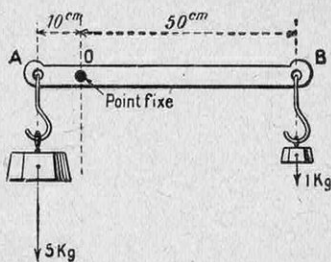
FIG. 4. - LEVIER DU PREMIER GENRE
