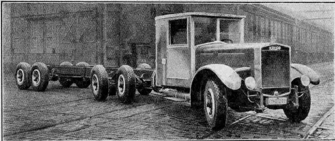
LE CAMION KRUPP A DIX ROUES EST CAPABLE, MALGRÉ SES 14 MÈTRES DE LONG, D'EFFEC-TUER SANS DIFFICULTÉ DES VIRAGES SERRÉS, GRACE A SON ARTICULATION ET A SON NOU-VEAU DISPOSITIF DE DIRECTION
