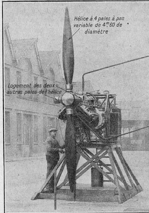
GRUPE MOTEUR DE L'AVION STRATOSPHERIQUE FRANÇAIS FARMAN-WASEIGE
