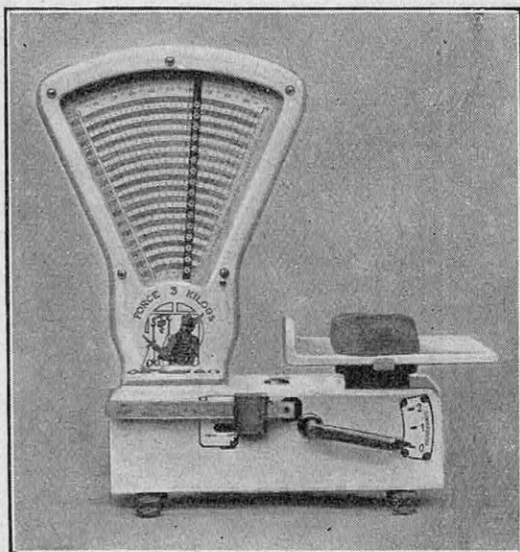
FIG. 3. — BALANCE AUTOMATIQUE A UN SEUL PLATEAU
