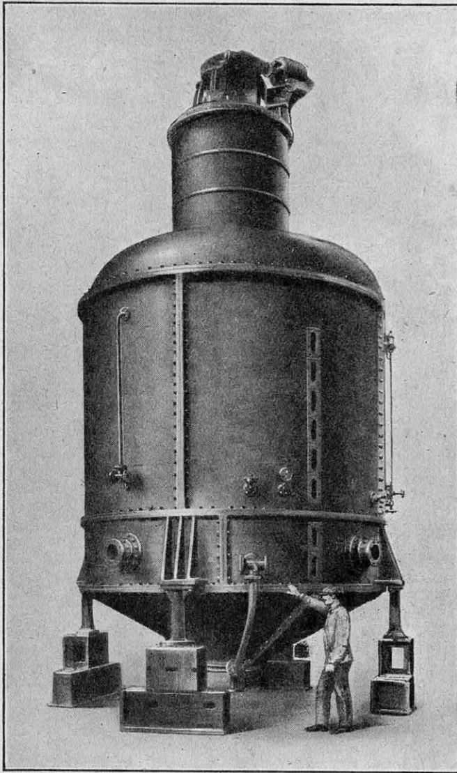
FIG. 7. — CHAUDIÈRE POUR CUIRE LE JUS SUCRÉ, CHAUFFÉE PAR UN FAISCEAU TUBULAIRE PARCOURU PAR DE LA VAPEUR A BASSE PRESSION
