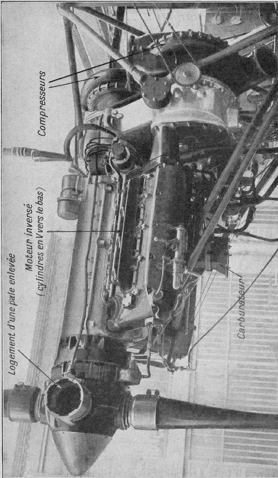
LE MOTEUR DE 350 CH DESTINÉ A L'AVION STRATOSPHERIQUE WASEIGE-FARMAN. C'EST UN MOTEUR A HUIT CYLINDRES EN V RENVERSÉS QUI REÇOIT L'AIR SOUS PRESSION DE TROIS COMPRESSEURS MONTÉS EN SÉRIE. L'HÉLICE, DE GRAND DIAMÈTRE (4 M 60), EST A PAS RÉGLABLE ET COMPORTE QUATRE PALES. DEUX DE CES PALES SONT ENLEVÉES SUR CETTE PHOTOGRAPHIE.
