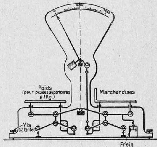
FIG. 26. — BALANCE SEMI-AUTOMATIQUE, MÉCANISME TYPE BÉRANGER
