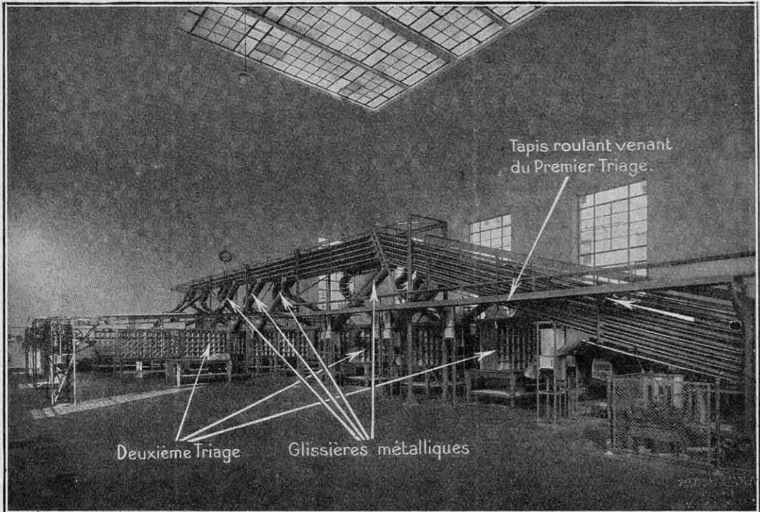
LE COURRIER, APRÈS UN PREMIER TRIAGE, EST AMENÉ AUTOMATIQUÉMENT VERS LE DEUXIÈME ET DERNIER TRIAGE PAR DES TAPIS ROULANTS ET DES GLISSIÈRES MÉTALLIQUES
