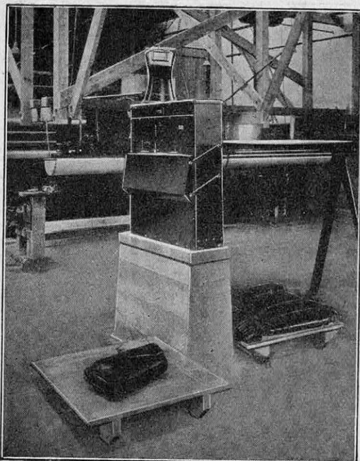
FIG. 32. — CONTRÔLE DE L'ÉPAISSEUR DE TISSUS CAOUTCHOUTÉS, AVEC ENREGISTREMENT GRAPHIQUE DU POIDS TROUVÉ
