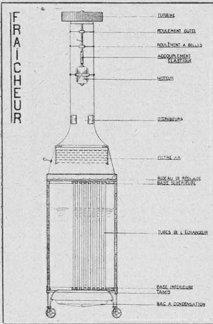
MODÈLE A GLACE
