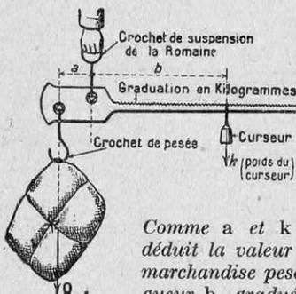
FIG. 7. — BALANCE ROMAINE
