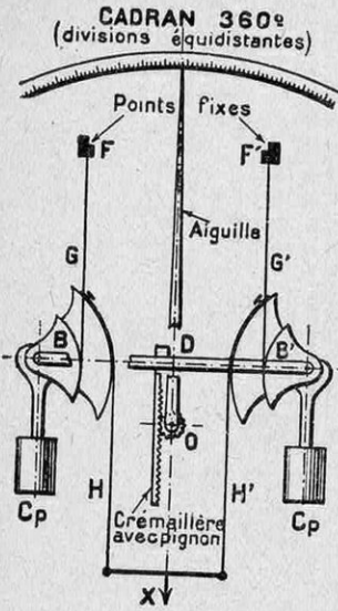
FIG. 15. — APPAREIL AUTOMATIQUE A DEUX PESONS A DOUBLE CAME CHACUN
