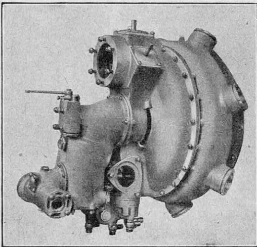
VUE EXTERIEURE D'UN COMPRESSEUR DÉBRAYABLE DESTINÉ A UN MOTEUR ANGLAIS DE 480 CH EN ÉTOILE
