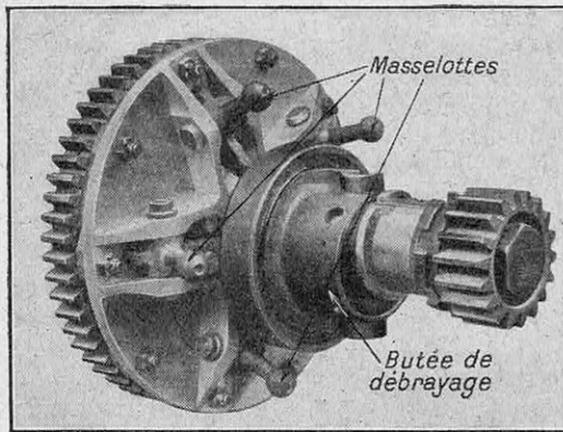
EMBRAYAGE CENTRIFUGE DES COMPRESSEURS FARMAN, AVEC SA BUTÉE DE DÉBRAYAGE
