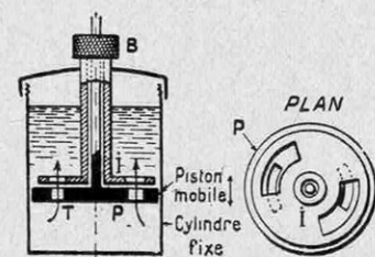
FIG. 23. — SCHEMA D'UN AMORTISSEUR A AIR On règle le frein plus ou moins « dur » en fermant plus ou moins le robinet R.
