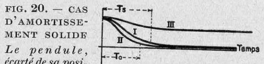
FIG. 20. — CAS D'AMORTISSEMENT SOLIDE Le pendule, écarté de sa position d'équilibre, ne peut y revenir qu'au bout d'un temps infini (courbe I). Parmi ces courbes, la courbe II correspond à l'amortissement « critique » ; le pendule revient très rapidement vers sa position d'équilibre au bout d'un temps très court ( T_c ), mais sans atteindre cette position. En III, le pendule s'arrête au bout d'un certain temps ( T_s ) avant d'avoir atteint sa position d'équilibre.
