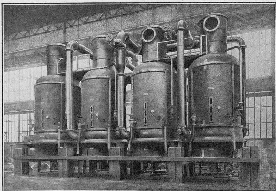
FIG. 6. — AUTRE OUTILLAGE A QUATRE « CAISSES » POUR L'ÉVAPORATION DES JUS SUCRÉS
