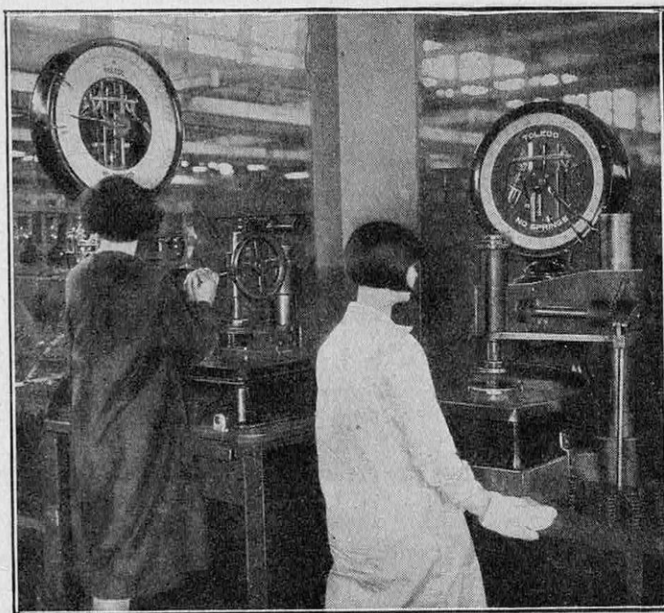
FIG. 31. — TARAGE DES RESSORTS AU MOYEN DE BALANÇES AUTOMATIQUES
