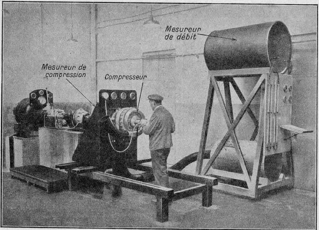
SALLE D'ESSAIS DES COMPRESSEURS AUX USINES FARMAN
