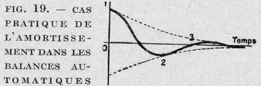
FIG. 19. — CAS PRATIQUE DE L'AMORTISSEMENT DANS LES BALANCES AUTOMATIQUES
