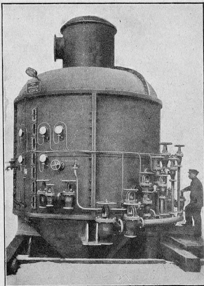
FIG. 8. — AUTRE TYPE DE CHAUDIÈRE POUR LA CUISSON DU JUS SUCRÉ, CHAUFFÉE PAR DES SERPENTINS CIRCULAIRES POUR VAPEUR A HAUTE PRESSION
