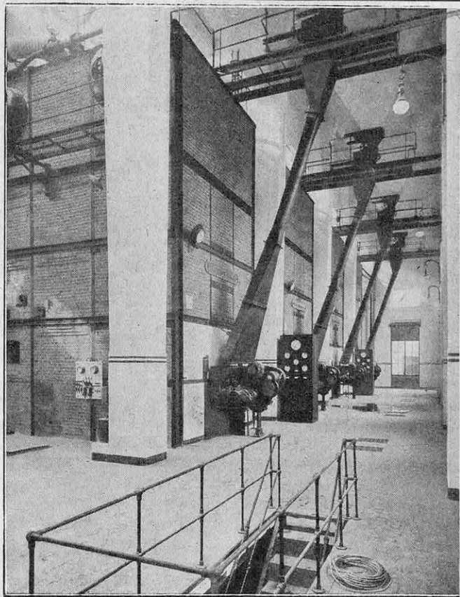
LA CENTRALE THERMIQUE DE LA GARE DE MILAN En haut, trémies de chargement du charbon ; en bas, les quatre chaudières à foyer automatique de la centrale thermique.
