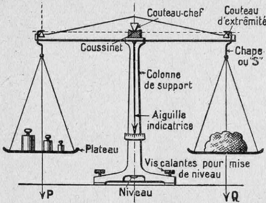
FIG. 6. — BALANCE-FLÉAU A BRAS ÉGAUX Le fléau oscille, puis se met en équilibre, de telle manière que l'aiguille soit bien verticale. A ce moment, le poids de la marchandise Q est égal aux poids P placés dans le plateau opposé. L'axe d'oscillation du fléau est constitué par la fine arête d'un « couteau », en acier trempé ou en agate (variété de silice très dure), reposant sur un « coussinet » également très dur.
