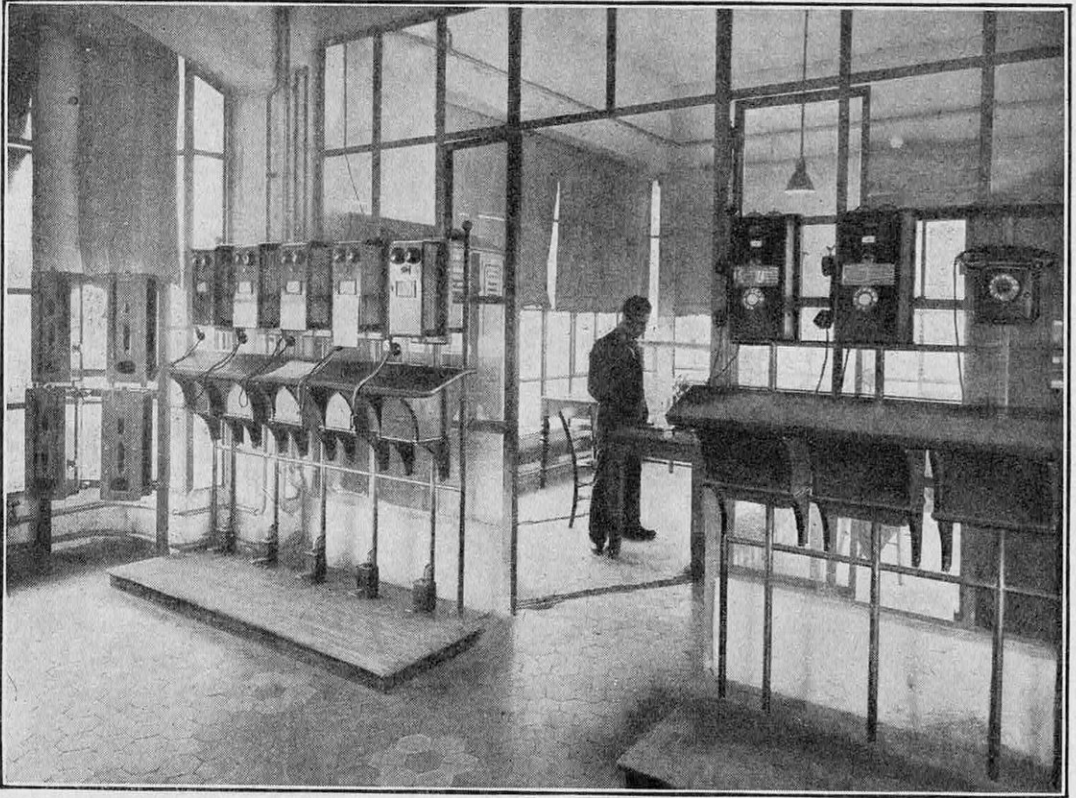
LES SERVICES TÉLÉPHONIQUES QUI RELIENT LA CABINE CENTRALE DES SIGNAUX DE LA GARE DE MILAN AUX HUIT AUTRES CABINES, AFFECTÉES CHACUNE A UNE ZONE DE VOIES
