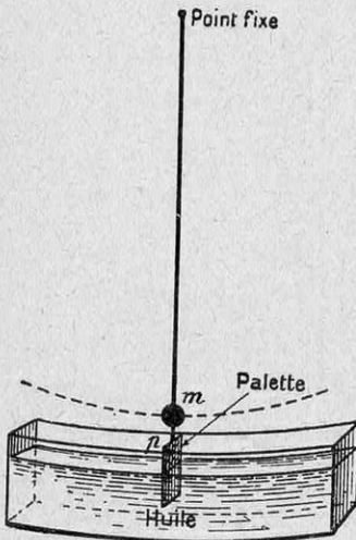
FIG. 16. — DISPOSITIF D'AMORTISSEMENT D'UN PENDULE, PAR IMMERSION PLUS OU MOINS GRANDE DE LA PALETTE « P » DANS L'HUILE
