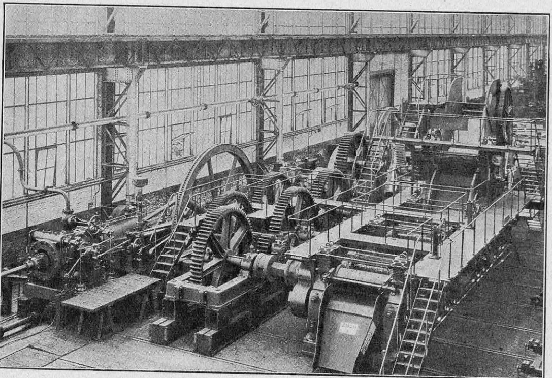
FIG. 4. — CET AUTRE MOULIN, CAPABLE DE BROYER SEULEMENT 600 TONNES DE CANNES A SUCRE PAR JOUR, EST ACTIONNÉ PAR LA MACHINE A VAPEUR VISIBLE A GAUCHE
