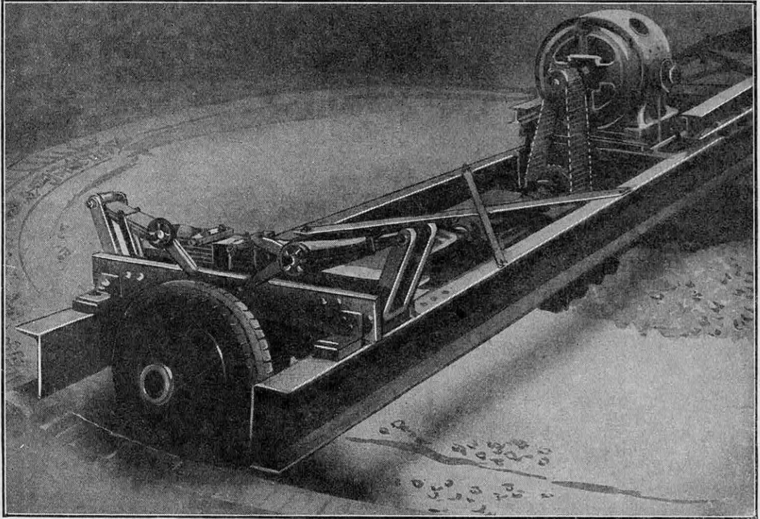
FIG. 3. — AVANT D'ÊTRE FABRIQUÉS EN SÉRIE, LES MODÈLES DE PNEUMATIQUES SUBISSENT DES ESSAIS RIGoureux, DANS LES CONDITIONS LES PLUS VOISINES POSSIBLE DE LA PRATIQUE
