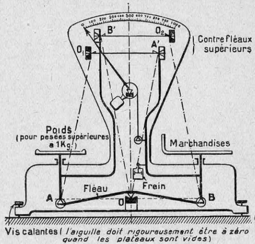
FIG. 25. — BALANCE SEMI-AUTOMATIQUE, MÉCANISME ROBERVAL, A CONTRE-FLÉAUX SUPÉRIEURS
