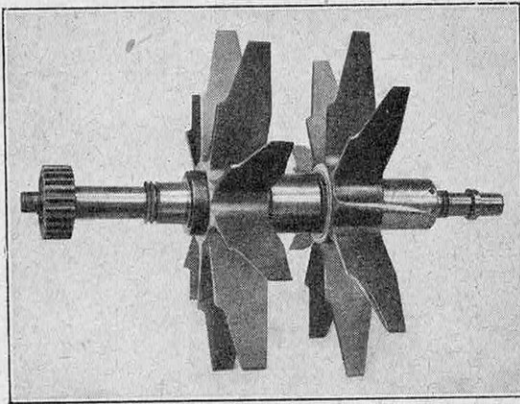
VOICI LES DEUX GROUPES D'AUBES MOBILES D'UN COMPRESSEUR A DEUX ETAGES
