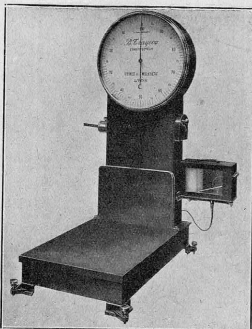
FIG. 33. — BASCULE AUTOMATIQUE AVEC « CHRONO ENREGISTREUR » INSCRIVANT L'HEURE EXACTE DE CHAQUE PESÉE
