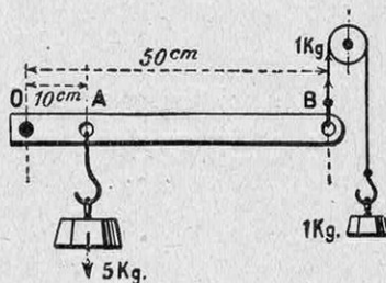
FIG. 5. - LEVIER DU DEUXIEME GENRE
