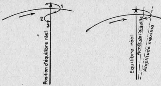
FIG. 21 ET 22. — AMORTISSEMENT CORRECT (A GAUCHE) ET AMORTISSEMENT INCORRECT DE L'AIGUILLE INDICATRICE (A DROITE)
