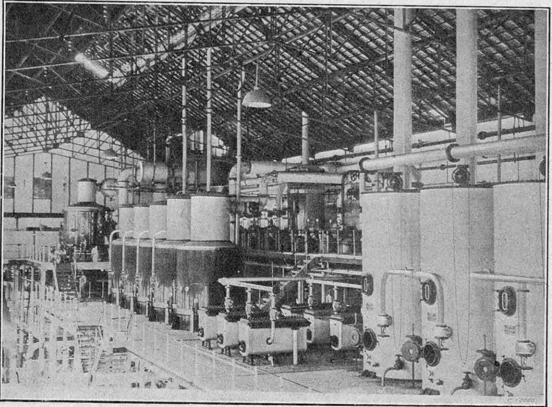
FIG. 1. — VUE INTÉRIEURE D'UNE SUCRERIE, AVEC LES APPAREILS DE CARBONATATION, D'ÉVAPORATION ET DE CUISSON (1)
