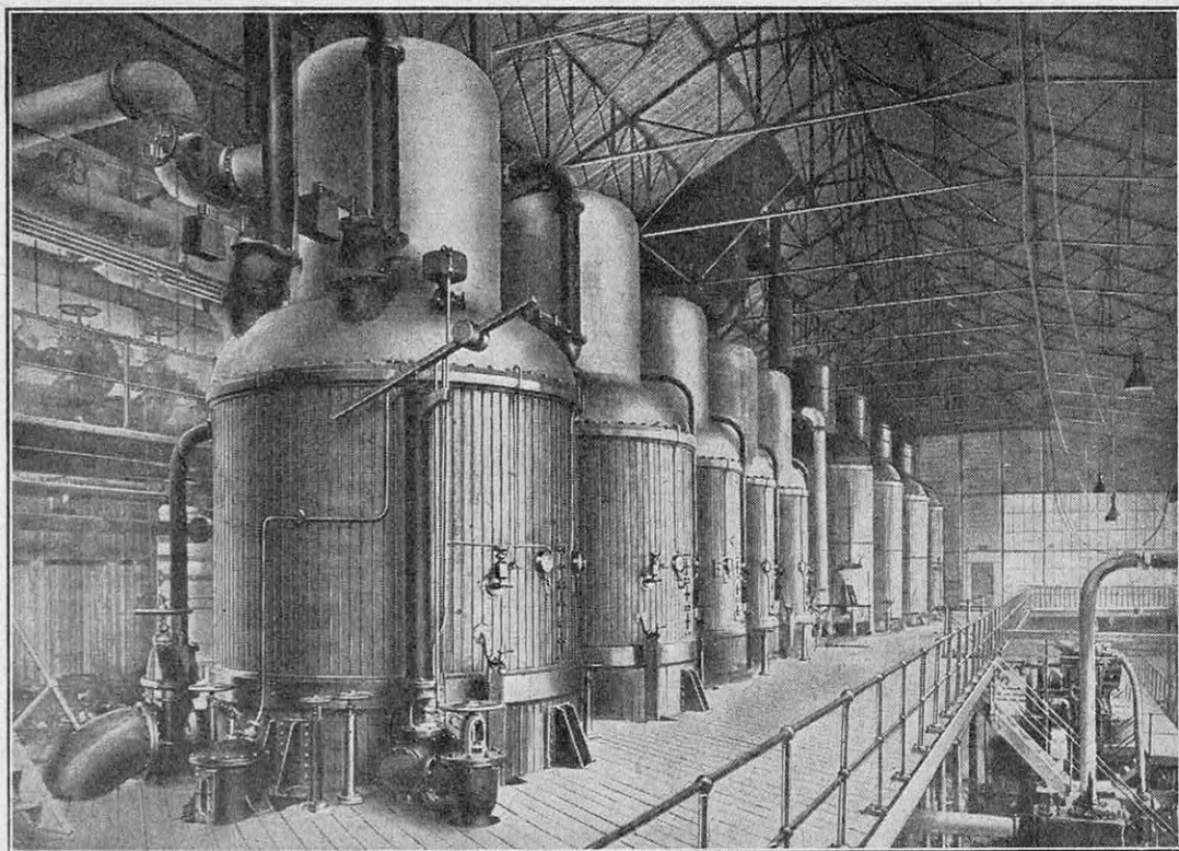
FIG. 5. — APPAREIL A CINQ « CAISSES » POUR L'ÉVAPORATION DES JUS SUCRÉS
