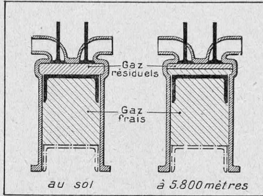
SCHÉMA D'UN CYLINDRE EN COUPE MONTRANT LE VIDAGE PLUS PARFAIT DES GAZ RÉSIDUELS A HAUTE ALTITUDE
