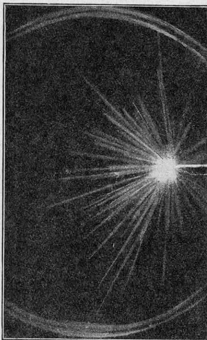
FIG. 3. — INSTANTANÉ PHOTOGRAPHIQUE DES CHOCs MOLÉCULAIRES RÉSULTANT DE L'ÉMISSION DE CORPUSCULES « ALPHA » DANS UN ESPACE SATURÉ DE VAPEUR D'EAU
