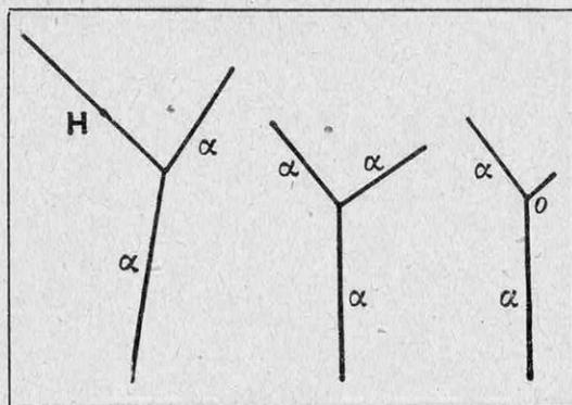
FIG. 4. — VOICI, D'APRÈS LE PHYSICIEN ANGLAIS BLACKWELL, COMMENT LES CORPUSCULES « ALPHA » SONT DÉVIÉS PAR DIVERS CORPS : HYDROGÈNE, HÉLIUM, OXYGÈNE
