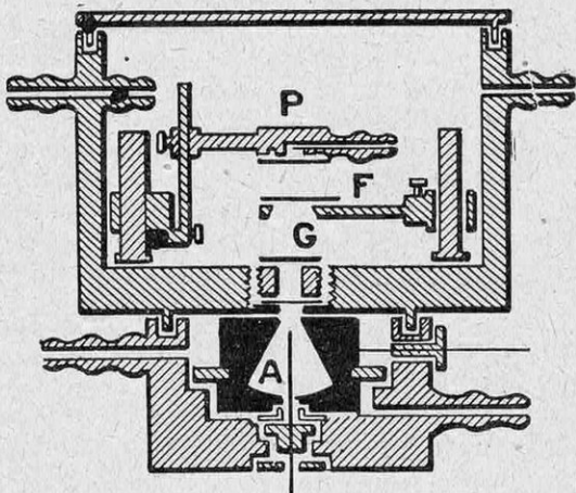
FIG. 6. — APPAREIL EMPLOYÉ PAR LES DEUX PHYSICIENS FRANÇAIS MAURICE DE BROGLIE ET LEPRINCE-RINGUET, POUR ÉTUDIER AVEC PRÉCISION LES PHÉNOMÈNES DE DÉSINTÉGRATION DES ATOMES
