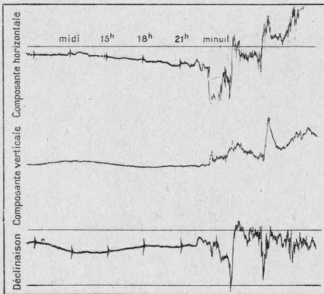
COURBES ENREGISTRÉES A L'OBSERVATOIRE DU VALJOYEUX, PRÈS DE PARIS, LORS D'UNE DES PLUS FORTES PERTURBATIONS MAGNÉTIQUES DE CES DERNIÈRES ANNÉES (JUILLET 1928)
