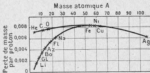
FIG. 1. — COURBE MONTRANT LA PERTE D'ÉNERGIE QUE CHAQUE PROTON A DU SUBIR DU FAIT DES CONDENSATIONS DU NOYAU ATOMIQUE DANS LES DIFFÉRENTS CORPS SIMPLES
