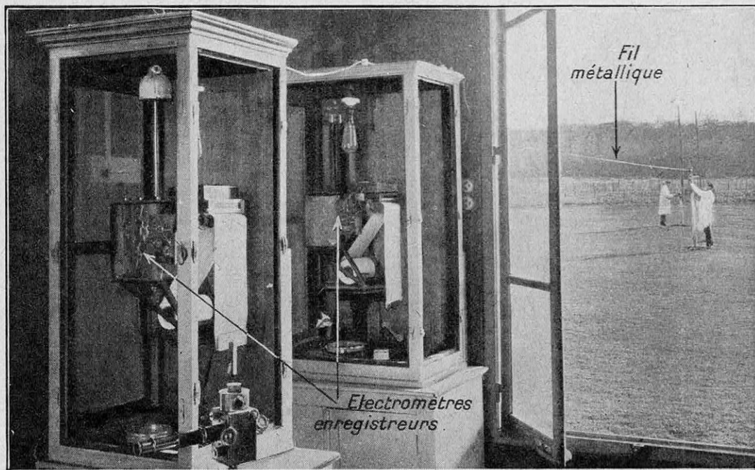
MESURE ET ENREGISTREMENT DU CHAMP ÉLECTRIQUE DE L'ATMOSPHÈRE, A L'OBSERVATOIRE DU VAL-JOYEUX, PRÈS DE PARIS
