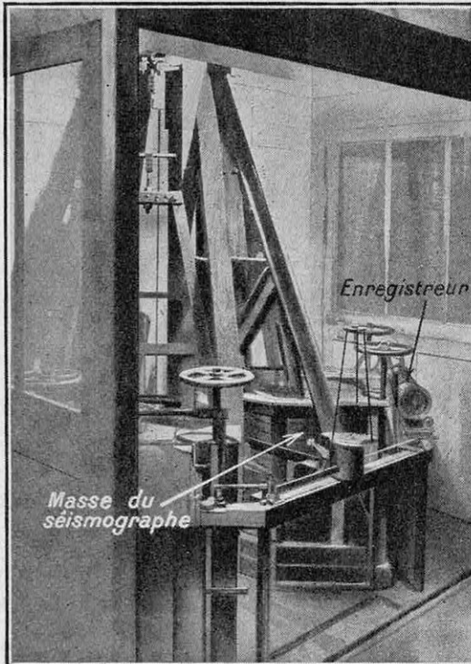
ENSEMBLE DU SÉISMOGRAPHE MAINKA EN SERVICE A L'OBSERVATOIRE DU PARC-SAINT-MAUR, PRÈS DE PARIS
