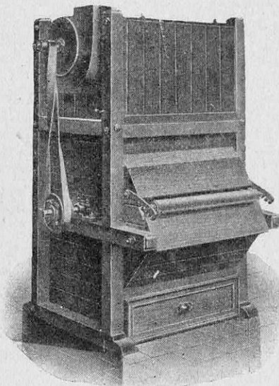
LA MACHINE A NETTOYER LES SACS
