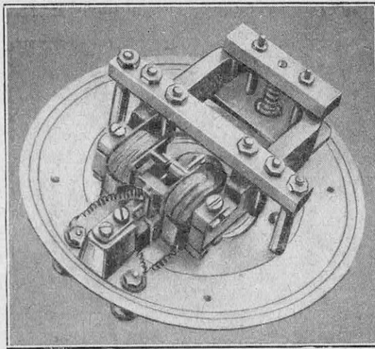
LE HAUT-PARLEUR AL-MA
