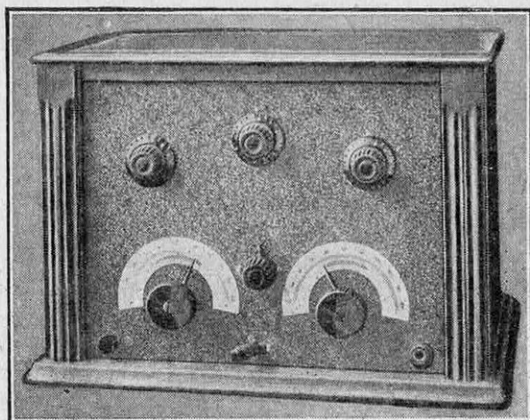
LE RADIOMODULATEUR BIGRILLE DUCRETET
