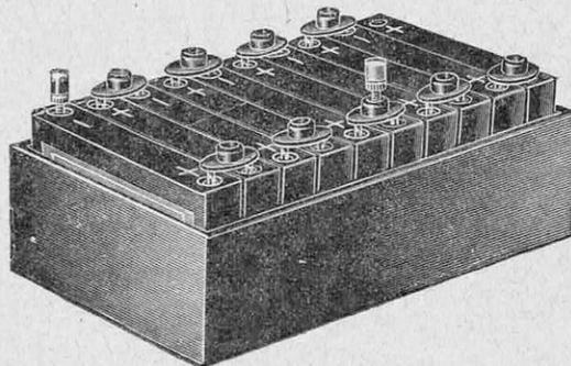
LA BOITE DE PILES HYDRA
