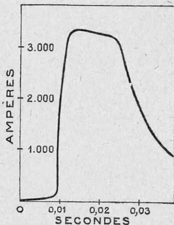
FIG. 4. - GRAPHIQUE DU COURANT DE DÉCHARGE ENREGISTRÉ A L'OSCILLOGRAPHE
