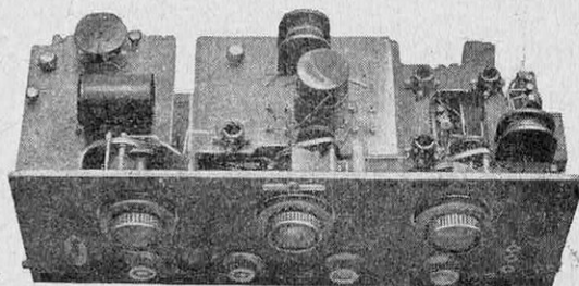
INTÉRIEUR DU POSTE RADIOMUSE
