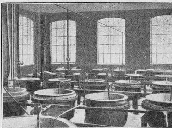
FIG. 4. — VUE D'UNE PARTIE DE L'ATELIER DE CRISTALLISATIONS DU SEL RADIFÈRE (OOLEN)
