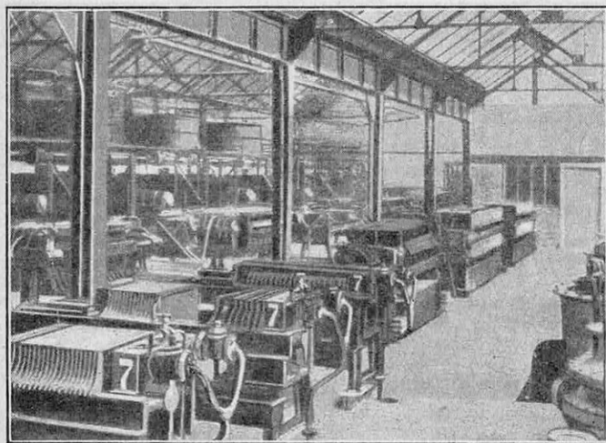
FIG. 3. — TRAITEMENT DE LA PECHBLENDE DANS LES CUVES ET FILTRES-PRESSES (USINE D'OOLEN, BELGIQUE)
