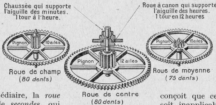
LES TROIS ENGRENAGES MULTIPLICATEURS QUI CONSTITUENT LE ROUAGE
