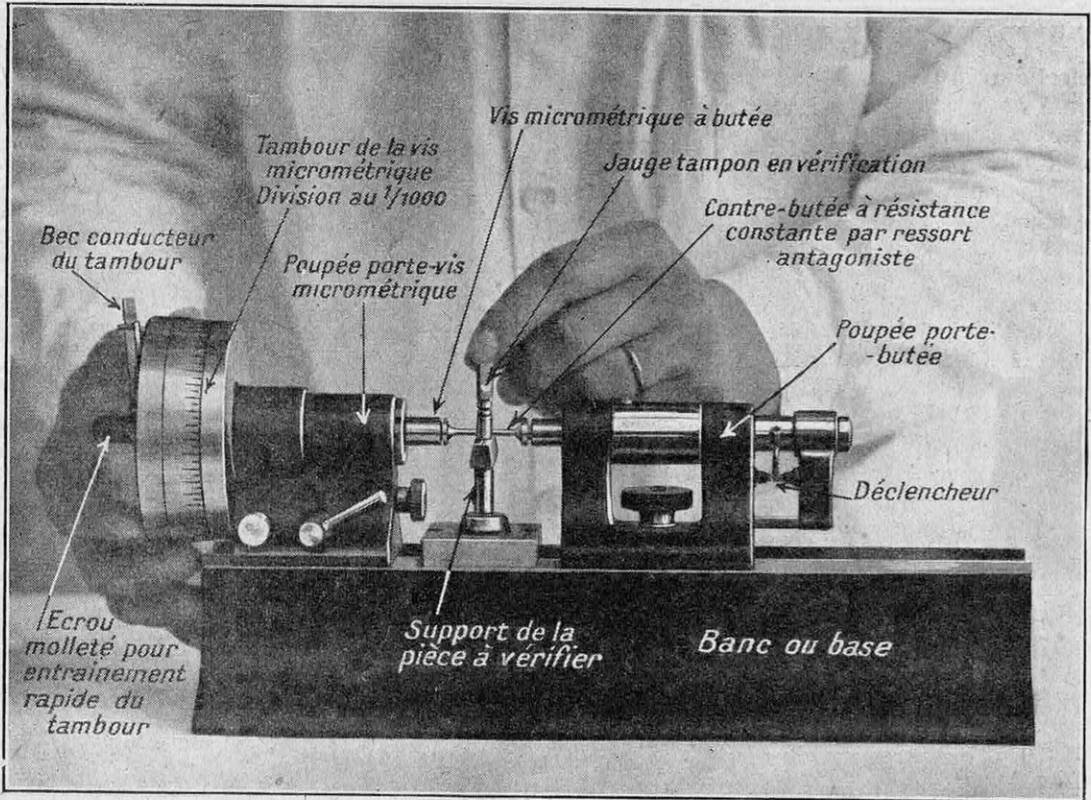
COMPARATEUR AU MILLIÈME DE MILLIMÈTRE (ZÉNITH)
