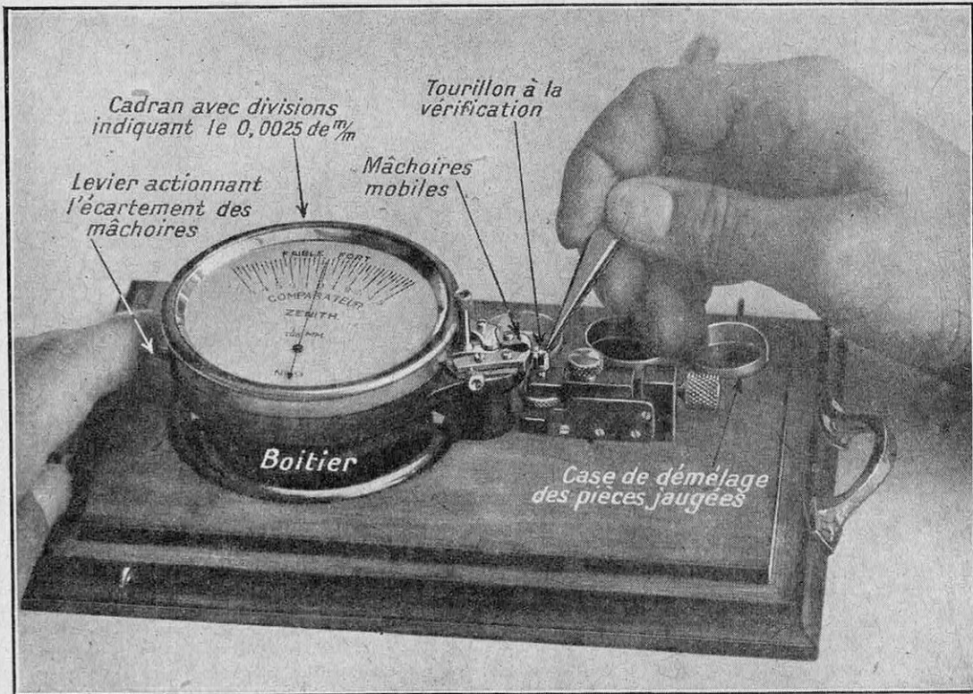
COMPARATEUR AU CENTIÈME DE MILLIMÈTRE
