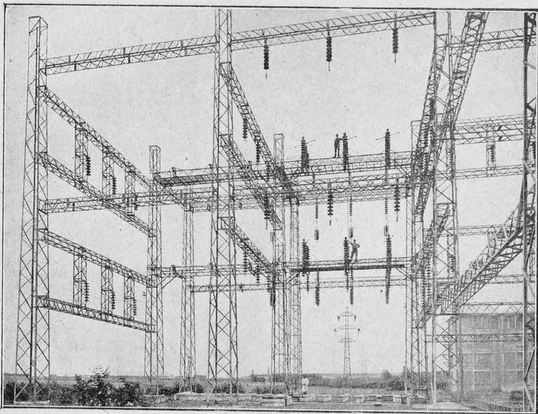
FIG. 7. — CETTE VUE D'UN POSTE 120.000 VOLTS, EN COURS DE MONTAGE, MONTRE BIEN LES GRANDES DIMENSIONS DES CHAINES D'ISOLATEURS QUI SUPPORTENT LES LIGNES A TRÈS HAUTE TENSION, A 25 MÈTRES DE HAUTEUR
