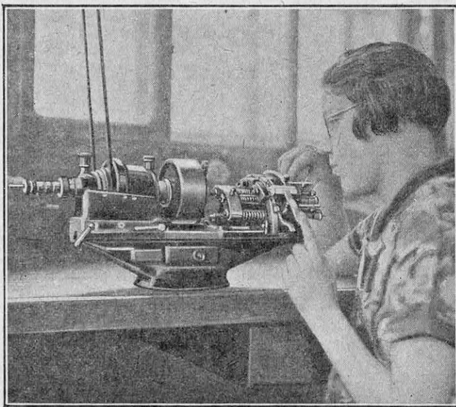
TOUR A BURIN POUR CREUSER LES PLATINES (OMÉGA)
