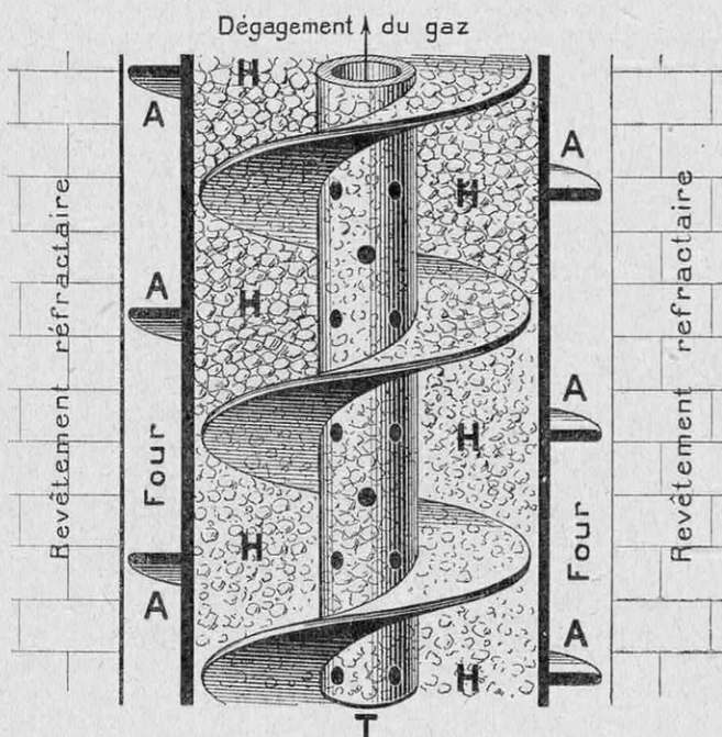
UN PROCÉDÉ AMÉRICAIN UTILISÉ SUR UNE GRANDE ÉCHELLE, A DENVER (COLORADO), POUR LA DISTILLATION DE LA HOUILLE A BASSE TEMPÉRATURE
