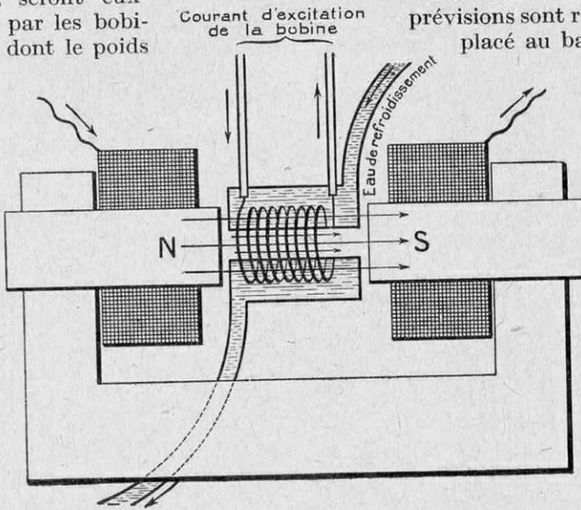
FIG. 2. — PRINCIPE DE L'ELECTRO « PASTEUR »
