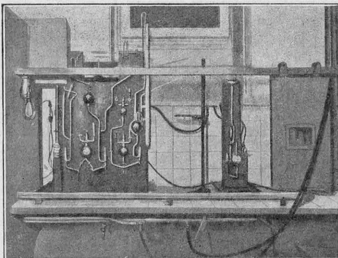
FIG. 10. — APPAREIL SERVANT A L'EXTRACTION, A LA PURIFICATION ET A LA CONCENTRATION DE L'ÉMANATION
