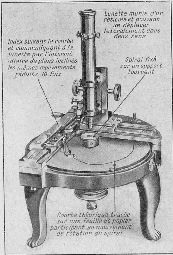
LE « CAMPYLOSCOPE »
