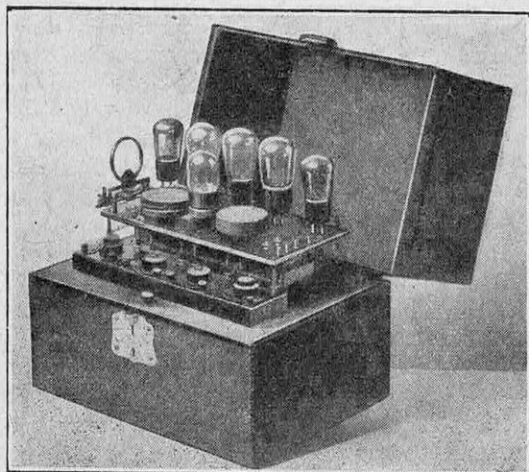
LE BIGRILLE MODULADYNE D'HORACE HURM
