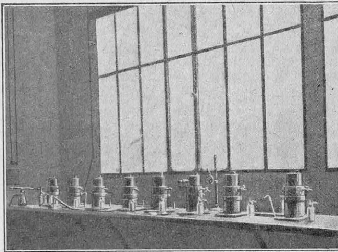
FIG. 7. — LABORATOIRE INDUSTRIEL DE MESURES Salle des électroscopes de l'usine de Nogent-sur-Marne.
