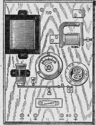
"TABLEAU A VIBREUR" 4 et 80 V. 4 A.
