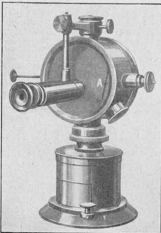
FIG. 6. — ÉLECTROSCOPE POUR MESURES RADIOACTIVES DE MM. CHÉNEVEAU ET LABORDE
