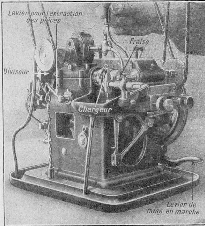
MACHINE A TAILLER LES ROUES DE REMONTOIRS
