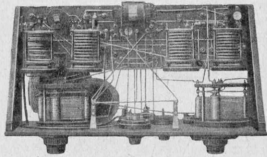
LE SUPERHÉTÉRODYNE GODY
