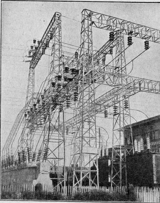
FIG. 4. — VUE DES « BARRES » AÉRIENNES A 60.000 VOLTS ALIMENTANT LES TRANSFORMATEURS-ABAISSEURS D'UNE SOUS-STATION DE TRACTION
