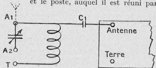
DISPOSITIF PERMETTANT DE RENDRE UN POSTE PLUS SÉLECTIF
