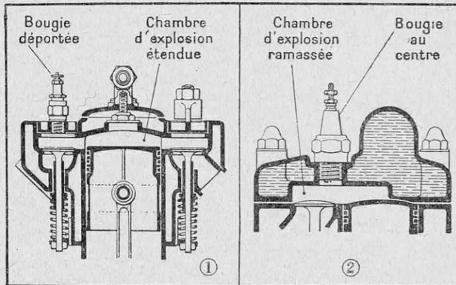
FIG. 2. — CULASSE D'UN MOTEUR ANCIEN A SOUPAPES SYMÉTRIQUES ET CULASSE D'UN MOTEUR MODERNE A SOUPAPES LATÉRALES
