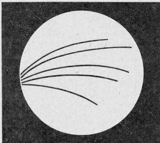
FIG. 5. — COURBURE DES RAYONS ALPHA DU RADIUM, DANS UN CHAMP DE 130.000 GAUSS La vitesse de ces rayons atteint 15.000 kilomètres par seconde.
