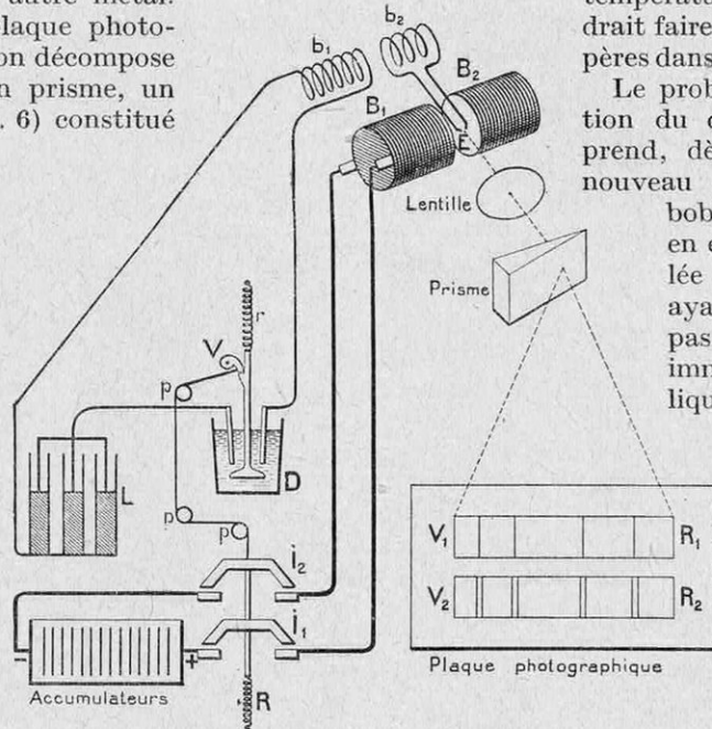
FIG. 6. — EXPÉRIENCE DE KAPITZA
