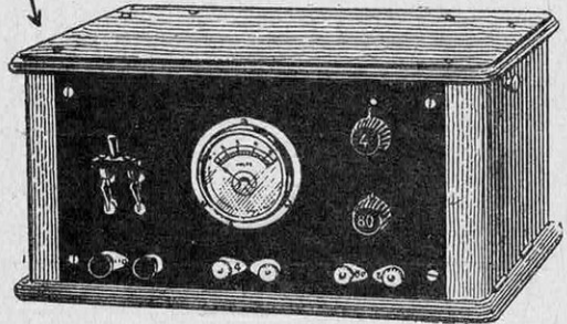
"BOITE D'ALIMENTATION TOTALE" 4 et 80 V.
