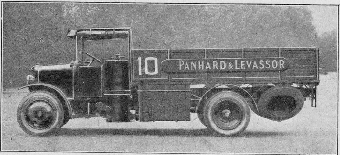
CAMION AUTOMOBILE ÉQUIPÉ AVEC UN GAZOGÈNE PANHARD
