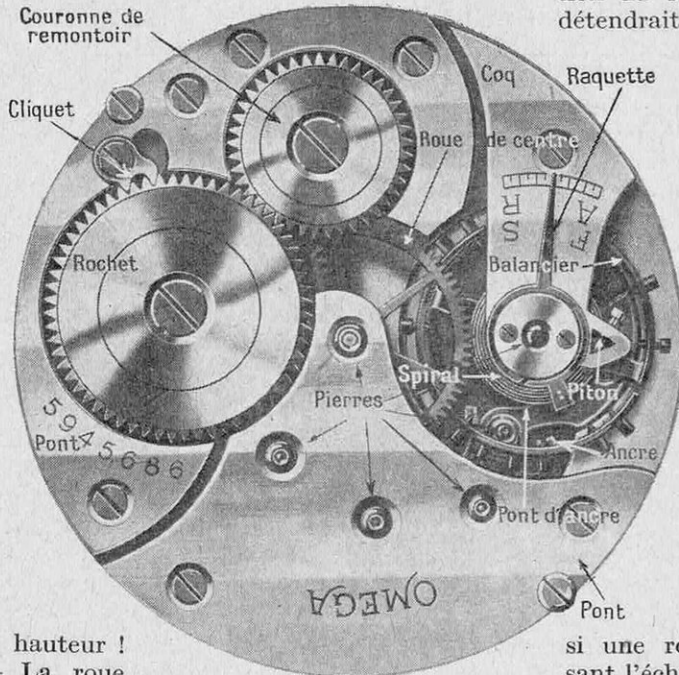
CE QUE L'ON VOIT QUAND ON OUVRE LE BOITIER INTÉRIEUR D'UNE MONTRE
