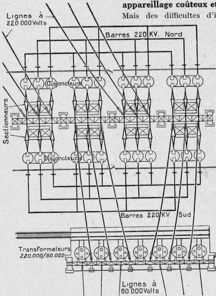
FIG. 3. — DISPOSITION SCHEMATIQUE DES APPAREILS D'UN POSTE DE COUPURE SUR LIGNE A 220 KILOVOLTS (220.000 VOLTS), AVEC TRANSFORMATEURS-ABAISSERS A 60.000 VOLTS ALIMENTANT UN RESEAU SECONDAIRE
