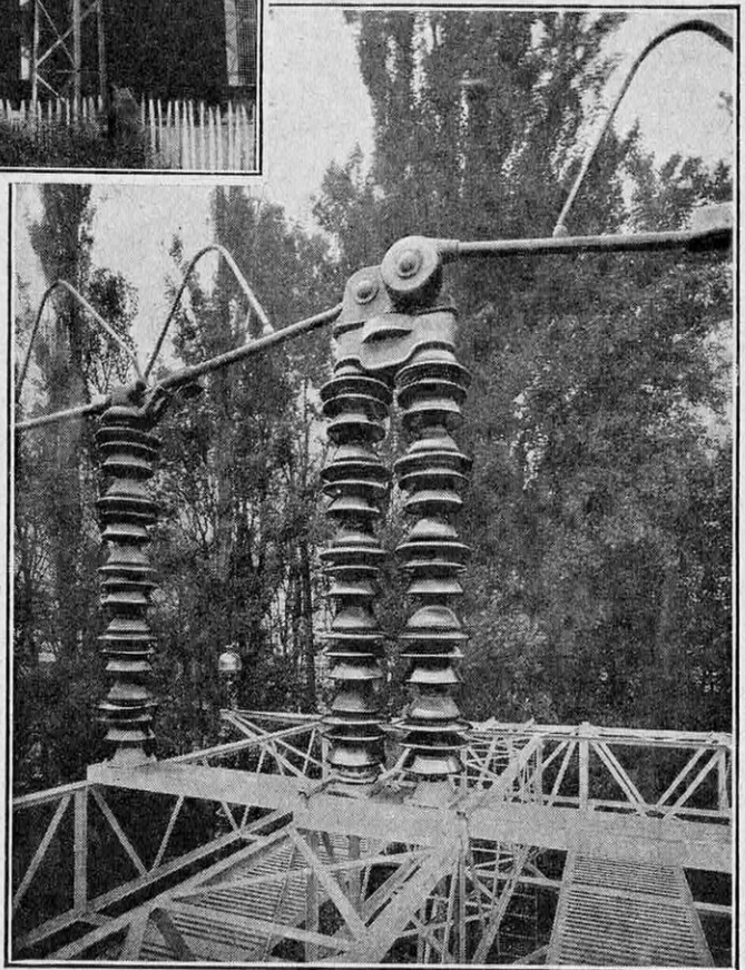
FIG. 5. — SECTIONNEURS A 120.000 VOLTS PERMETTANT DE COUPER DIRECTEMENT LE COURANT SUR LES LIGNES Placés à environ 20 mètres au-dessus du sol, la commande peut en être effectuée par de longues tringles de manœuvre.
