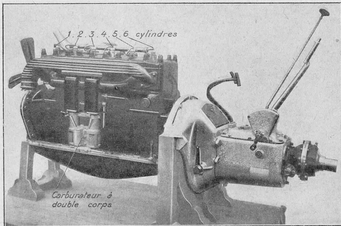
FIG. 1. - MOTEUR A 6 CYLINDRES FORMANT BLOC AVEC L'EMBRAYAGE ET LA BOITE DES VITESSES Le 6 cylindres est préféré pour sa souplesse, sa douceur d'entraînement et son fonctionnement silencieux. Il augmente l'agrément de marche de la voiture et le confort des passagers (bloc-moteur 6 cylindres Berliet).
