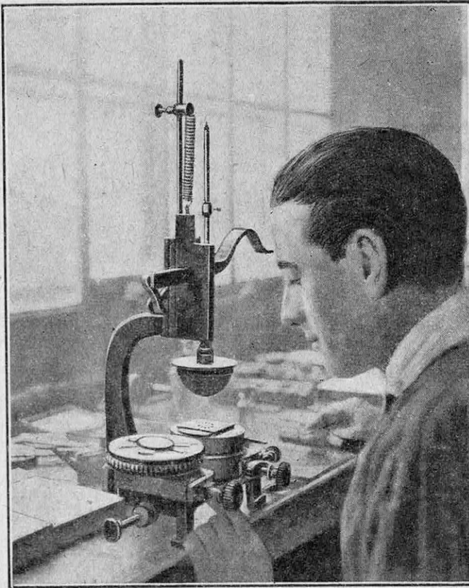
APPAREIL A IMPRIMER LES HEURES SUR LES CADRANS DE MONTRES
