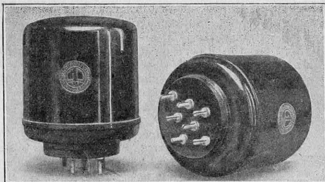
SELF « UNIVOQUE » POUR MONTAGES A ÉTAGES MULTIPLES ET A RÉGLAGE UNIQUE (ÉLECTRONS)
