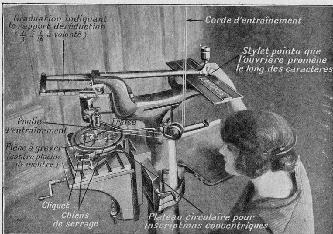
PANTOGRAPHE POUR GRAVER LES CONTRE-PLATINES DE MONTRES
