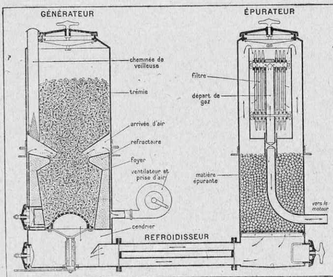
VUE EN COUPE DU GAZOGÈNE PANHARD
