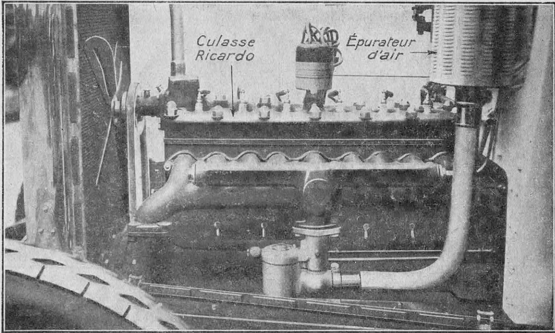
FIG. 3. — UN MOTEUR MODERNE A 6 CYLINDRES AVEC CULASSE RICARDO
