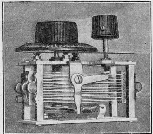
LE CONDENSATEUR PIVAL
