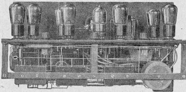
LE SUPERPHAL BIGRILLE 8 LAMPES
