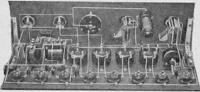
VUE INTÉRIEURE DU SUPERHÉTÉRODYNE
