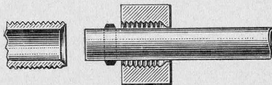
LE TUYAU A RACCORDER MUNI DE SA RONDELLE
