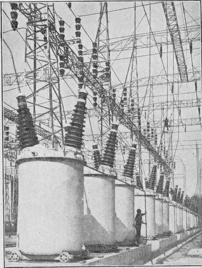
FIG. 6. — UNE SÉRIE DE DISJONCTEURS A 150.000 VOLTS Ces appareils à grande puissance sont unipolaires, c'est-à-dire un sur chaque conducteur. Les manœuvres d'enclenchement et déclenchement sont faites par commande automatique à distance. (Le dessin de notre couverture représente la partie supérieure de ces appareils, à plus grande échelle).
