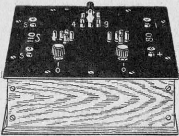
"RECTIFILTRE" pour tension-plaque 1, 2 ou 3 voltages.
