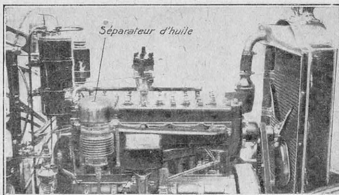
FIG. 5. — SÉPARATEUR D'HUILE
