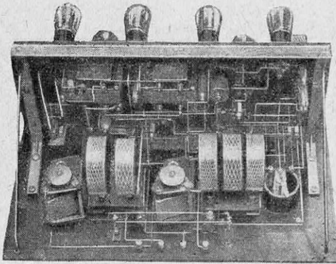
HYPERHÉTÉRODYNE LEMOUZY
