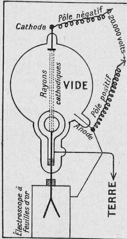
FIG. 1. - LA PREMIÈRE EXPÉRIENCE DE JEAN PERRIN (1895)
