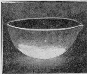
FIG. 12. — CAPSULE CONTENANT DU BROMURE DE RADIUM, PHOTOGRAPHIÉE EN CHAMBRE NOIRE PAR LA LUMINOSITÉ ÉMISE PAR LE RADIUM. (DIAMÈTRE DE LA CAPSULE : 350 MILLIMÈTRES) (Cliché communiqué par les usines d'Oolen, Belgique.)
