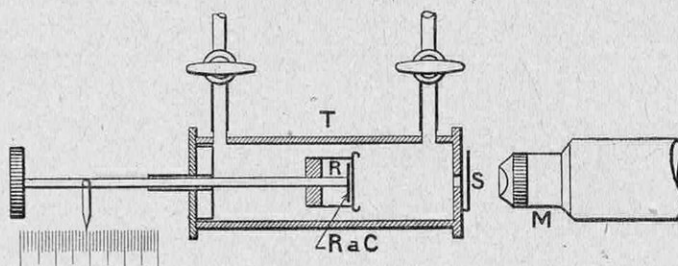
FIG. 8. — APPAREIL DE SIR E. RUTHERFORD POUR PRODUIRE LA DÉSINTÉGRATION ARTIFICIELLE DES ÉLÉMENTS PAR LES PARTICULES \alpha
