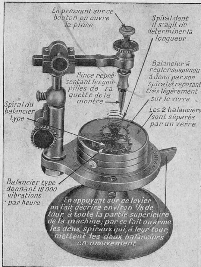
MACHINE A RÉGLER LES MONTRES Elle sert à déterminer la longueur du spiral, c'est-à-dire l'endroit où les goupilles de la raquette viendront limiter la partie utile du spiral (Longines).
