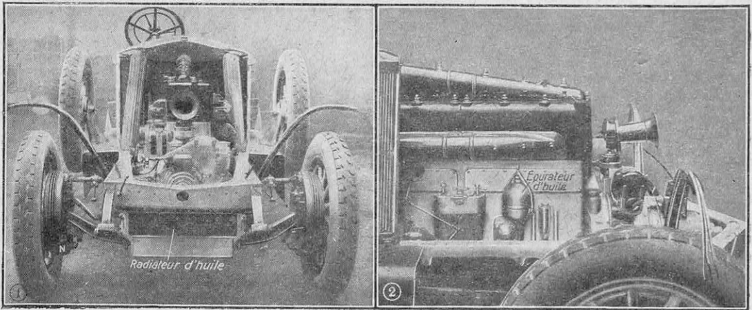
FIG. 4. — RADIATEUR ET ÉPURATEUR D'HUILE
