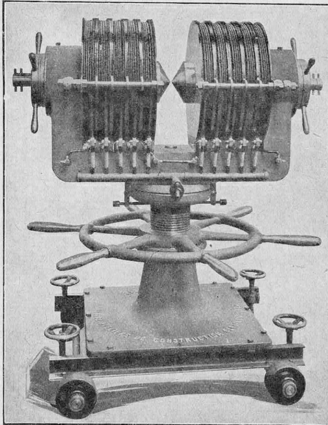
FIG. 1. — LE GROS ÉLECTRO-AIMANT DE WEISS
