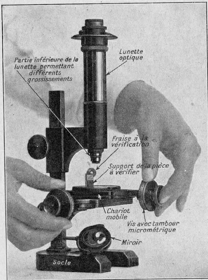
MICROSCOPE THURY ET AMEZ POUR VÉRIFIER LES PETITES PIÈCES (ZÉNITH)
