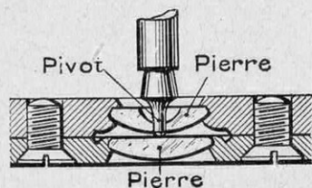
VOICI COMMENT SONT DISPOSÉES LES PIERRES DU PIVOT DU BALANCIER
