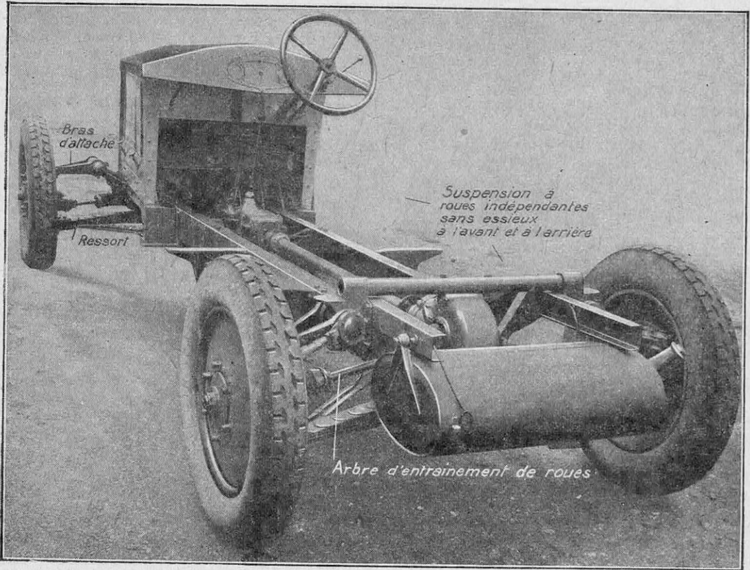
FIG. 6. — UN CHASSIS A ROUES INDÉPENDANTES
