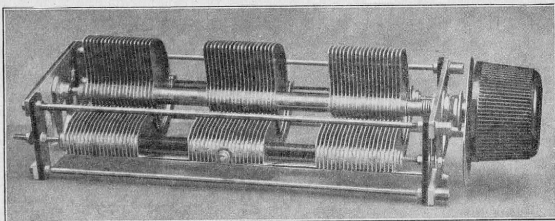
CONDENSATEUR TRIPLE « SQUARE LAW » POUR POSTES A COMMANDE UNIQUE (ÉLECTRONS)
