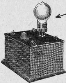
"REDRESSEUR-FILTRE" avec lampe biplaque redressant les 2 1/2 périodes pour toute tension de 30 à 250 V.
