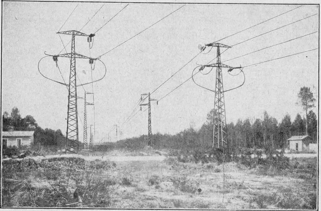
FIG. 2. — LIGNE DOUBLE A 150.000 VOLTS, ÉTABLIE PAR LES CHEMINS DE FER DU MIDI ENTRE BORDEAUX ET DAX
