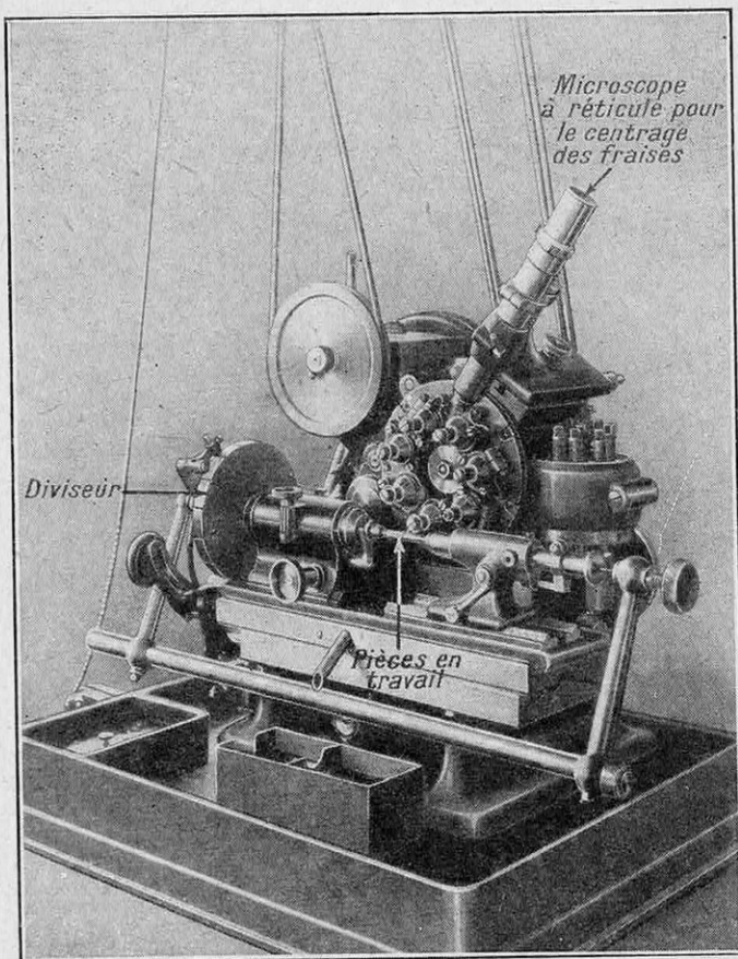
VUE D'ENSEMBLE DE LA MACHINE A TAILLER LA DENTURE DES ROUES D'ÉCHAPPEMENT (OMÉGA)
