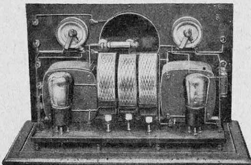
L'ULTRA-MODULATEUR LEMOUZY
