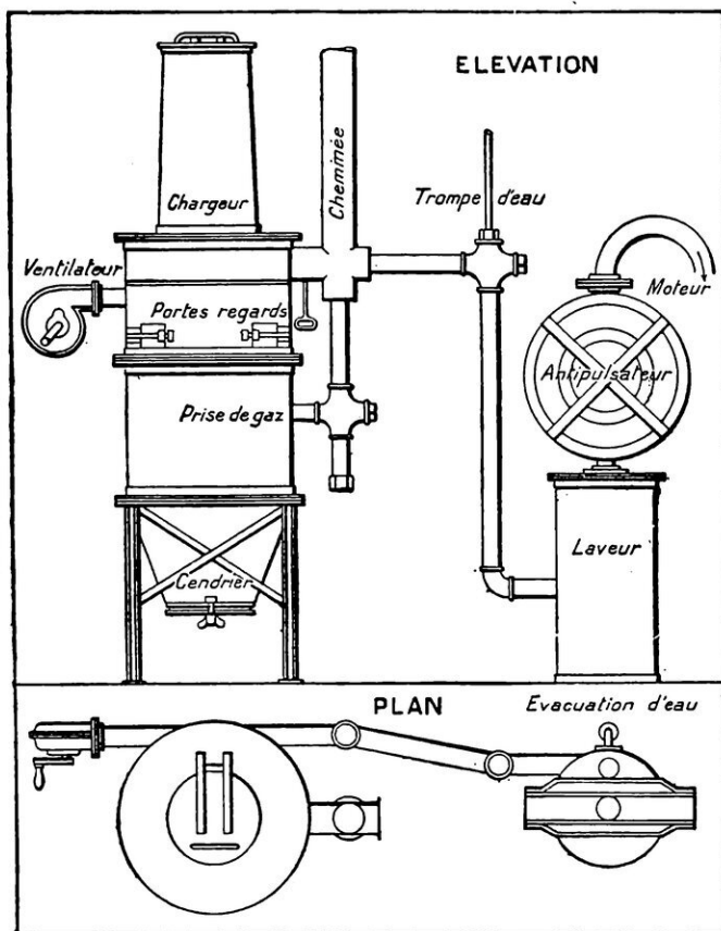
INSTALLATION D'UN GAZOMÈTRE AU BOIS DE 25 CHEVAUX Ce gazomètre brûle environ, par cheval, un kilogramme de bois, sciures, copeaux, branchages, etc.
