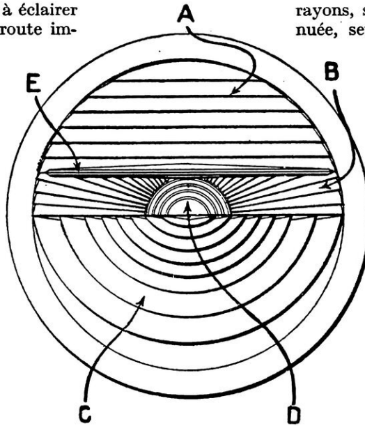
FIGURE SCHÉMATIQUE DES SYSTÈMES OPTIQUES Les systèmes A, B, C, D ont pour but de projeter les rayons lumineux horizontalement, sur les côtés et vers le bas, mais aucun vers le haut ; E est un abat-jour qui diffuse les rayons horizontaux supérieurs.
