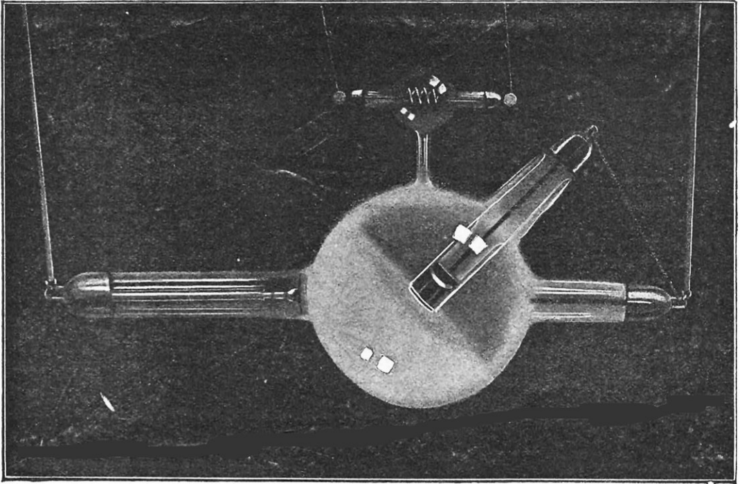
TUBE A FAIBLE INTENSITÉ POUR LES INSTALLATIONS TRANSPORTABLES Ce type est principalement utilisé dans les voitures radiologiques du Service de santé militaire.
