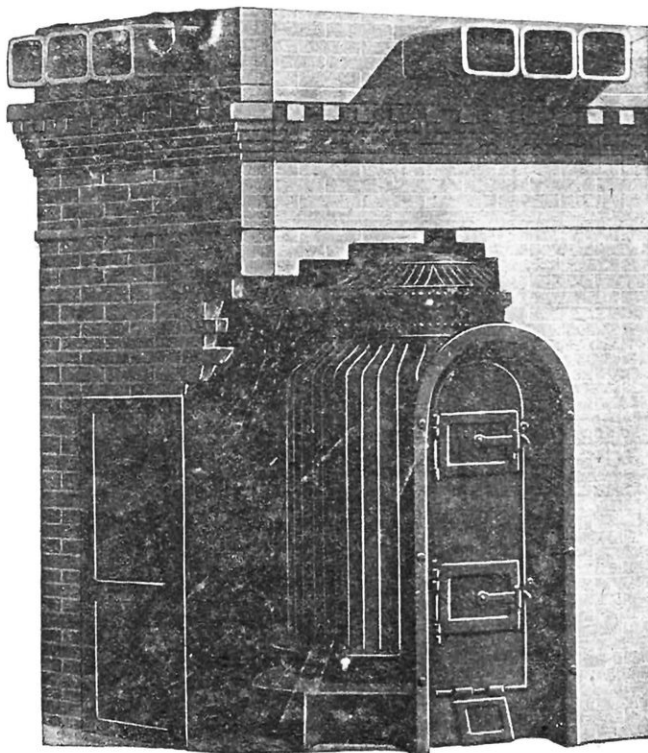
CALORIFÈRE GURNEY (MONTAGE DAVÈNE ET ROBIN)
