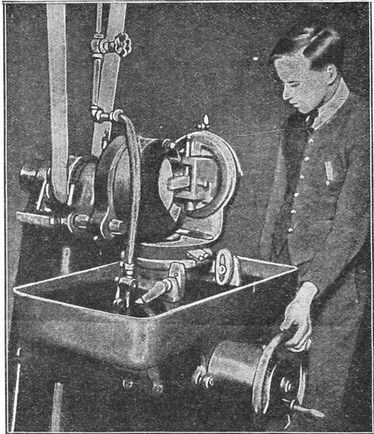
FIG. 15. — MACHINE A AFFÛTER
