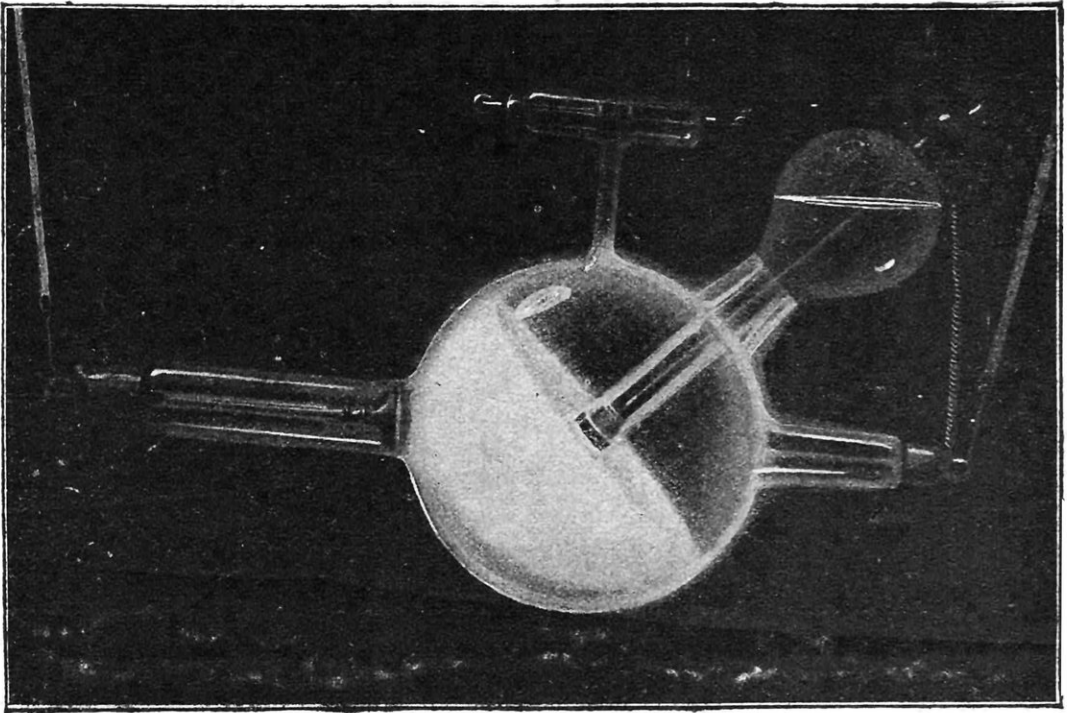
MODÈLE DE TUBE A RÉSERVOIR D'EAU POURVU D'UN RÉGULATEUR ÉLECTRIQUE
