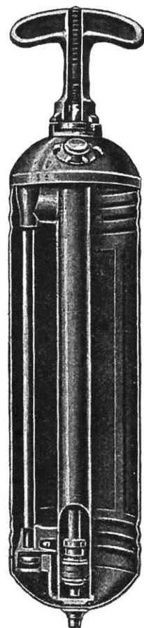
LE PYRÈNE Coupe partielle.
