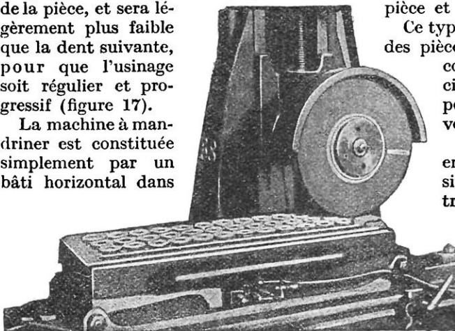
FIG. 16. — MACHINE A MEULER MUNIE D'UN PLATEAU A ADHÉRENCE MAGNÉTIQUE
