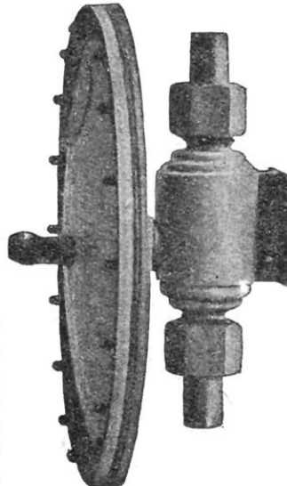
VUE EXTÉRIEURE DU PULSATEUR ET DE LA BOÎTE A CLAPETS
