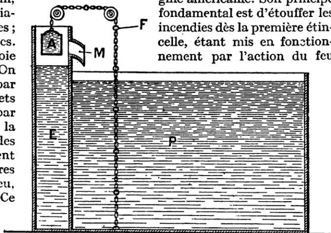
EXTINCTEUR AUTOMATIQUE POUR RÉSERVOIR A PÉTROLE E, colonne contenant le liquide destiné à produire la mousse ; A, acide dans un récipient suspendu par une chaîne ; F, un des anneaux en métal fusible placés de distance en distance sur la chaîne ; M, orifice de sortie de la mousse produite ; P, pétrole dans le réservoir à protéger. — Si le pétrole (ou tout autre combustible liquide) prend feu, la flamme fera fondre instantanément un des anneaux en métal fusible de la chaîne ; le récipient à acide A, n'étant plus soutenu, tombera dans le liquide E ; le mélange formera de la mousse en abondance qui sortira par M et tombera à la surface du pétrole dont les flammes, privées ainsi du contact de l'air, seront vite étouffées.
