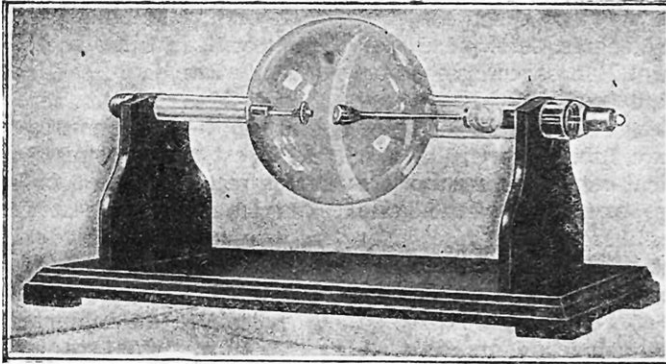
SPÉCIMEN PHOTOGRAPHIQUE DE TUBE « COOLIDGE »
