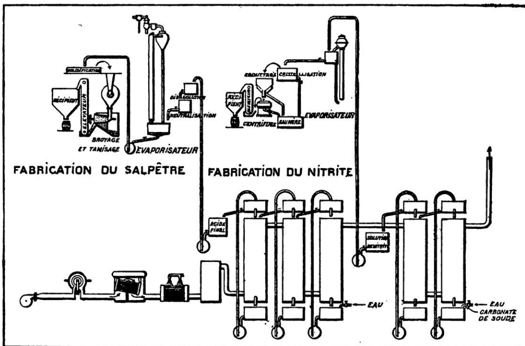
FIG. 12. — INSTALLATION SCHEMATIQUE DE LA PRÉPARATION DE L'ACIDE NITRIQUE On prépare par les mêmes procédés électro-chimiques le nitrate de chaux et le nitrate de soude.
