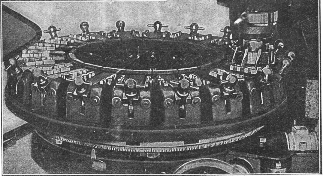
FIG. 13. — MACHINE A FRAISER PERMETTANT L'USINAGE CONTINU
