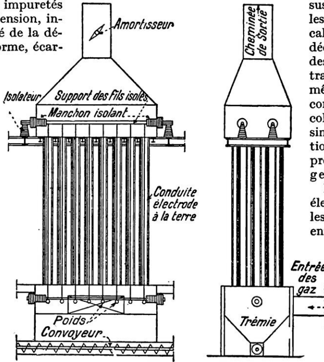
PRÉCIPITATEUR A CONDUITES MULTIPLES
