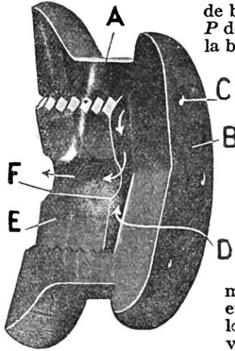
COUPE AGRANDIE DE LA SOUPAPE
