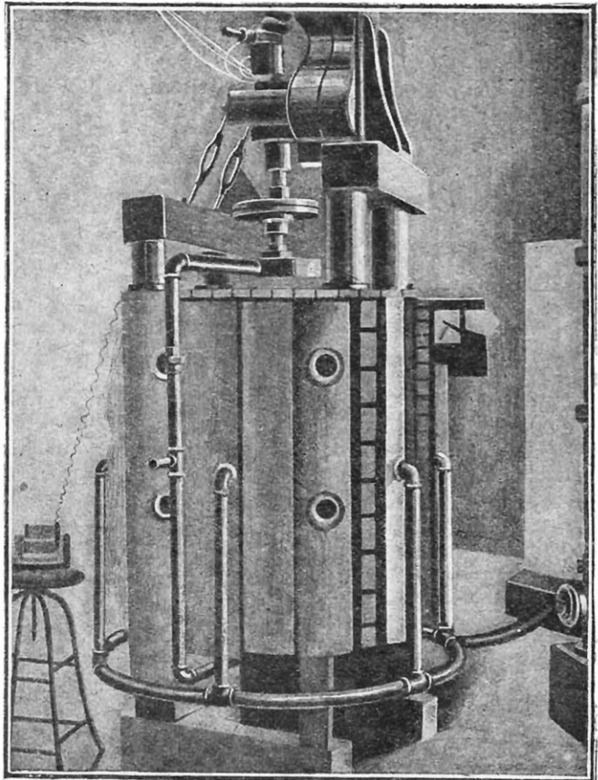
FIG. 3. — VUE D'ENSEMBLE D'UN APPAREIL BRADLEY
