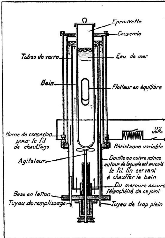
COUPE DE L'INSTRUMENT PERMETTANT DE DÉTERMINER LA DENSITÉ DE L'EAU DE MER
