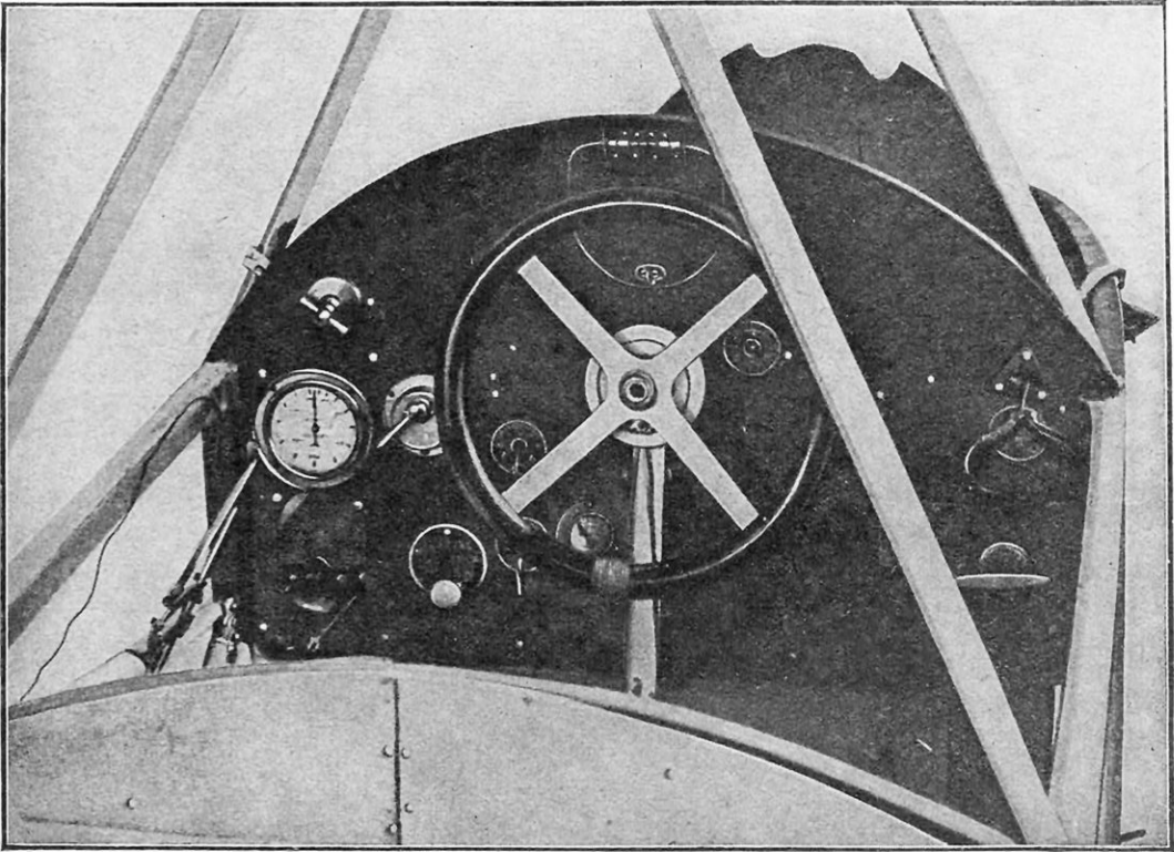
POSTE DE PILOTAGE SUR UN AVION ALLEMAND DU TYPE « RUMPLER »
