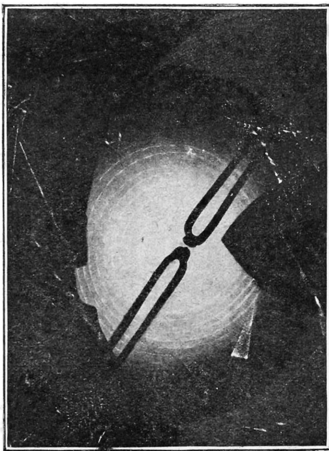
FIG 7 bis. — DISQUE LUMINEUX PRODUIT, DANS LE PROCÉDÉ BIRKELAND, PAR DES ÉLECTRODES CREUSES EN CUIVRE
