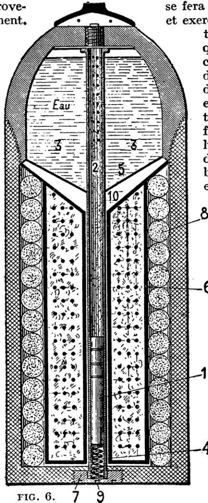
PROJECTILE A ACÉTYLÈNE
