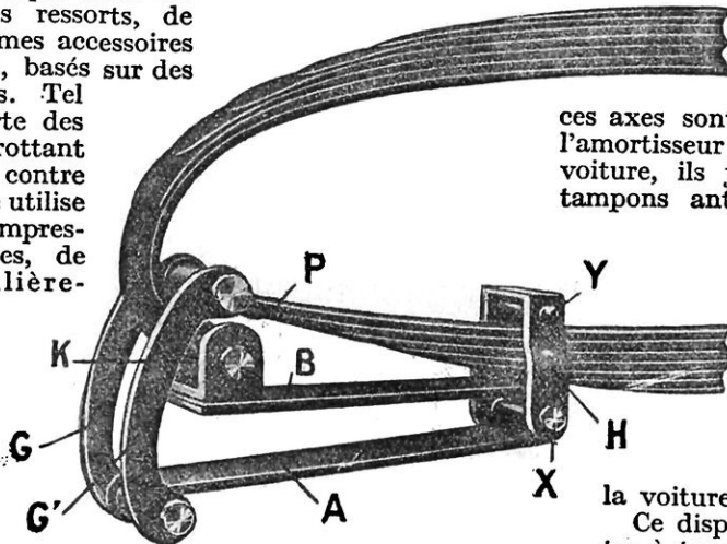
DISPOSITIF DE L'AMORTISSEUR G. P.
