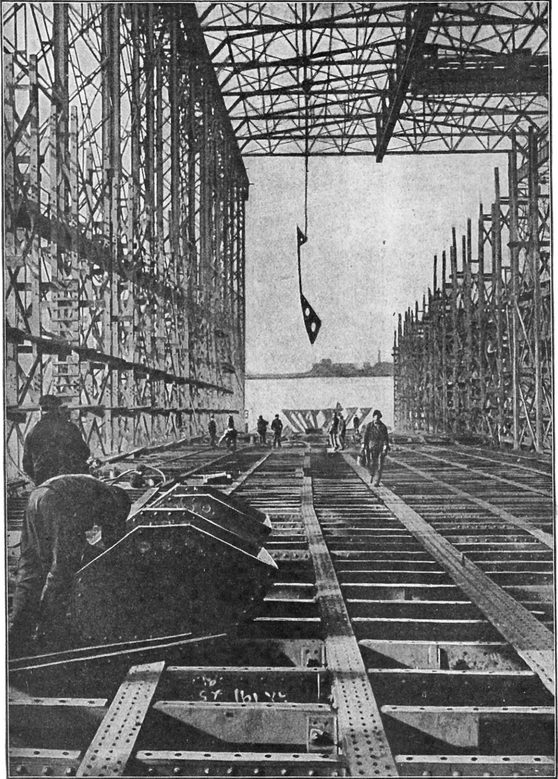
LE FOND ET LES PAROIS D'UN BATEAU EN CONSTRUCTION A HOG ISLANG
