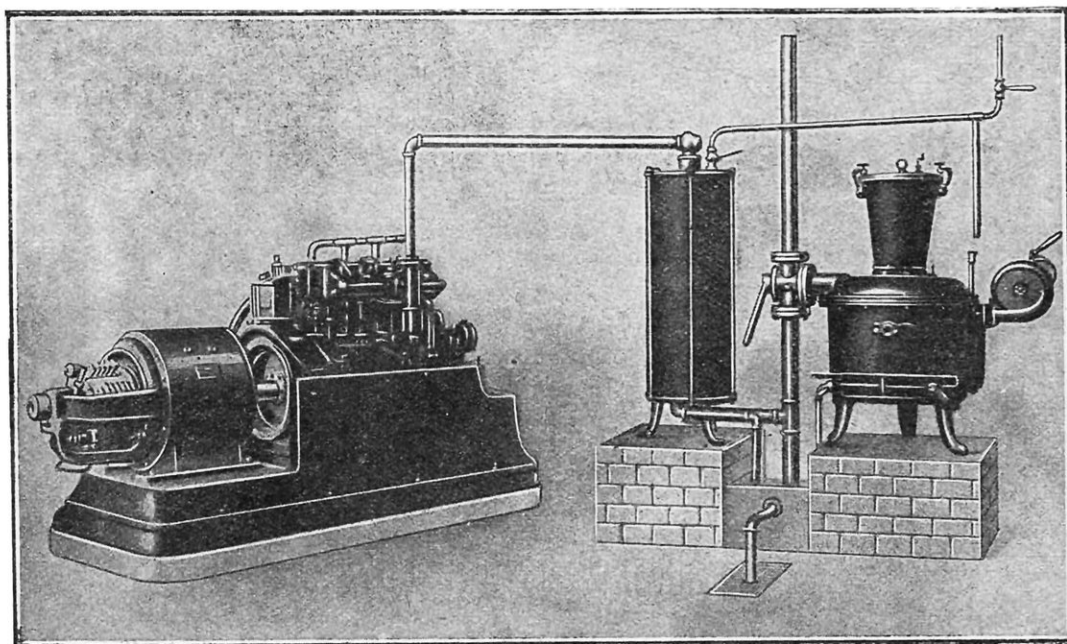
INSTALLATION COMPLÈTE D'UN GROUPE ÉLECTROGÈNE A GAZ PAUVRE
