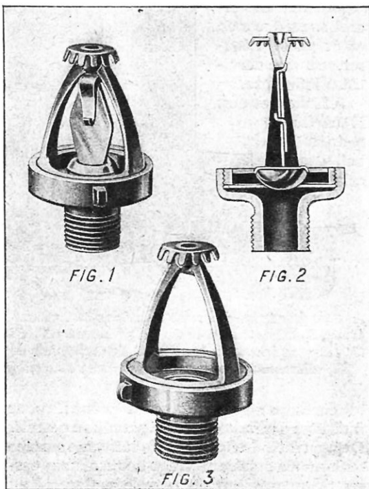
TÊTES DU DISPOSITIF GRINNELL
