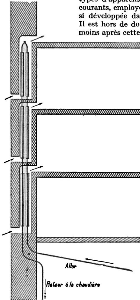
Schéma d'une installation de chauffage indirect par batteries enfermées dans des coffrages formant gaines (système Anceau).
