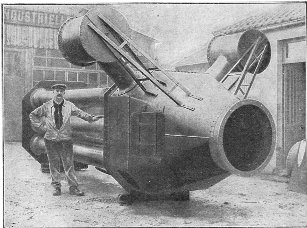
APPAREIL SPÉCIAL DE PURIFICATION POUR CHEMINÉE DE NAVIRE
