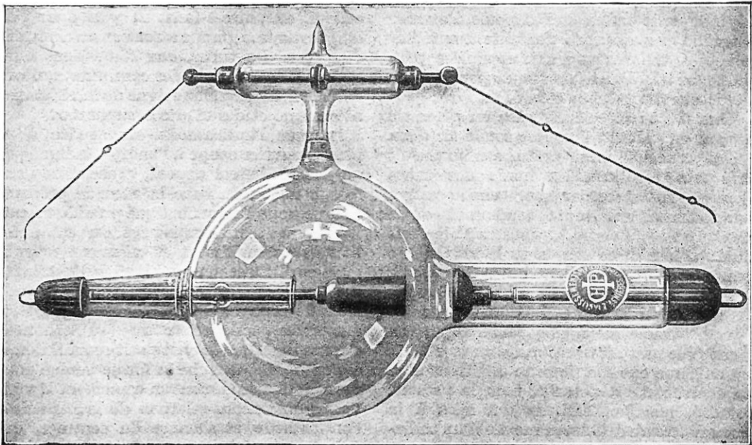
MODÈLE DE TUBE OU SOUPAPE DESTINÉE A ÉLIMINER LE COURANT DE SENS INVERSE
