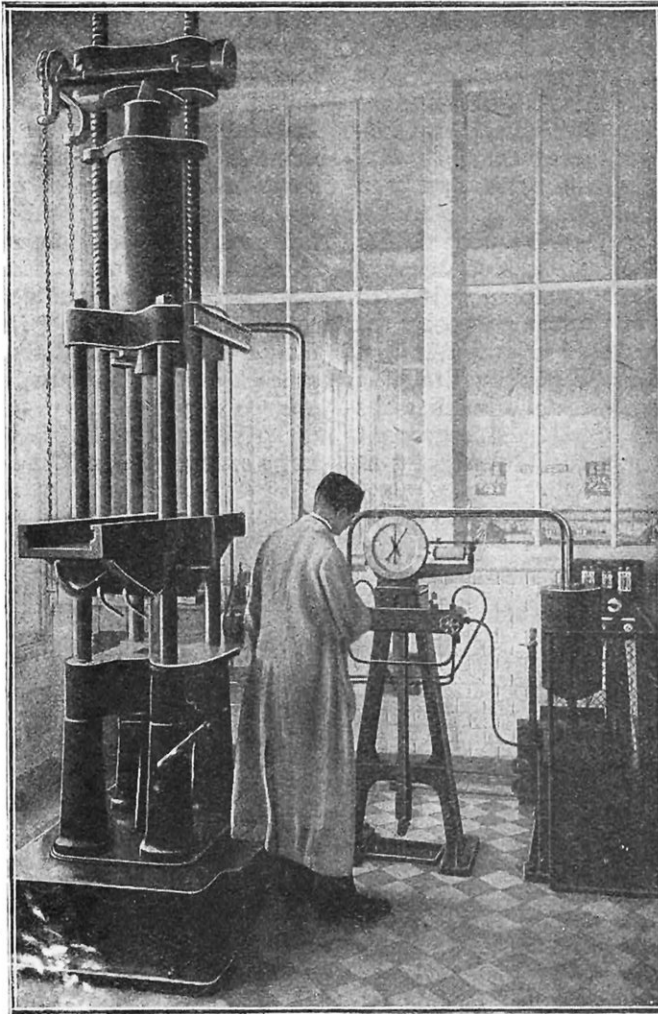
MACHINE A TRACTION AMSLER, DE 50 TONNES Cette machine, dont tout laboratoire sérieux est doté, permet des essais de traction, compression, flexion, pliage et dureté.
