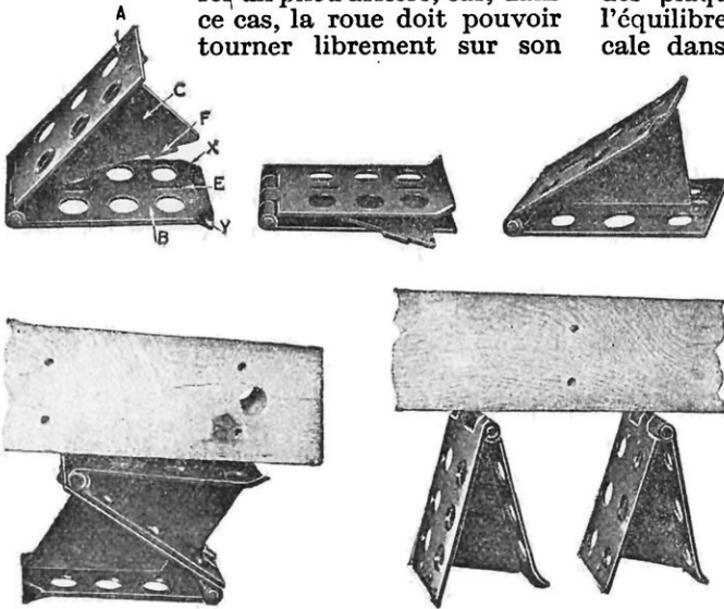
LES DIVERS MODES D'EMPLOI DE LA CALE PLIANTE
