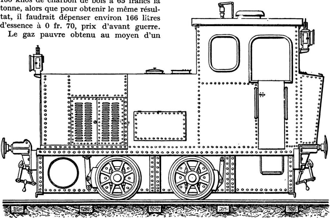
LOCOMOTEUR A GAZ PAUVRE POUR CHEMIN DE FER A VOIE ÉTROITE
