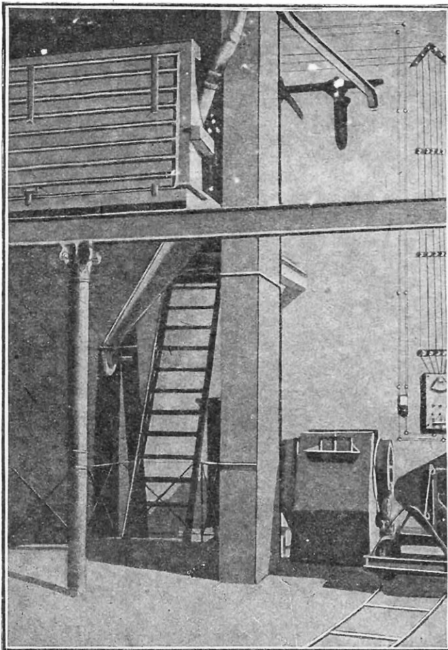
FIG. 13. — ATELIER DE BROYAGE DE LA CYANAMIDE
