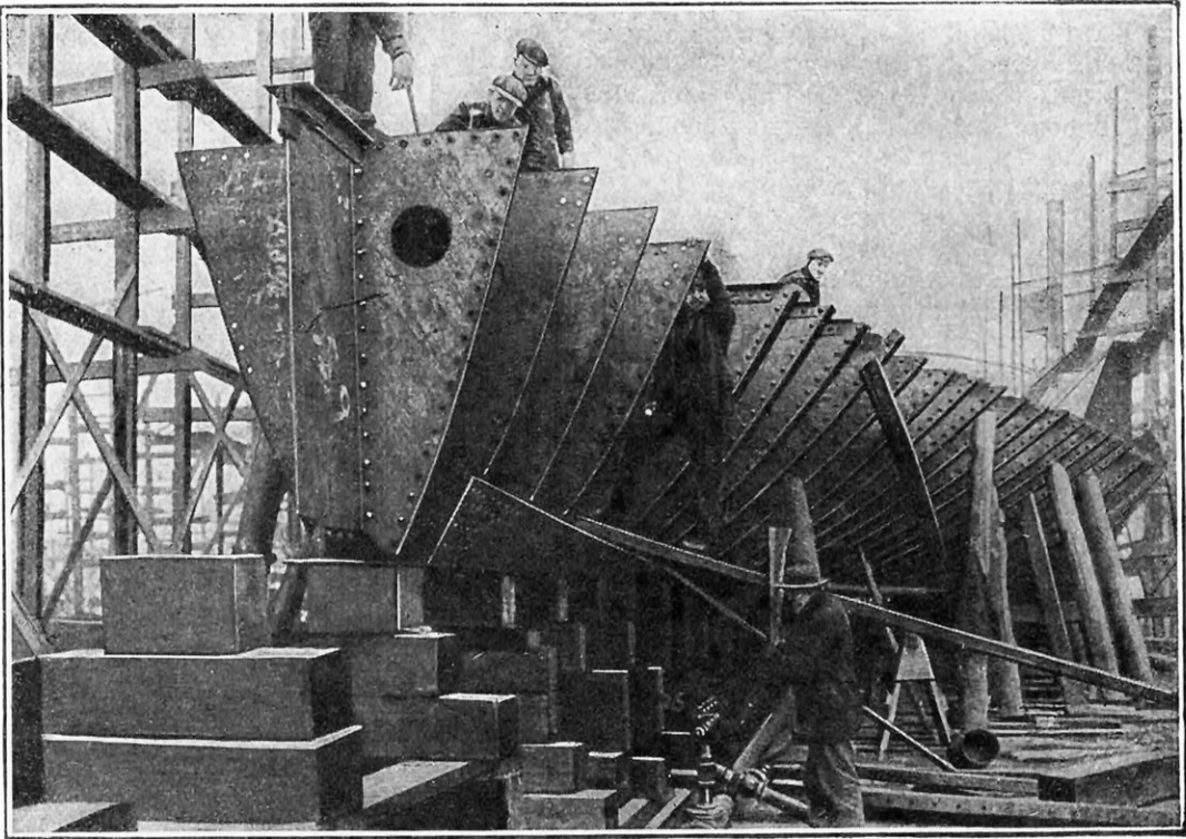
MONTAGE DE LA QUILLE ET AMORCES DES COUPLES DU NAVIRE « FABRIQUÉ »
