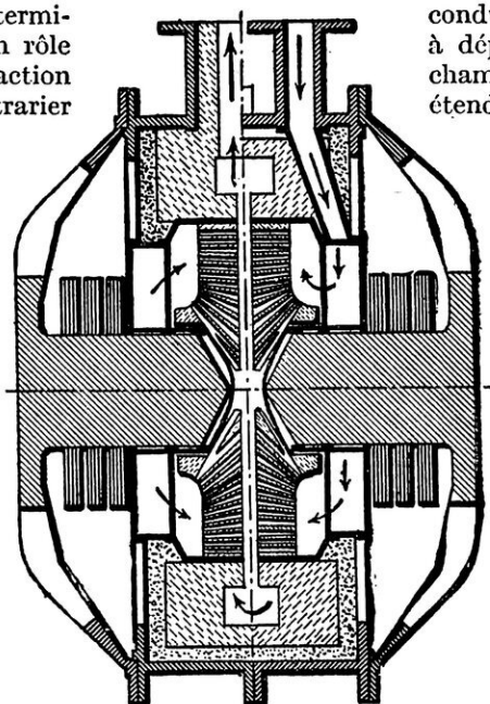
FIG. 9. — COUPE MONTRANT LA MARCHE DES GAZ DANS LE FOUR BIRKELAND-EYDE
