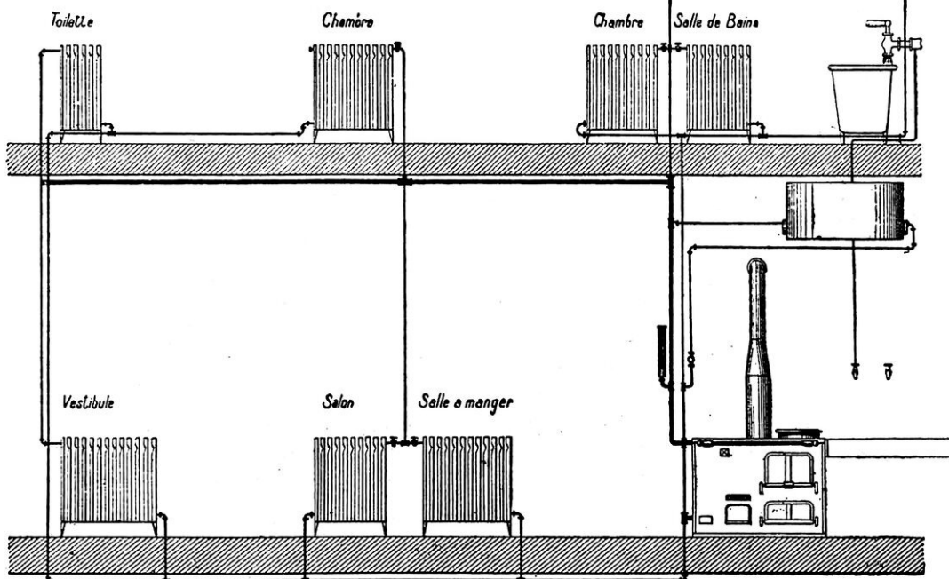
SCHEMA D'INSTALLATION DE CHAUFFAGE CENTRAL D'UNE VILLA, AVEC SERVICE D'EAU CHAUDE, PAR FOURNEAU DE CUISINE (SYSTEME D'AVÈNE ET ROBIN).
