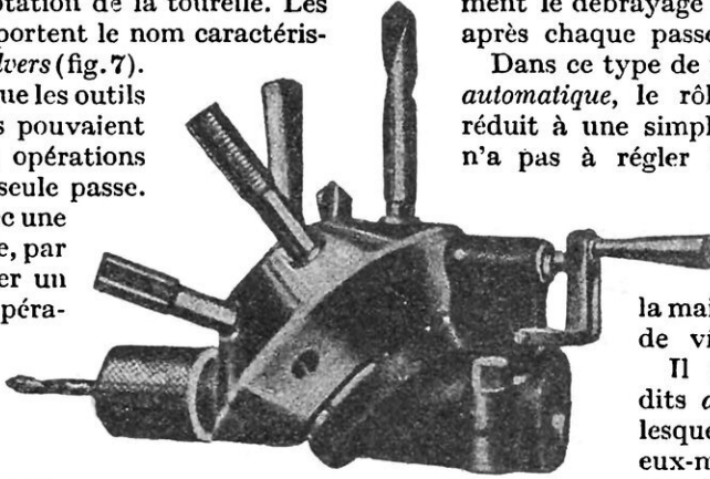
FIG. 8. — PORTE-OUTILS POUVANT ÊTRE MONTÉ SUR LA POUPEE D'UN TOUR ORDINAIRE
