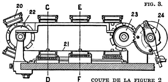
20, formes sur la courroie sans fin; 21, courroie sans fin; 22 et 23, tambours de la courroie; 24, rochet du tambour 23.
