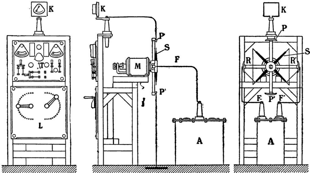
REDRESSEUR DE COURANT DE LA SOCIÉTÉ DE PURIFICATION DES GAZ (FACE, PROFIL, ARRIÈRE)
