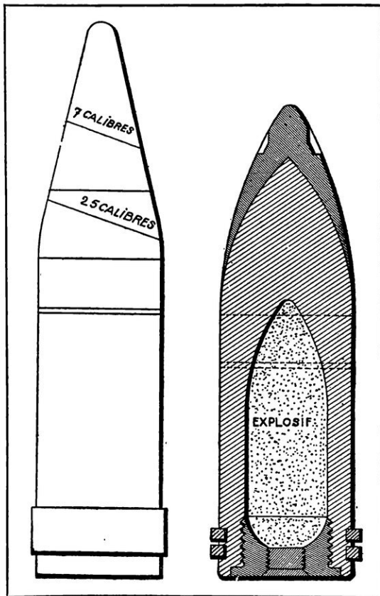
MODÈLES RÉCENTS D'OBUS AMÉRICAINS ET ANGLAIS, A CAPE
