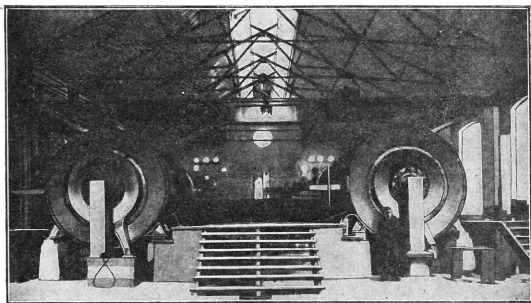
FIG. 10. — SALLE DES FOURS ÉLECTRIQUES DANS UNE USINE A ACIDE NITRIQUE
