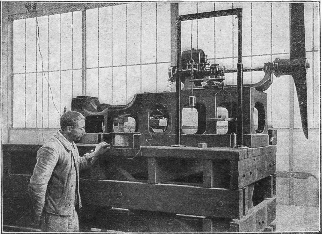
INSTALLATION POUR LES ESSAIS DE ROTATION DES HÉLICES AÉRIENNES
