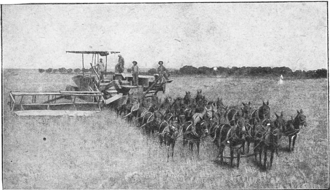
ATTELAGE DE 40 MULES REMORQUANT UNE GIGANTESQUE MOISSONNEUSE L'immense champ californien où cette machine puissante opère est moissonné en quelques heures.
