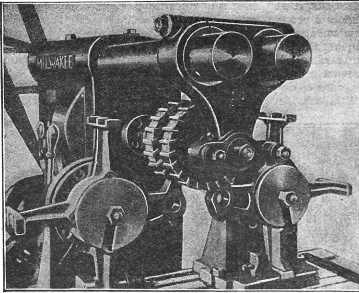
FIG. 12. — MACHINE A FRAISER PERFECTIONNÉE
