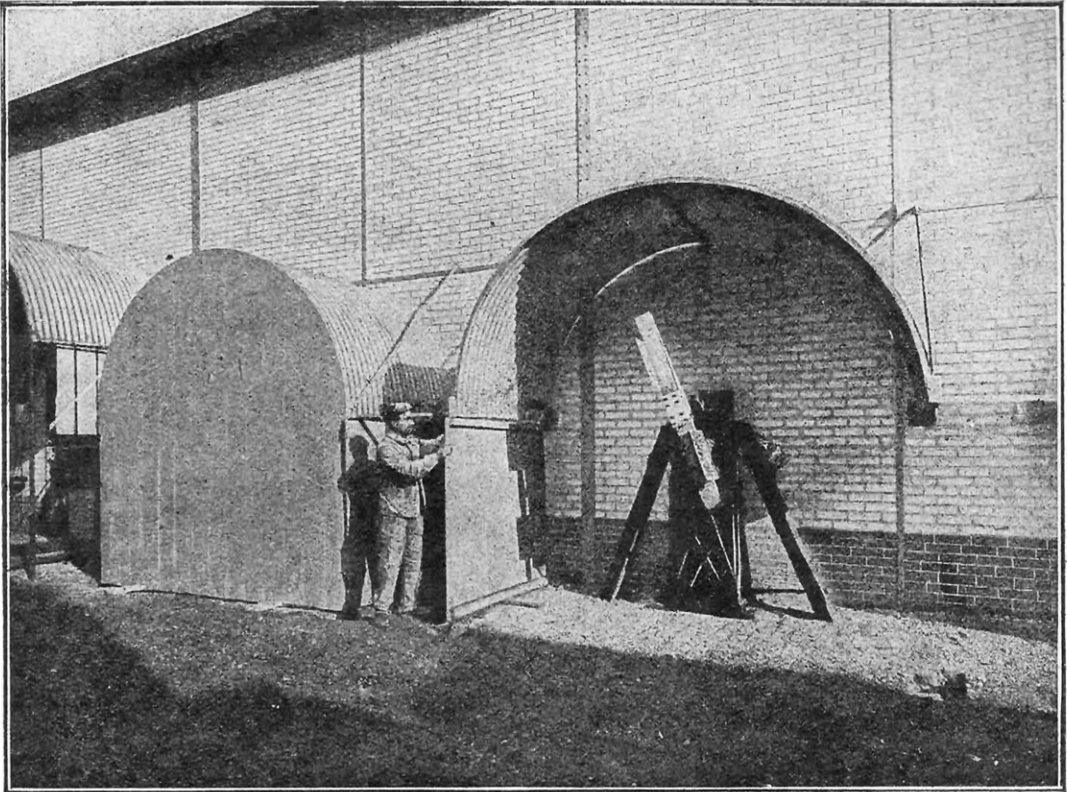
MOULINETS DYNAMOMÉTRIQUES IMAGINÉS PAR LE COLONEL RENARD
