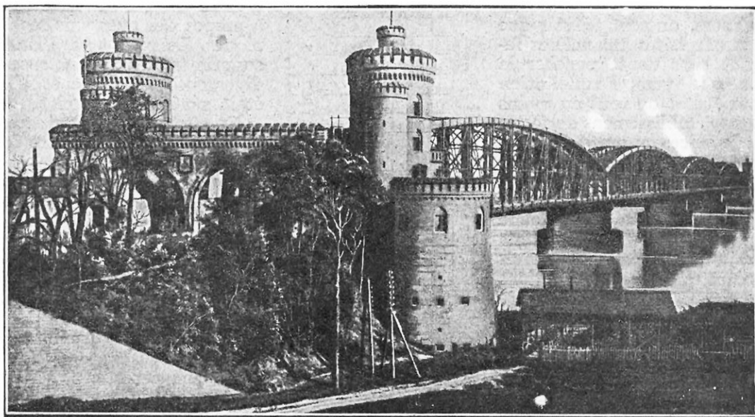
PONT MONUMENTAL DE CHEMIN SUR LE RHIN, A MAYENCE
