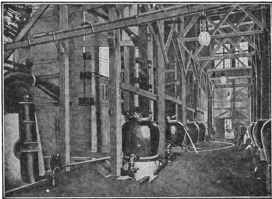
FIG. 11. — TOURS D'ABSORPTION DES OXYDES D'AZOTE (FABRIQUE D'ACIDE NITRIQUE)
