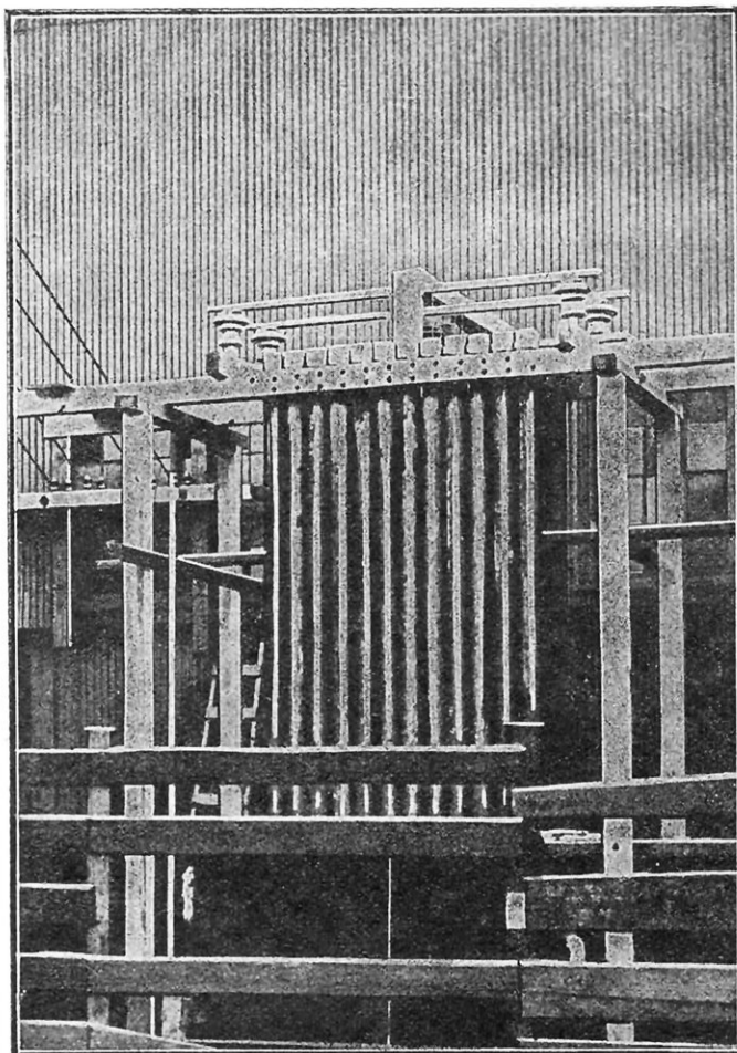
INSTALLATION D'ESSAI DANS UNE FONDERIE DE CUIVRE (CIRCUIT FERMÉ)
