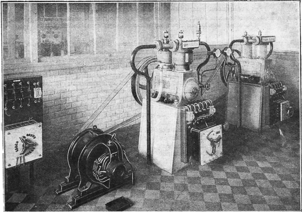
COMPRESSEUR ET POMPE A VIDE EN SERVICE DANS LES GRANDS LABORATOIRES
