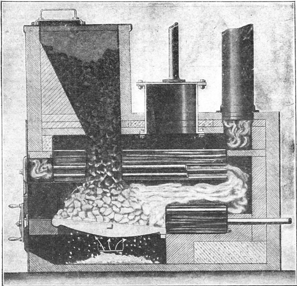
CHAUDIÈRE TUBULAIRE HORIZONTALE POUR LES GRANDES INSTALLATIONS DE CHAUFFAGE CENTRAL PAR LA VAPEUR
