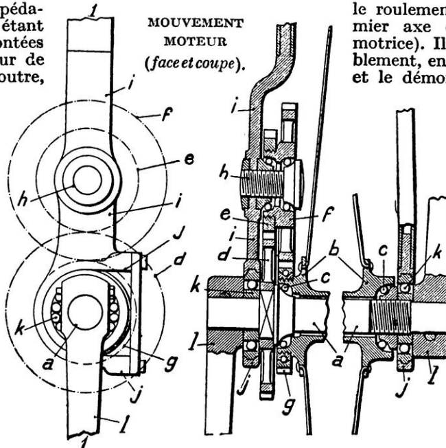
a, axe de la roue motrice; b, moyeu; c, roulement à billes; d, première roue d'engrenage; e, premier pignon; f, seconde roue d'engrenage; g, second pignon; h, second axe porté par le cadre; i, montant du cadre; j, étrier; k, roulement à billes sur l'axe a; l, l, manivelles auxquelles sont adaptées les pédales.
