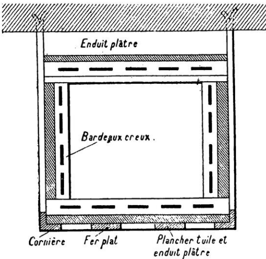
UN TYPE DE CONDUIT DE CHALEUR
