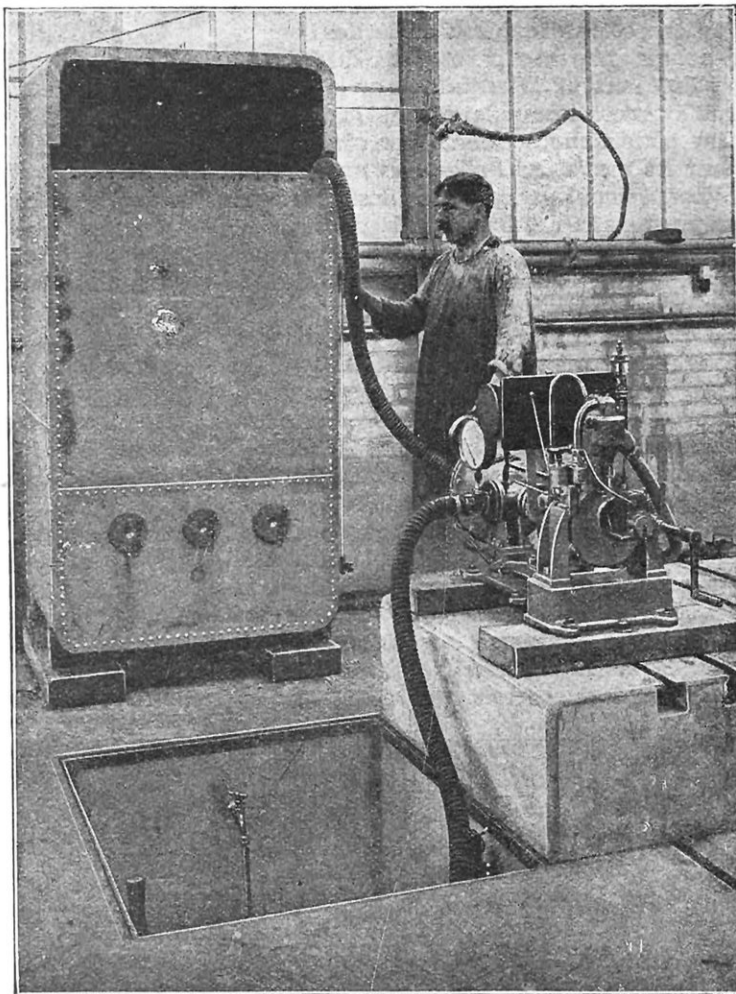
ESSAI D'UNE MOTO-POMPE SYSTÈME TONY-HUBER Le débit de la pompe s'évalue tout naturellement au moyen d'un récipient préalablement jaugé.
