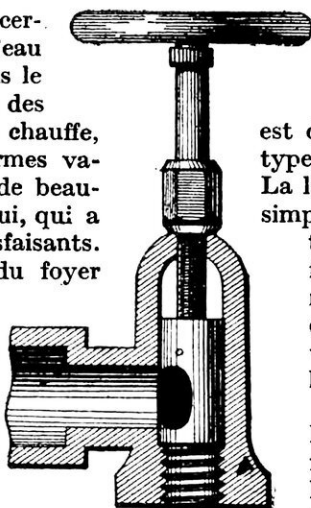
ROBINET AMÉRICAIN « QUART DE TOUR » A BOISSEAU CREUX.
