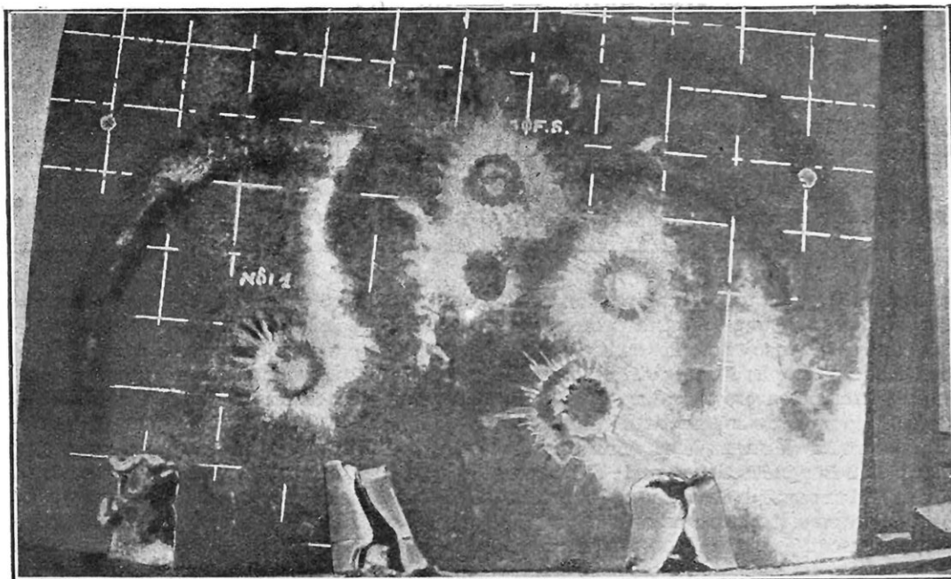
PLAQUE CÉMENTÉE « BETHLEHEM » POUR CUIRASSE DE CEINTURE (337 MM.)
