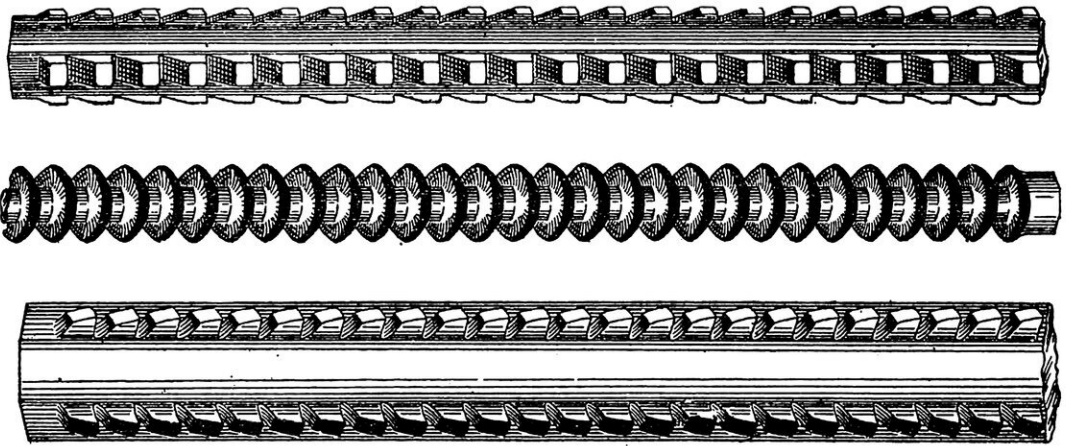
FIG. 17. — MANDRINS « LAPOINTE » EN ACIER SPÉCIAL CONSTITUÉS PAR UNE SÉRIE DE DISQUES A DENTS A SECTION LÉGÈREMENT CROISSANTE, FOURNISSANT UN TRAVAIL RAPIDE Ces dents présentent les angles de coupe nécessaires à l'usinage, et leur profil correspond exactement à celui de la pièce à obtenir. Cet outillage est promptement amorti et permet une grande précision.
