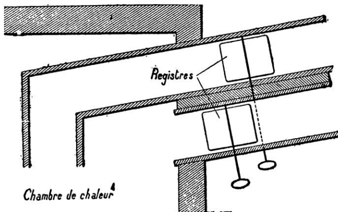
CONDUITS D'AIR CHAUD SUPERPOSÉS AU DÉPART DE LA CHAMBRE DE CHALEUR ET INCLINÉS POUR DIMINUER LES PERTES DE CHARGE
