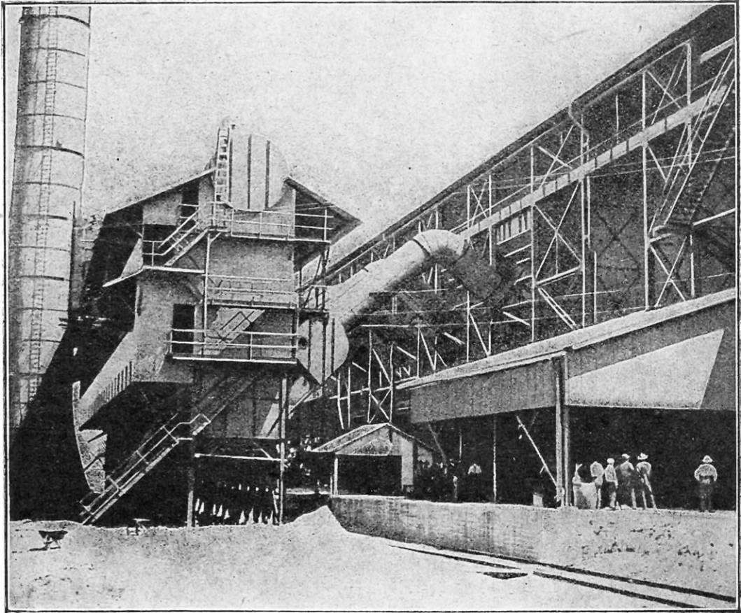
ENSEMBLE D'UNE INSTALLATION MODERNE DE PRÉCIPITATION ÉLECTRIQUE
