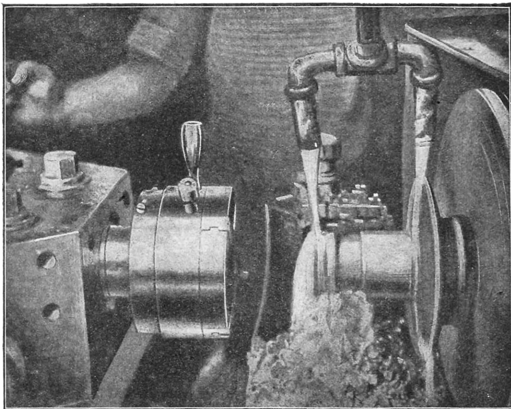
FIG. 2 — LE RENDEMENT DES OUTILS, MÊME LORSQU'ILS SONT ÉTABLIS EN ACIER EXTRA-RAPIDE, EST NOTAMMENT AUGMENTÉ PAR UN JET D'EAU SAVONNEUSE ININTERROMPU, ALIMENTÉ PAR UNE PETITE POMPE A ENGRENAGE
