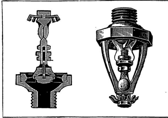
EXTINCTEUR AUTOMATIQUE SYSTÈME ADAM A droite : tête entièrement montée, prête à fonctionner, représentée en demi-grandeur ; à gauche : coupe avec l'arcade enlevée.
