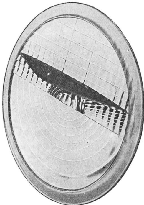
FACE DE LA LENTILLE TOURNÉE VERS LA LAMPE A INCANDESCENCE DU PHARE On remarquera tout particulièrement la forme et la position de l'abat-jour.
