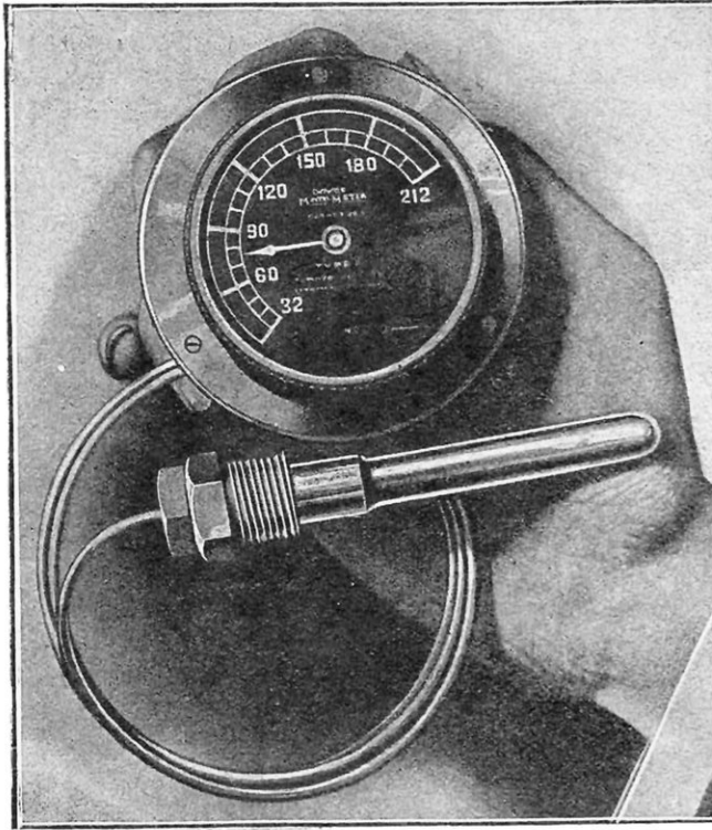
VUE EXTÉRIEURE DU THERMOMÉTROGRAPHE DONT SONT MUNIS LA PLUPART DES AVIONS AMÉRICAINS
