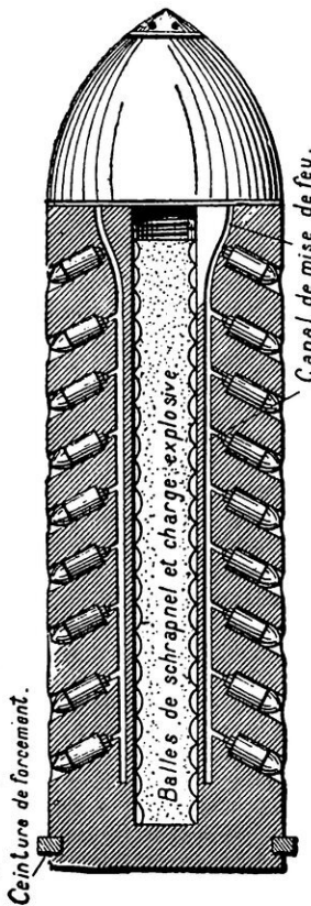
FIG. 1. — PROJECTILE LANÇANT DES PETITS OBUS VERS L'ARRIÈRE. (Voir la figure de la page suivante).
