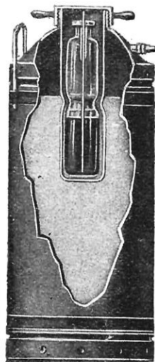
VUE INTÉRIEURE DE L' « AUTOMATIC » On distingue la bouteille en verre contenant l'acide réactif et se débouchant d'elle-même au moment du retournement de l'appareil.
