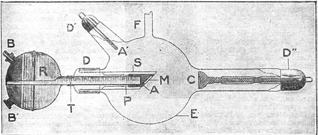
SCHÉMA D'UN TUBE A RAYONS X, INTENSIF, A REFROIDISSEMENT PAR EAU
