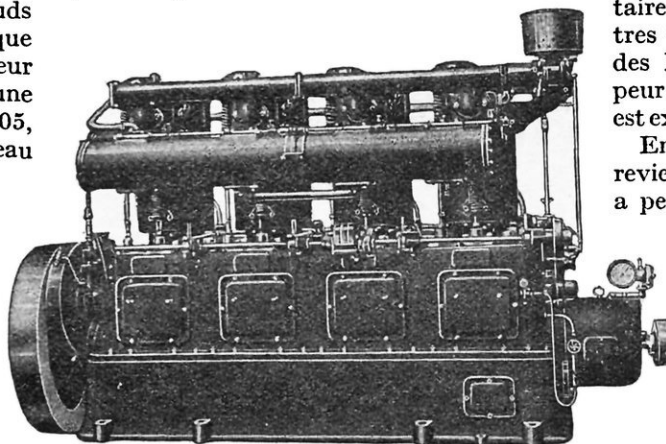
MOTEUR « GARDNER », TYPE VERTICAL, FONCTIONNANT AU GAZ DE VILLE OU AU GAZ PAUVRE
