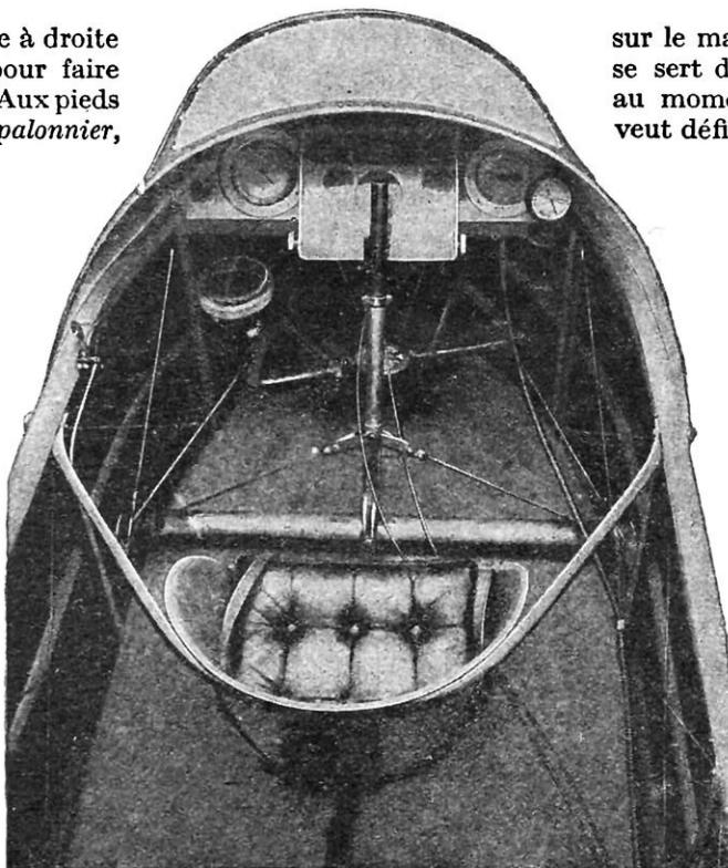
LES ORGANES DE COMMANDE SUR UN AVION DE 1914 Devant le siège du pilote est placé le «manche à balai». Au fond, près du plancher de la carlingue, on voit le palonnier; face à celui-ci est disposée la boussole à cardan; au-dessus, le déroule-carte; à droite, le compte-tours; à gauche, l'altimètre.
