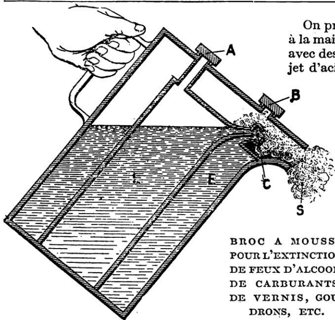
BROC A MOUSSE POUR L'EXTINCTION DE FEUX D'ALCOOL, DE CARBURANTS, DE VERNIS, GOUDRONS, ETC. A et B, trous de remplissage des deux récipients intérieur et extérieur ; E, liquide alcalin et savonneux du récipient extérieur ; L, acide ou eau fortement acidulée ; C, orifices de sortie des deux liquides et chambre où s'opère leur mélange fournissant la mousse ; S, mousse extinctrice projetée sur le foyer de l'incendie.
