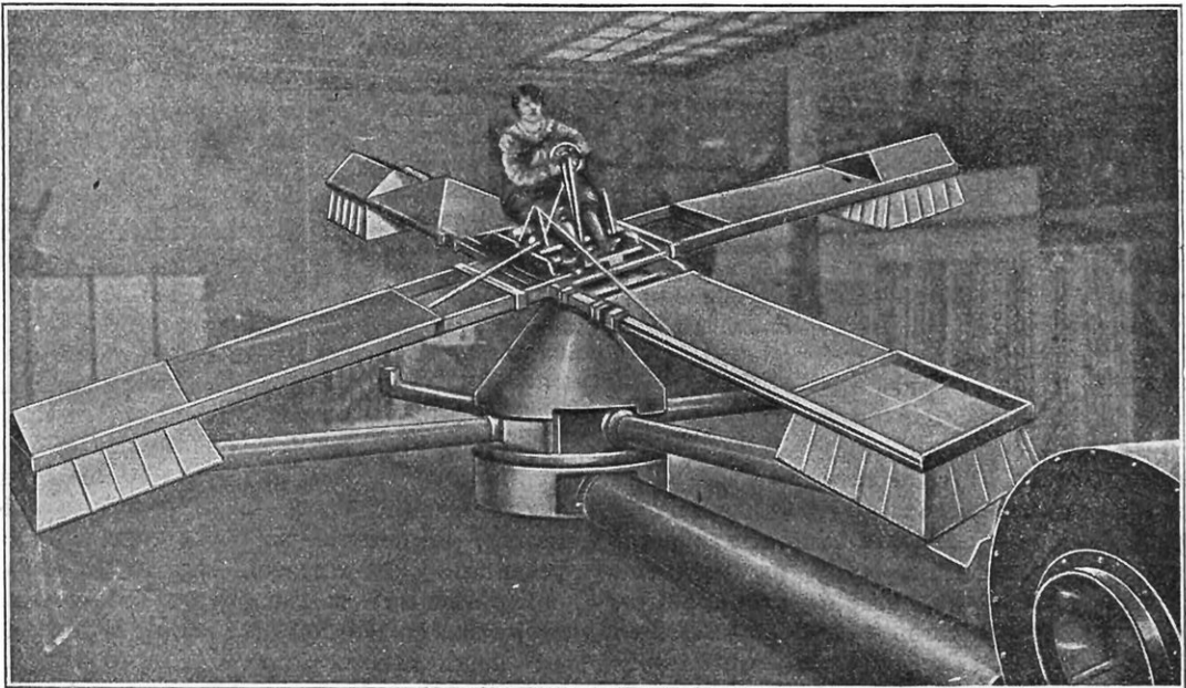
LA MACHINE AMÉRICAINE POUR APPRENDRE AUX FUTURS PILOTES LES ÉLÉMENTS DU VOL
