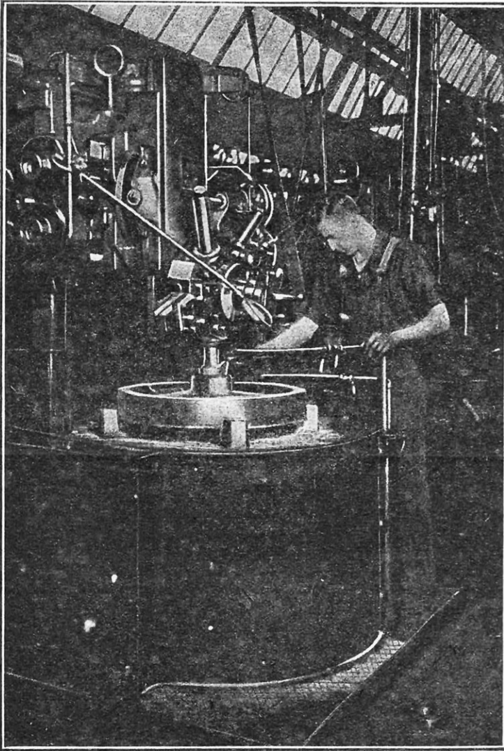
FIG. 10. — TYPE DE TOUR VERTICAL A TOURELLE
