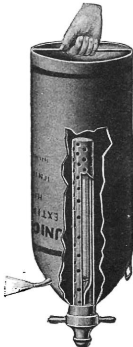
EXTINCTEUR « UNIC » Position de fonctionnement.
