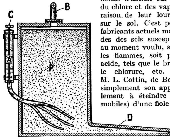
COUPE D'UN EXTINCTEUR A POUDRE
