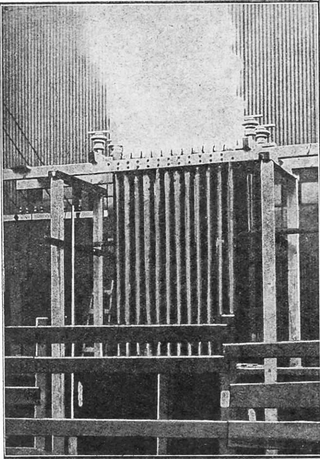
INSTALLATION D'ESSAI DANS UNE FONDERIE DE CUIVRE (CIRCUIT OUVERT)
