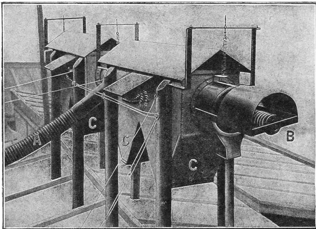
APPAREIL POUR LA CAPTATION DES POUSSIÈRES DE CIMENT
