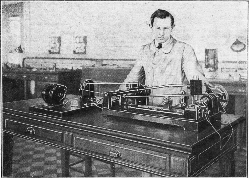
LA CURIEUSE MACHINE A CHOCS RÉPÉTÉS DE CAMBRIDGE
