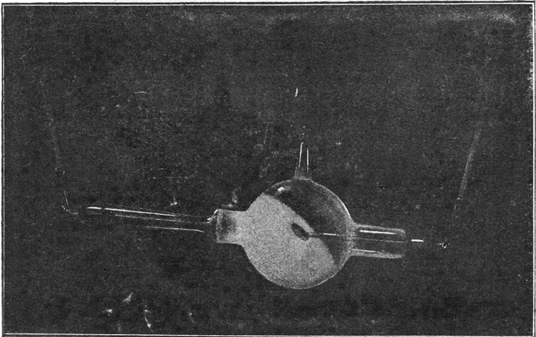
TUBE A OSMO RÉGULATEUR VILLARD, POUR LA RADIOTHÉRAPIE
