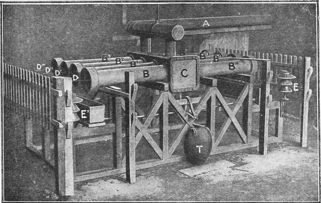
APPAREIL POUR LA CAPTATION DES PARTICULES D'ACIDE SULFURIQUE
