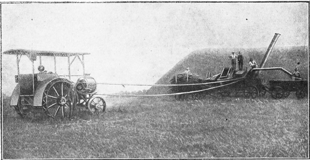
MACHINE A BATTRE « NOUVEAU SIÈCLE », ACTIONNÉE PAR UN MOTEUR A PÉTROLE Le long tube dressé obliquement sert à chasser, par le ventilateur, la paille qui forme automatiquement une meule plus ou moins longue, suivant le déplacement de la batteuse.
