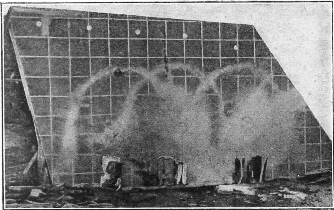
PLAQUE DE CUIRASSE « BETHLEHEM » (250 MM.) APRÈS ATTAQUE D'UN PROJECTILE DE 305
