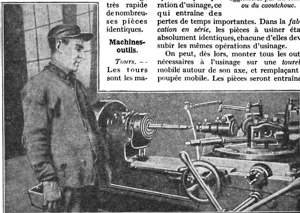
FIG. 7. — SÉRIE D'OUTILS MONTÉS SUR UNE TOURELLE ROTATIVE Grâce à leur disposition, ces outils peuvent travailler successivement et rapidement chaque pièce.
