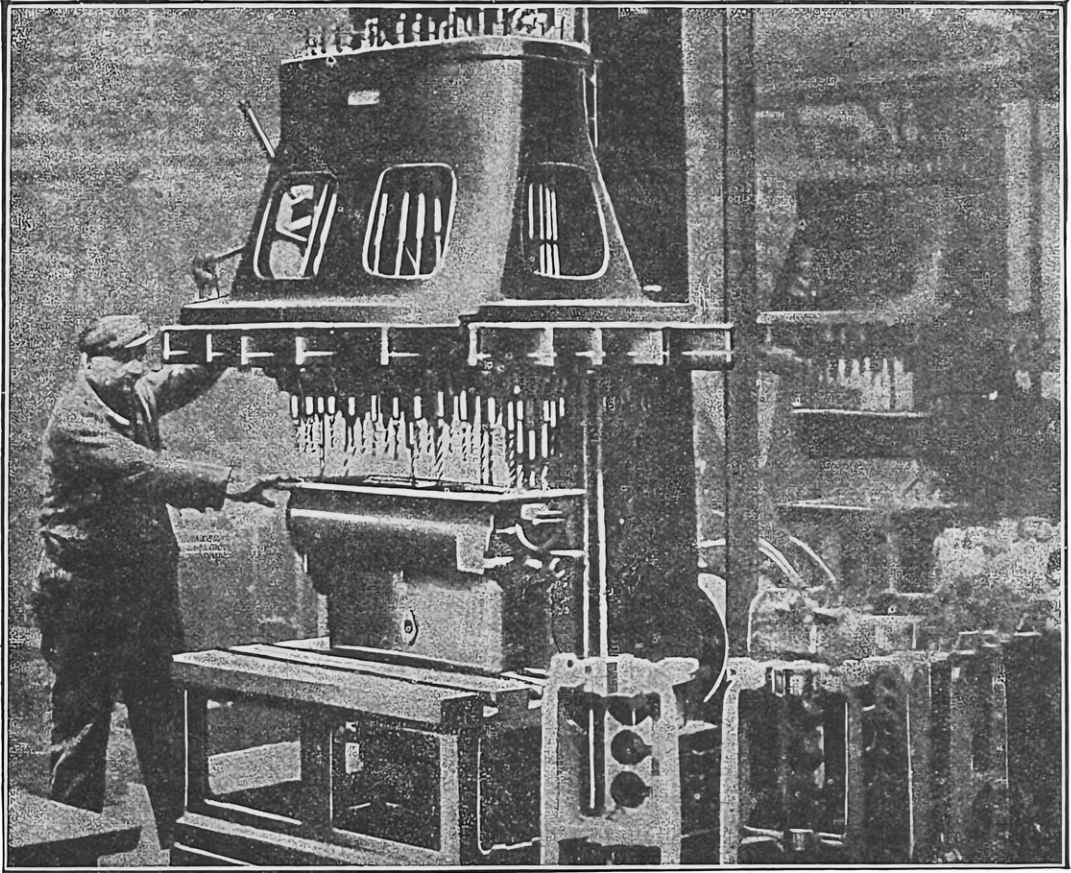
FIG. 11. — MACHINE EFFECTUANT DES PERCEMENTS MULTIPLES
