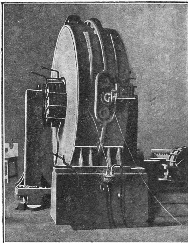
FIG. 8. — FOUR BIRKELAND-EYDE A OXYDES D'AZOTE
