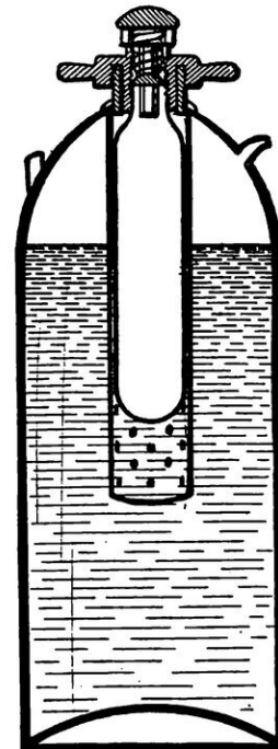
« UNIC » POUR AUTOS Coupe verticale.
