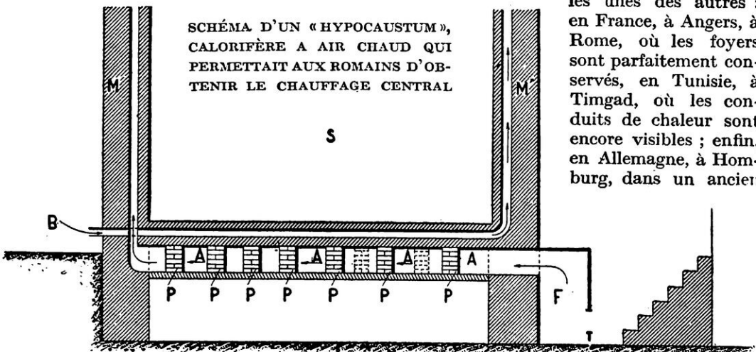
S, salle à chauffer ; F, foyer ; A, passage de la fumée chauffant le mur M ; P P, pieds-droits en maçonnerie de briques ; B, prise d'air ; le mur M' est chauffé intérieurement par un conduit d'air chaud.
