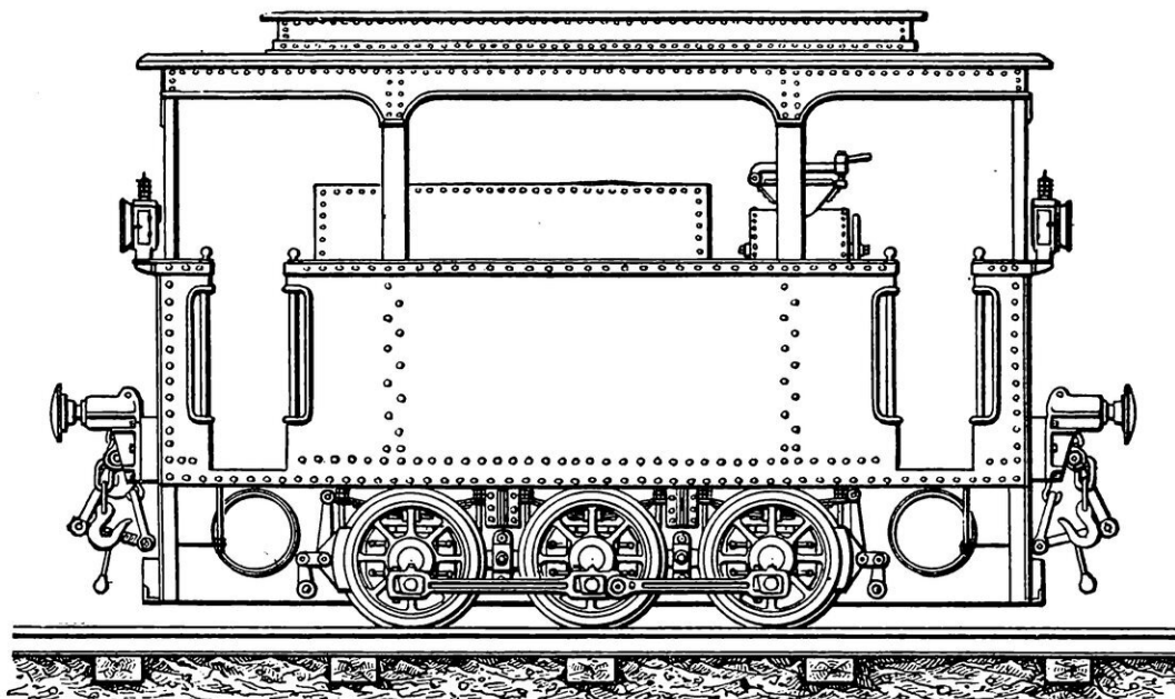
TYPE DE LOCOMOTIVE A GAZ PAUVRE (GAZOGÈNE AU BOIS) POUR VOIES FERRÉES
