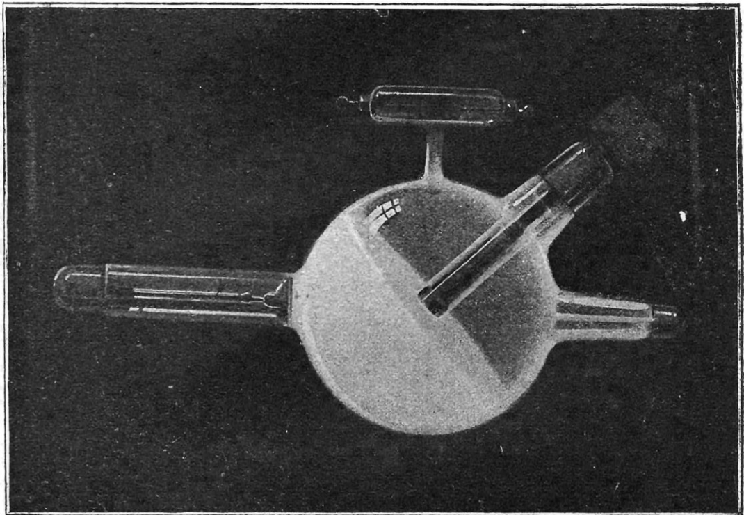
TUBE RADIOLOGIQUE A REFROIDISSEMENT AU MOYEN D'UNE CIRCULATION D'AIR
