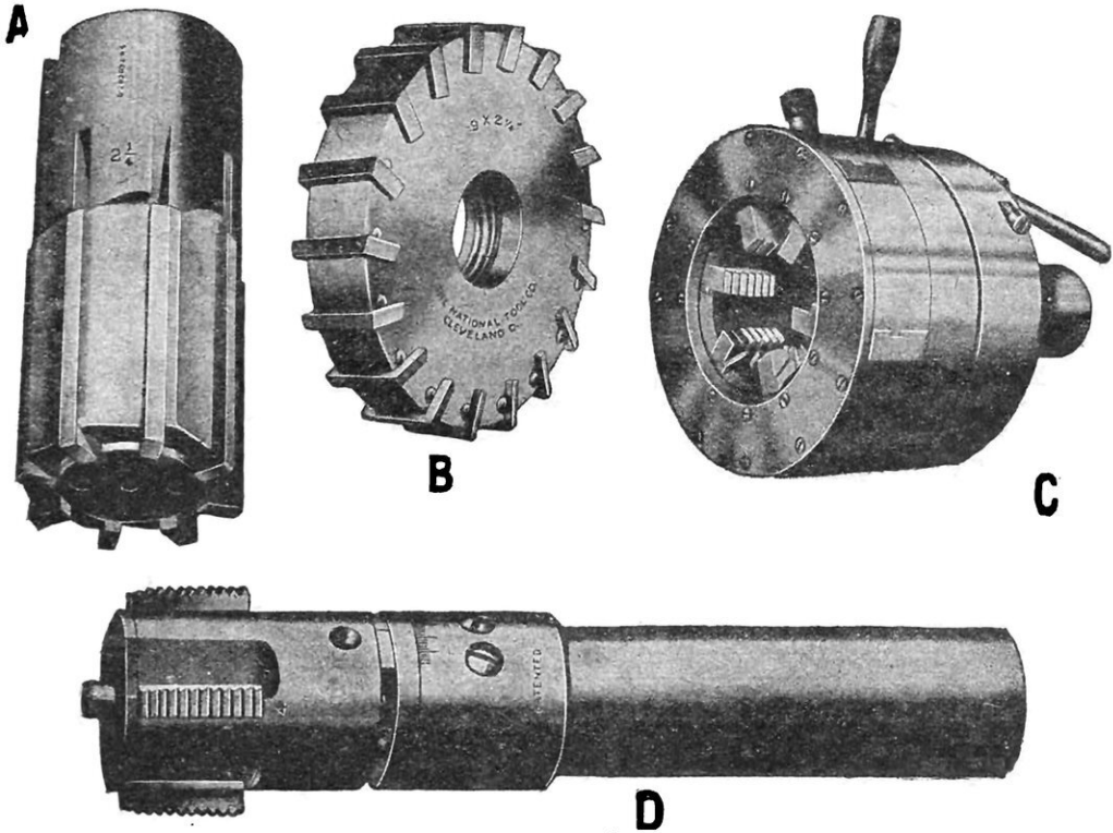
FIG. 5. — QUELQUES AUTRES TYPES D'OUTILS A LAMES RAPPORTÉES
