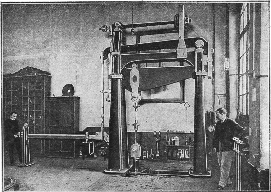
MACHINE SPÉCIALE POUR L'ESSAI DES MÉTAUX A LA TRACTION
