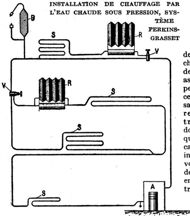
A, générateur ; B, vase d'expansion fermé ; S, surfaces de chauffe diverses dans le local ou l'appartement ; R, radiateurs à bouteille ; V, robinets-vannes.
