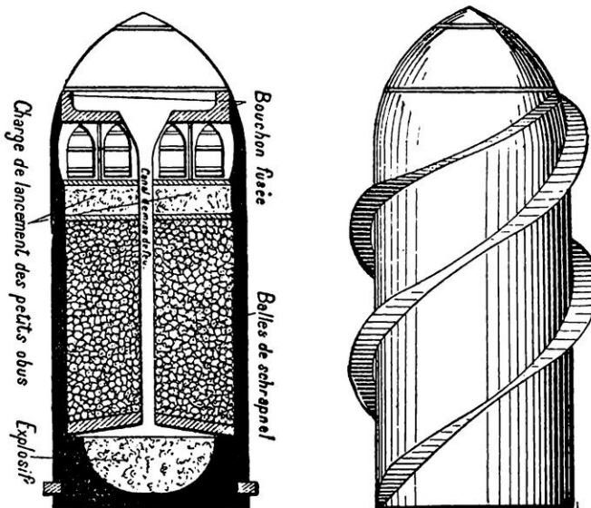
FIG. 3. — AUTRE PROJECTILE « MÈRE-GIGOGNE » POUR TIRER SUR DES BATTERIES MASQUÉES
