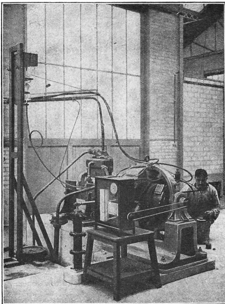
DYNAMO-DYNAMOMÈTRE SYSTÈME PANHARD-LEVASSOR
