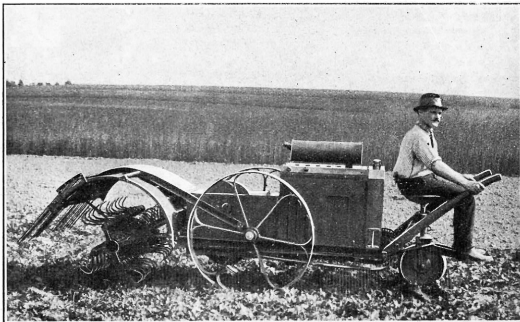
LE MOTOCULTEUR TYPE « VIGNERON » OU « MARAICHER »
