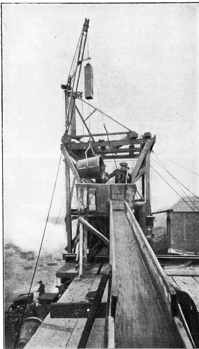
LA COULÉE DU BÉTON ENTRE DEUX PAROIS DE FONTE
