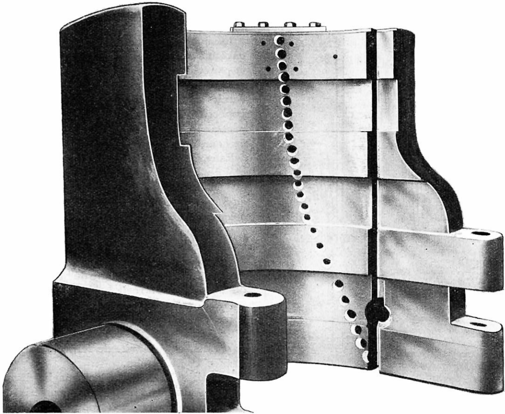
MANCHON A TOURILLONS D UN CANON DE 305 MILLIMÈTRES ROMPU, PRÉPARE POUR ÊTRE SOUDÉ Des trous ont été percés tout le long de la fissure afin de permettre au fer thermit de pénétrer dans la pièce brisée sous une épaisseur suffisante pour constituer une soudure homogène et solide.
