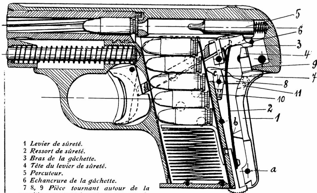
FIG 5. — LE PERCUTEUR A L'ARMÉ ET BLOQUÉ PAR LE MÉCANISME DE SURETÉ
