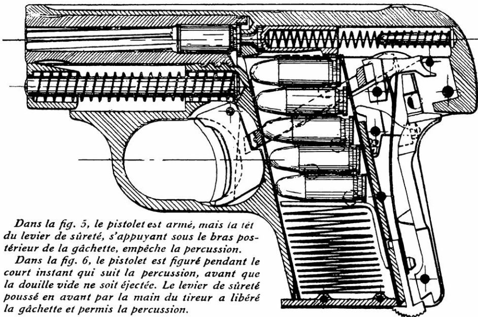
FIG. 6.— LE MÉCANISME DE SURETÉ DANS LA POSITION DU TIR ET LE PERCUTEUR A L'ABATTU
