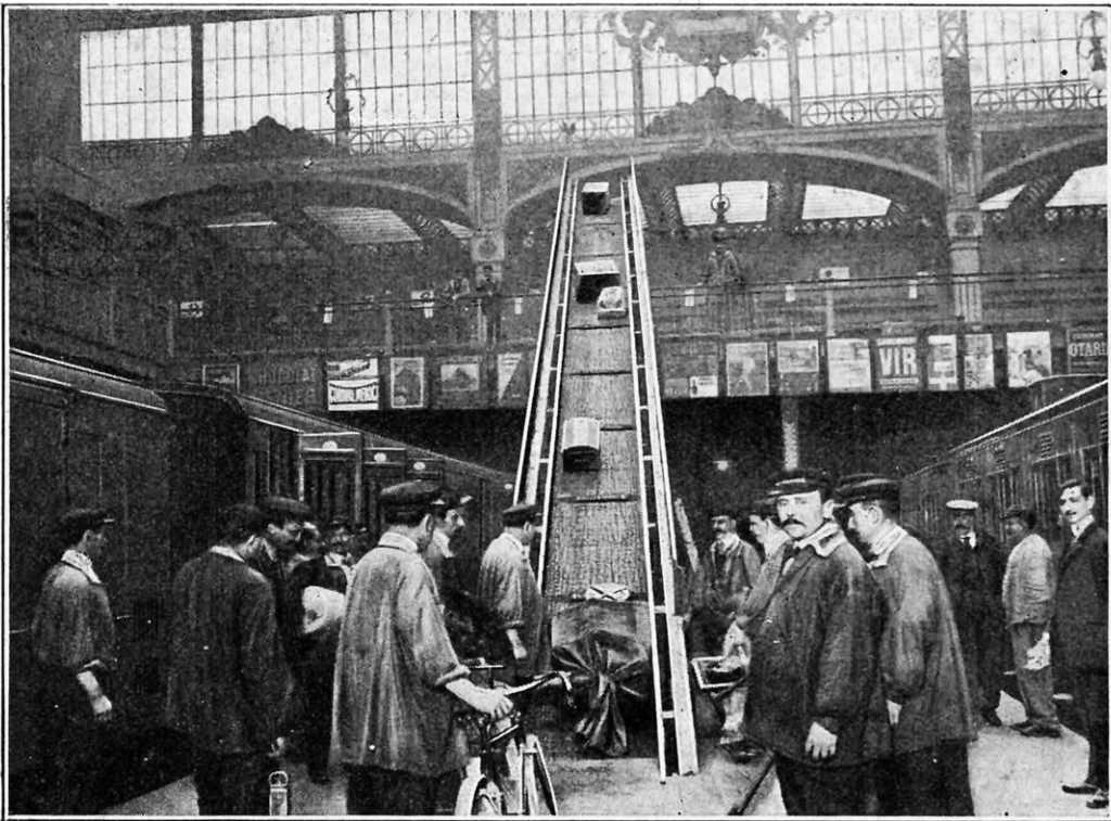
Une des toiles mobiles vue de face. Les bagages arrivent de la toile sur une partie souterraine invisible sur la figure. On les voit ici reparaitre et se diriger vers les salles du rez-de-chaussée.
