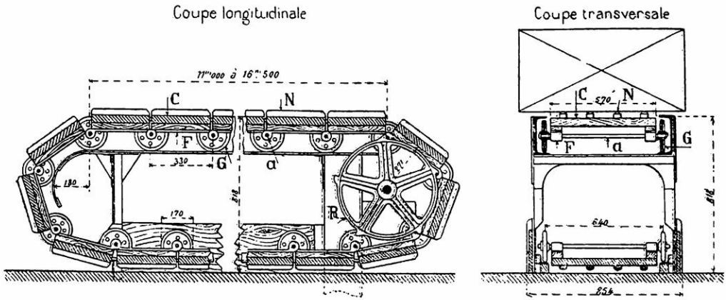
Coupe longitudinale et transversale d'un banc mobile. L'appareil est constitué par une chaîne de chariots C roulant sur des galets G. Chaque chariot est articulé au suivant par l'essieu a des galets communs. R roue motrice; F longeron; a essieu; G galet; N demi-fer rond.
