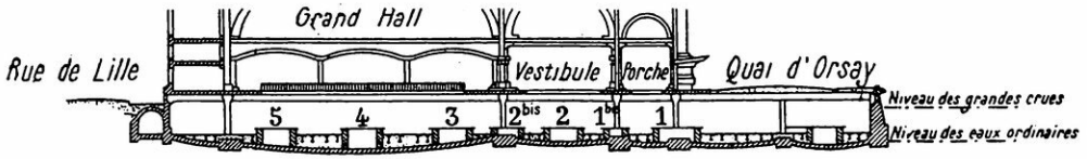
Coupe transversale suivant AB (Fig. 1)
