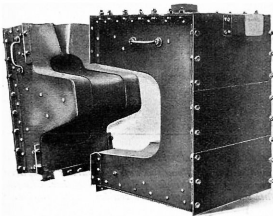
MOULE POUR LA RÉPARATION D'UNE PIÈCE EN U
