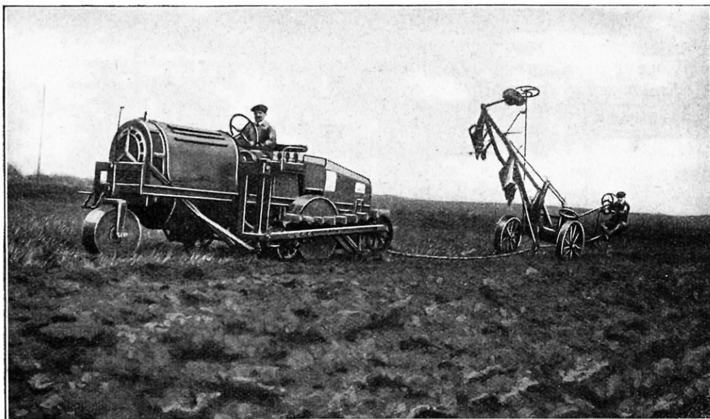
TRACTEUR AUTOMOBILE LEFEBVRE REMORQUANT UNE CHARRUE A BASCULE
