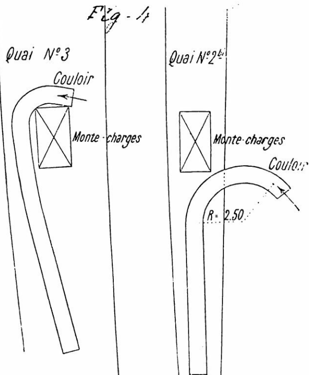
SCHÉMA MONTRANT LES FORMES VARIÉES DE COULOIRS
