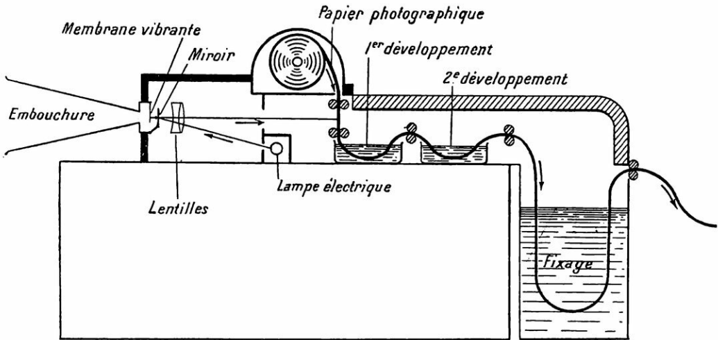
COUPE SCHÉMATIQUE DE L'APPAREIL QU'EMPLOIE M MARAGE POUR PHOTOGRAPHER LA VOIX
