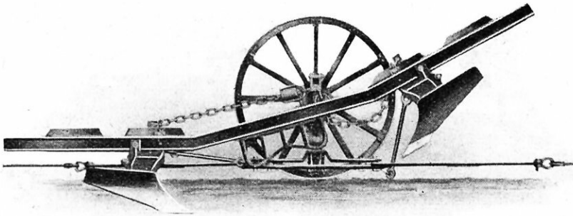
CHARRUE A BASCULE UTILISÉE DANS LE LABOURAGE A CABLE
