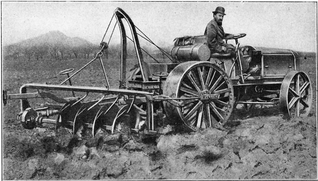
CHARRUE AUTOMOBILE A DISQUES SYSTÈME GILBERT
