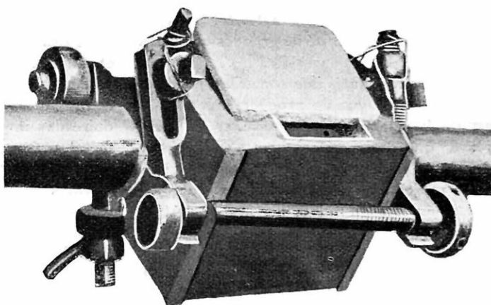
MOULE EN TÔLE POUR TUYAUX DE GRANDS DIAMÈTRES
