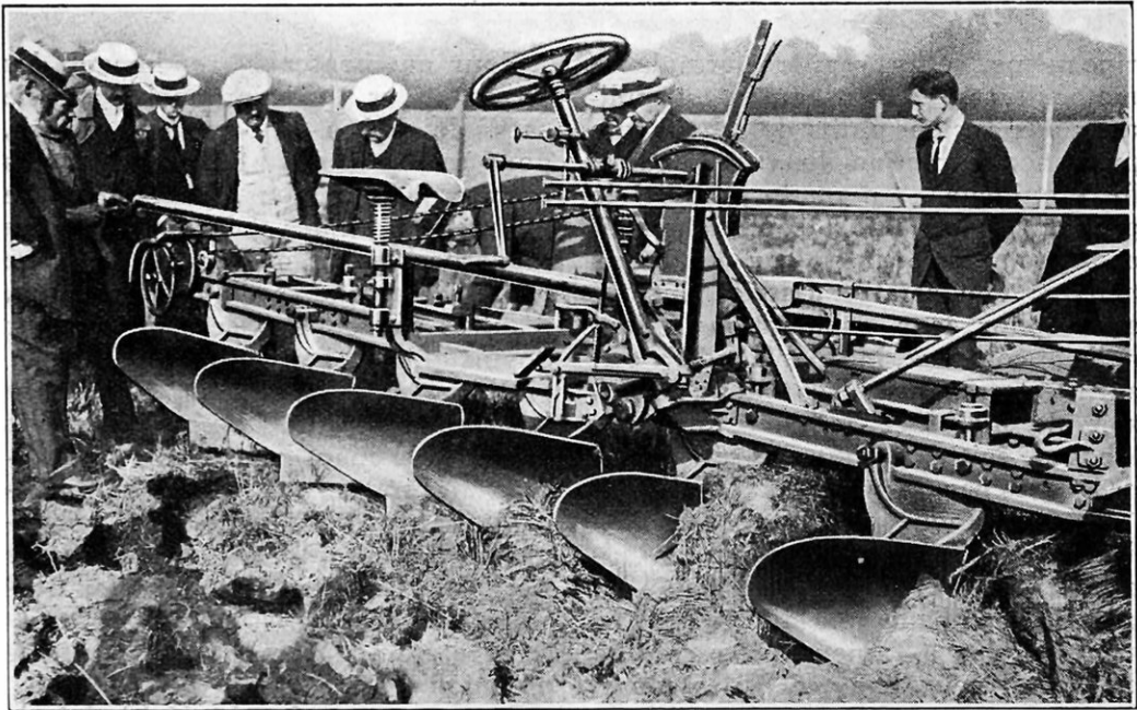
VUE DES SOCS ET DES COMMANDES D'UNE MOTOCHARRUE
