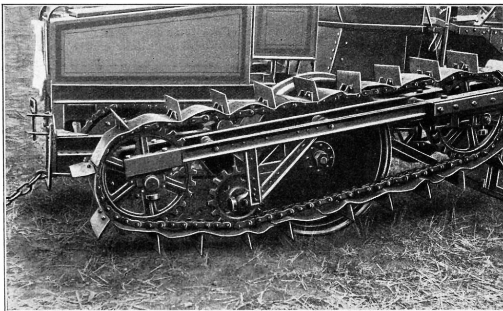
DÉTAILS DE LA CHAÎNE MOTRICE DU TRACTEUR LEFEBVRE
