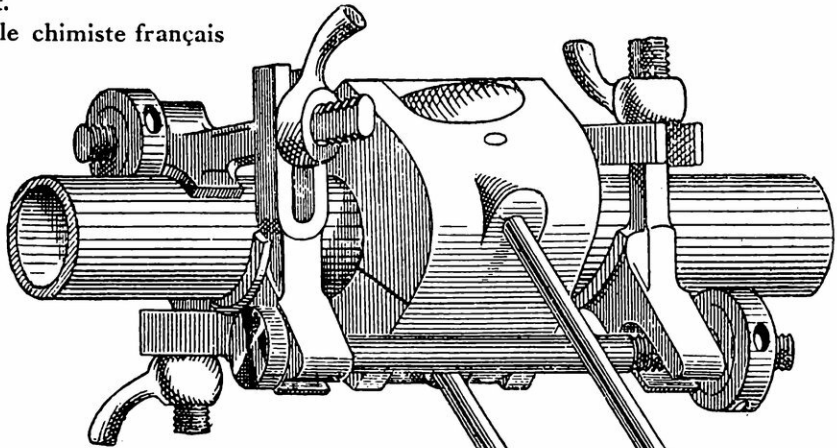
MOULE EN DEUX PARTIES POUR TUYAUX
