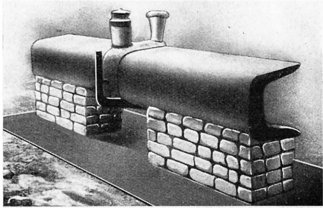
PIÈCE EN U SOUDÉE PAR LE PROCÉDÉ ALUMINOTHERMIQUE
