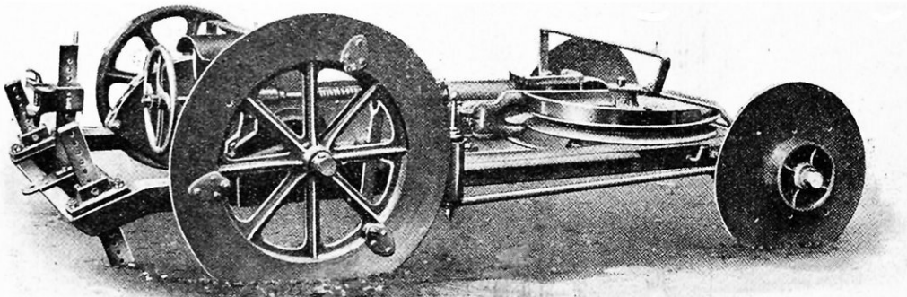
ANCRE AUTOMATIQUE POUR LE LABOURAGE A CABLE AVEC LOCOMOBILE UNIQUE
