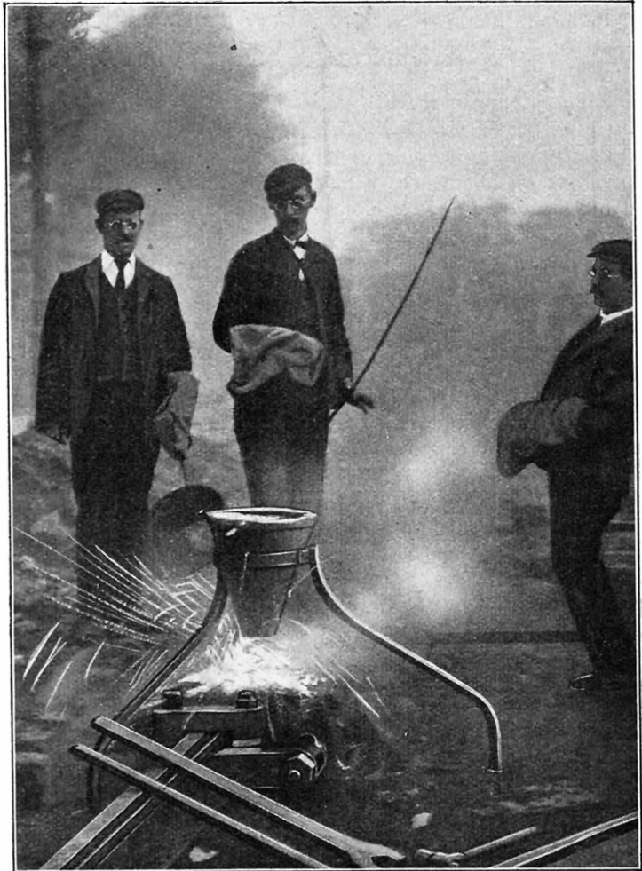
SOUDAGE DE RAILS DE TRAMWAYS
