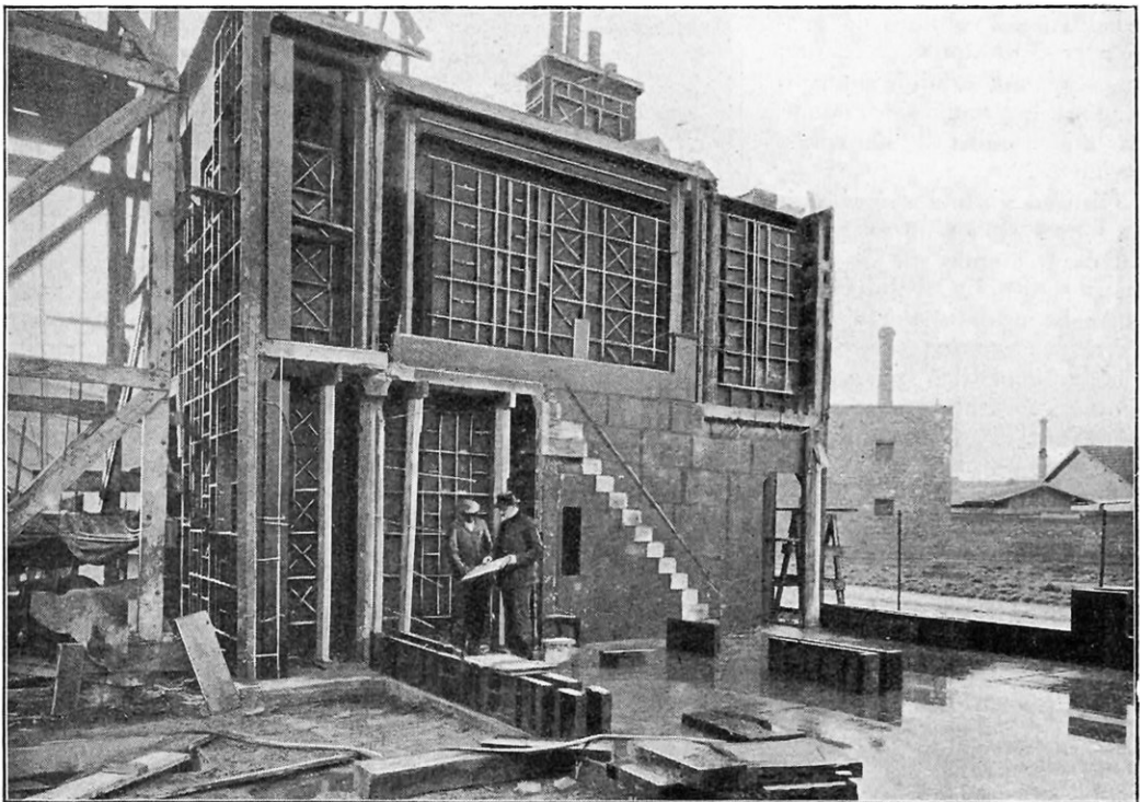
VUE D'UNE DES FACES INTERNES PENDANT L'ASSEMBLAGE DES PLAQUES DU MOULE
