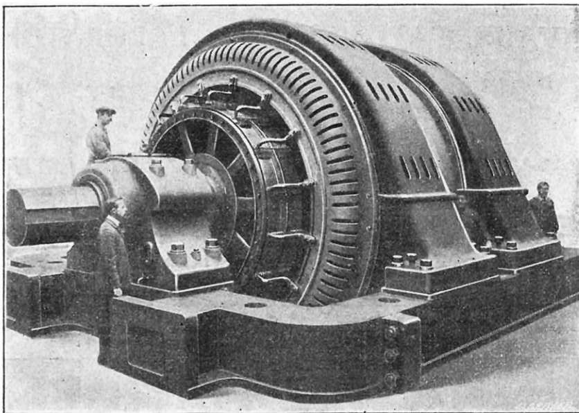
Moteur réversible de laminoir. Puissance : 16.000 chevaux à 60 tours. Installé à la Société de la Providence, à Rehon.
