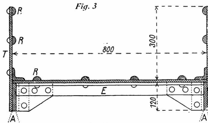
COUPE TRANSVERSALE D'UN COULOIR DE DESCENTE
