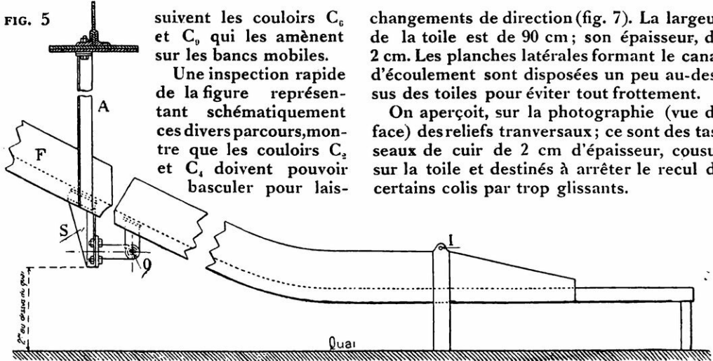
Schéma montrant l'articulation des grands couloirs mobiles, qui permet, lorsque ces couloirs restent inutilisés, de les relever afin de laisser plus d'espace libre sur le quai.
