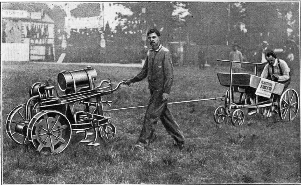
BINEUSE AUTOMOBILE REMORQUANT UN PLANTEUR DE POMMES DE TERRE
