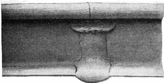
JOINT GOLDSCHMIDT SOUDÉ POUR RAILS
