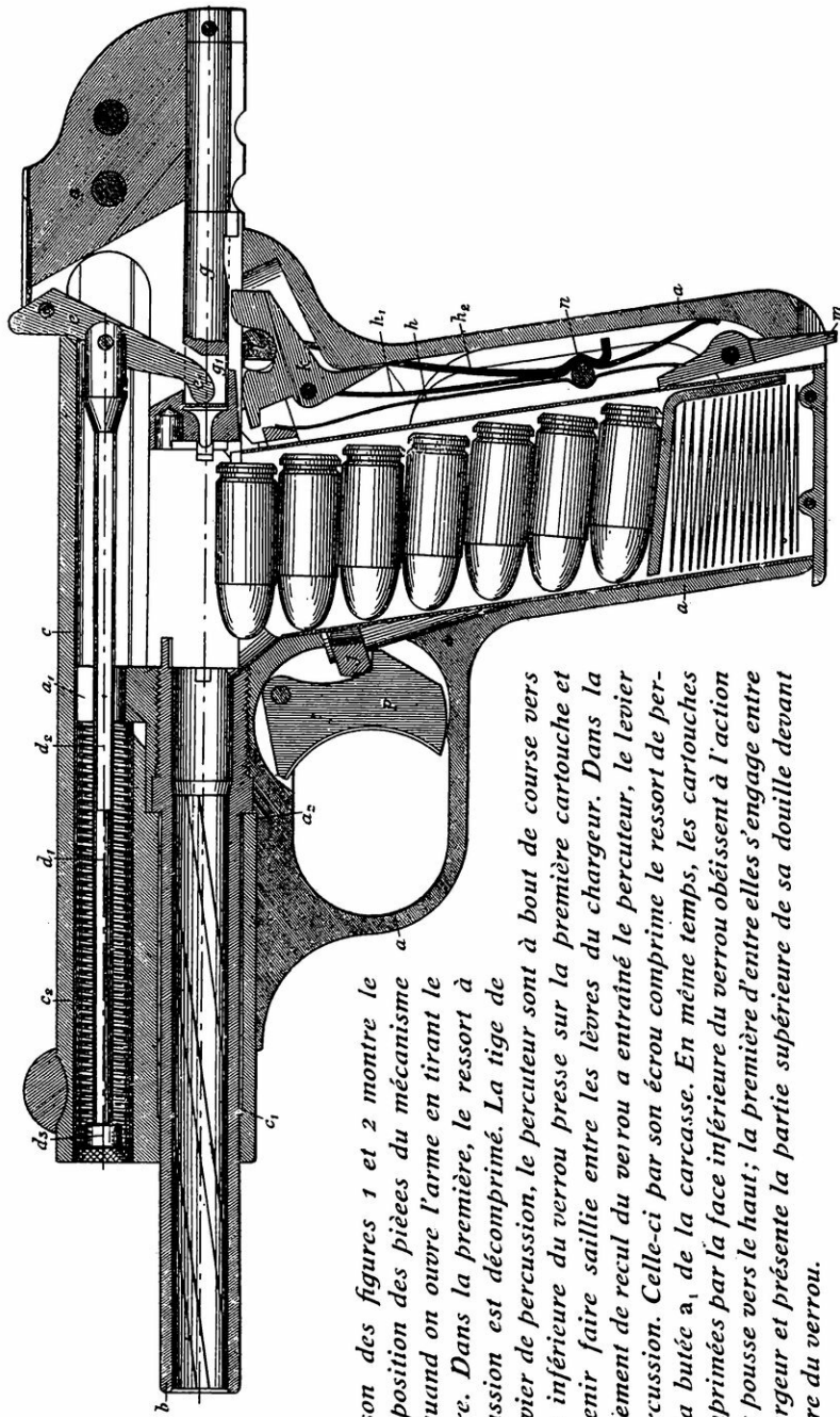
Fig. 2 — Coupe du pistolet Browning calibre 7,65. Position du chargement
