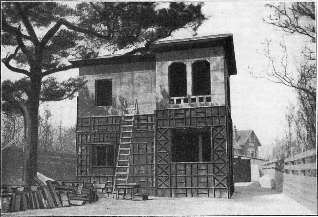
LE DÉMOULAGE DE LA MAISON COULÉE EN BÉTON, ÉDIFIÉE A SANTPOORT (HOLLANDE)
