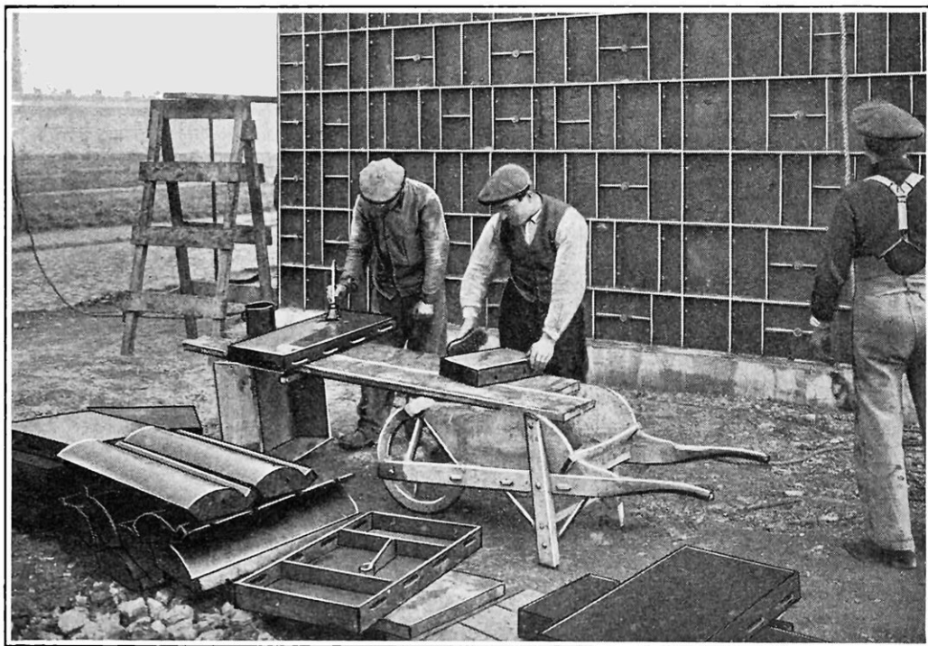
NETTOYAGE ET APPRÊT DES PLAQUES CONSTITUANT LE MOULE
