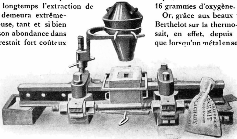
DISPOSITIF POUR LE SOUDAGE DE DEUX RAILS BOUT A BOUT DANS TOUTE LEUR SECTION
