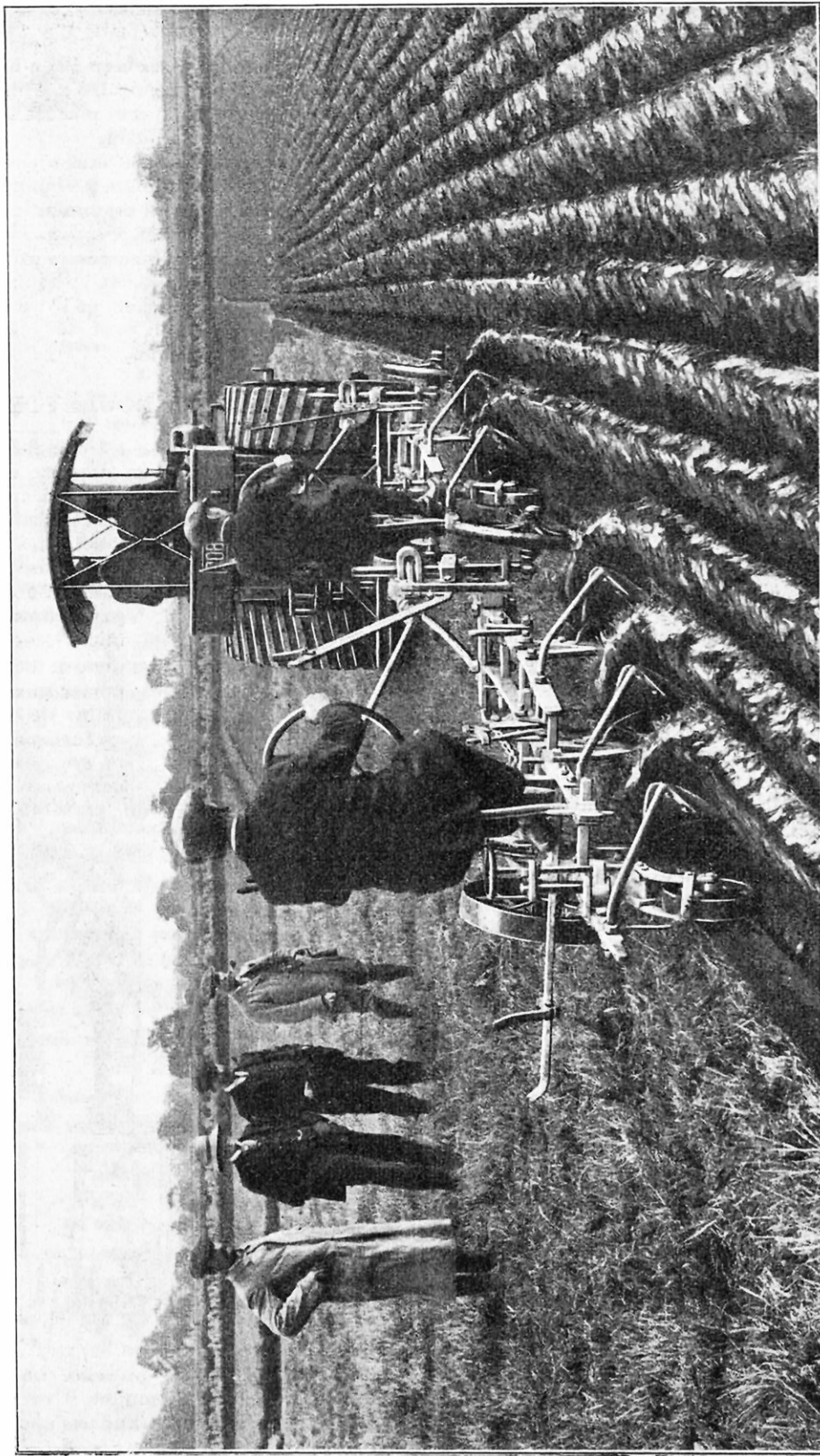
TRAIN DE DEUX CHARRUES A VERSOIRS REMORQUÉ PAR UN TRACTEUR A VAPEUR
