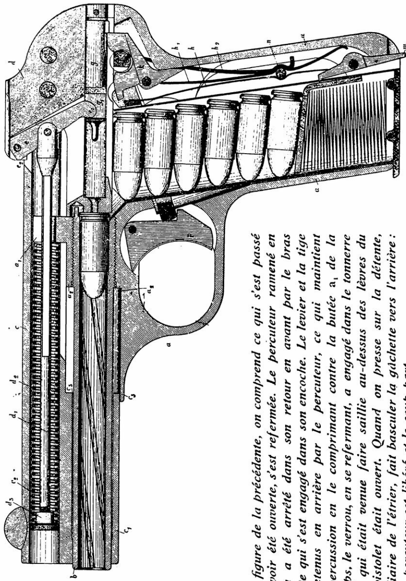
Fig. 3 — Coupe du pistolet automatique Browning calibre 7,65, le percuteur à l'armé.
