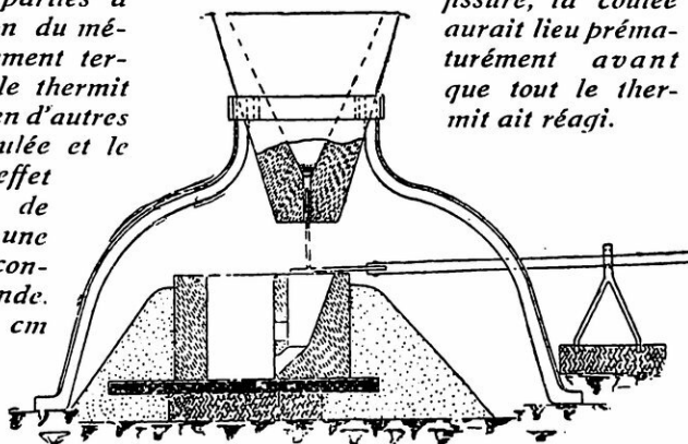
CREUSET AUTOMATIQUE. DÉBOUCHAGE DU TROU DE COULÉE
