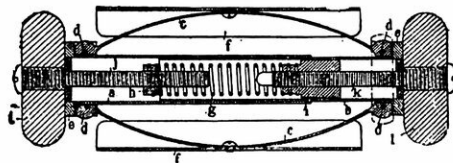
Haltère en coupe
